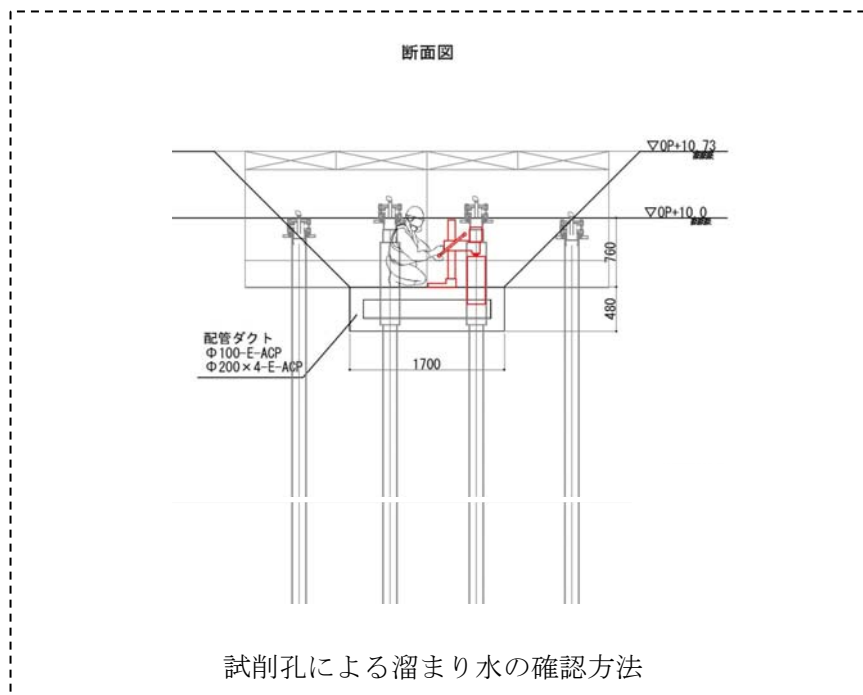
図14-26 【9-2】配管ダクト 施工方法（貫通施工）
