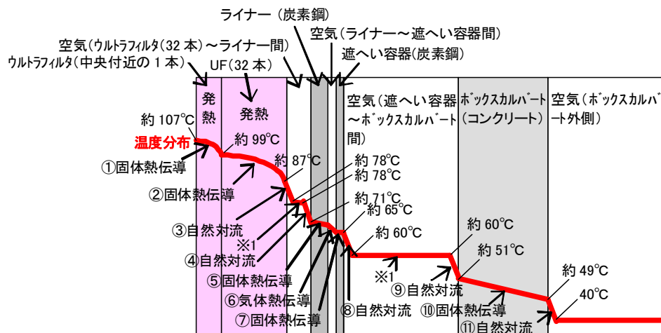
図ー２ 評価体系の概念図（１次元定常温度評価モデル）及び温度分布（ウルトラフィルタ） ※１：自然対流により混合され温度勾配はないものと仮定する。
