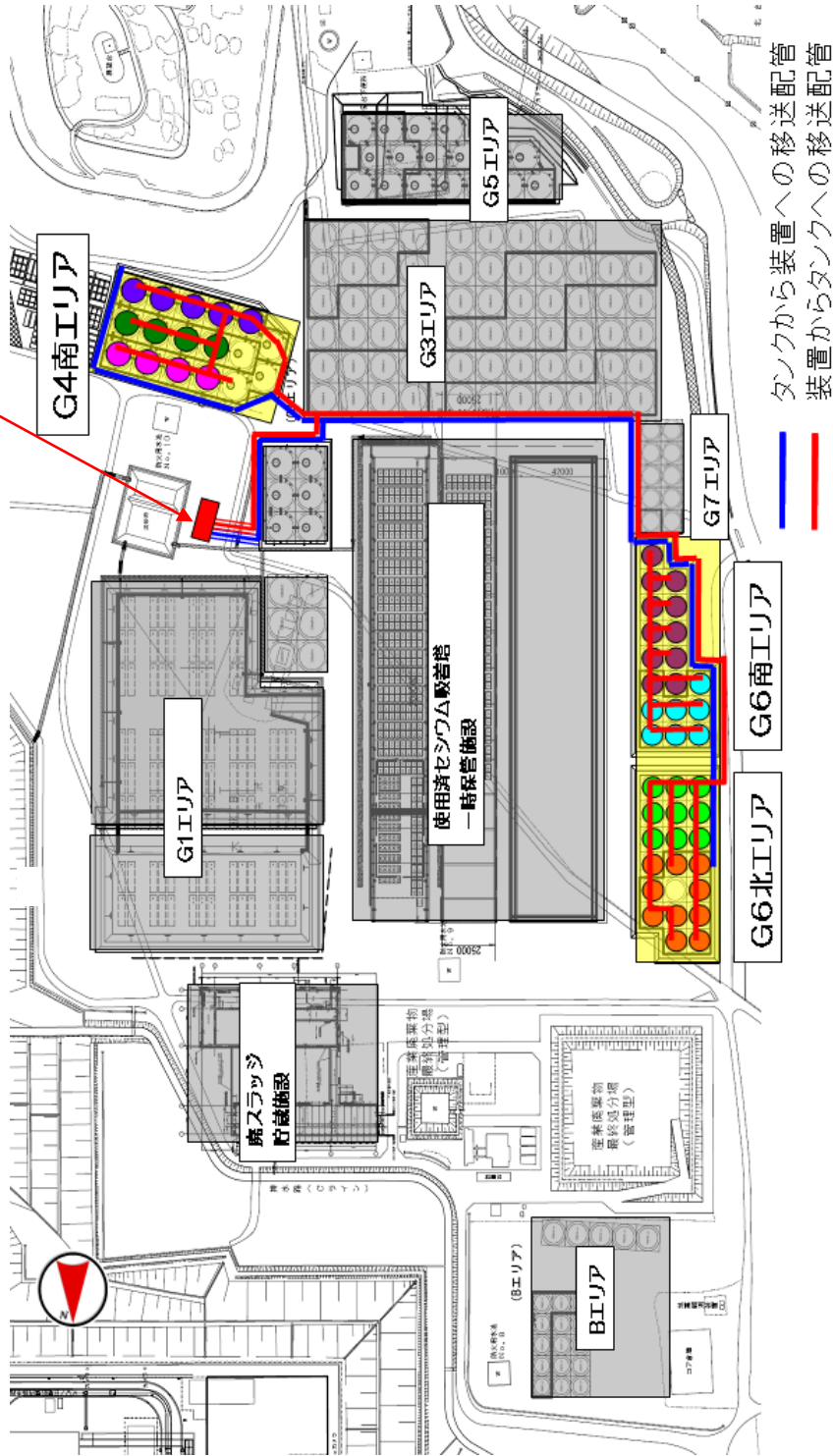
図-1 モバイル型ストロンチウム除去装置配置概要
