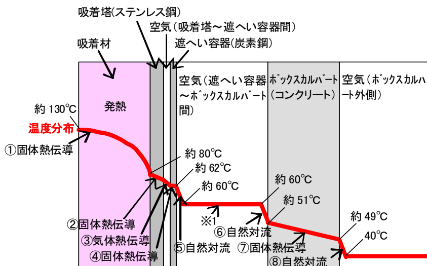
図-3 評価体系の概念図（1次元定常温度評価モデル）及び温度分布（吸着塔）
