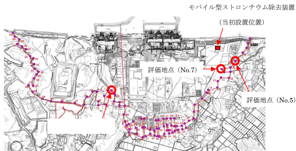
図1 モバイル型ストロンチウム除去装置（当初設置位置）と評価点の位置関係
