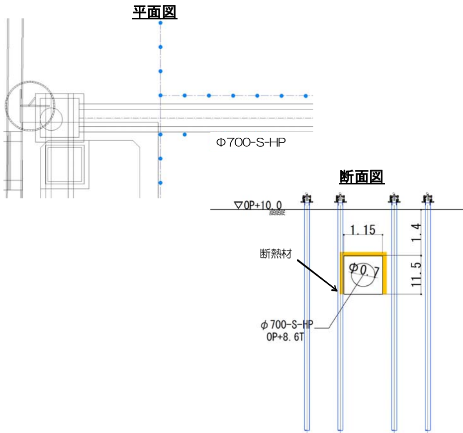
図 1 4 - 2 4 排水ヒューム管② 施工方法 (複列施工)
