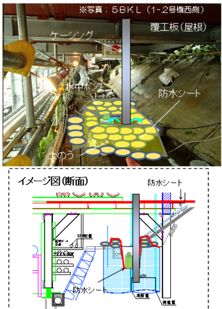
図 1 1 削孔水の漏えい対策イメージ
