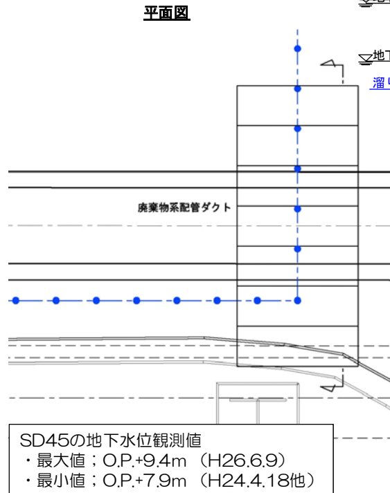
図14-21 廃棄物系共通配管ダクト① 施工方法 (貫通施工)
