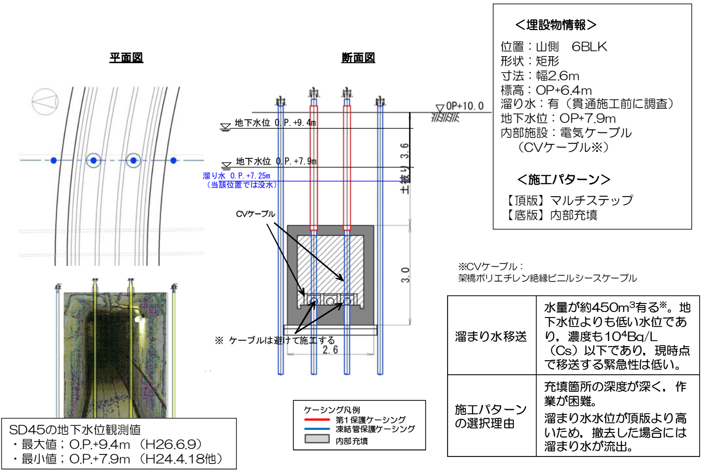
図14-16 4号機主変圧器ケーブルダクト 施工方法（貫通施工）
