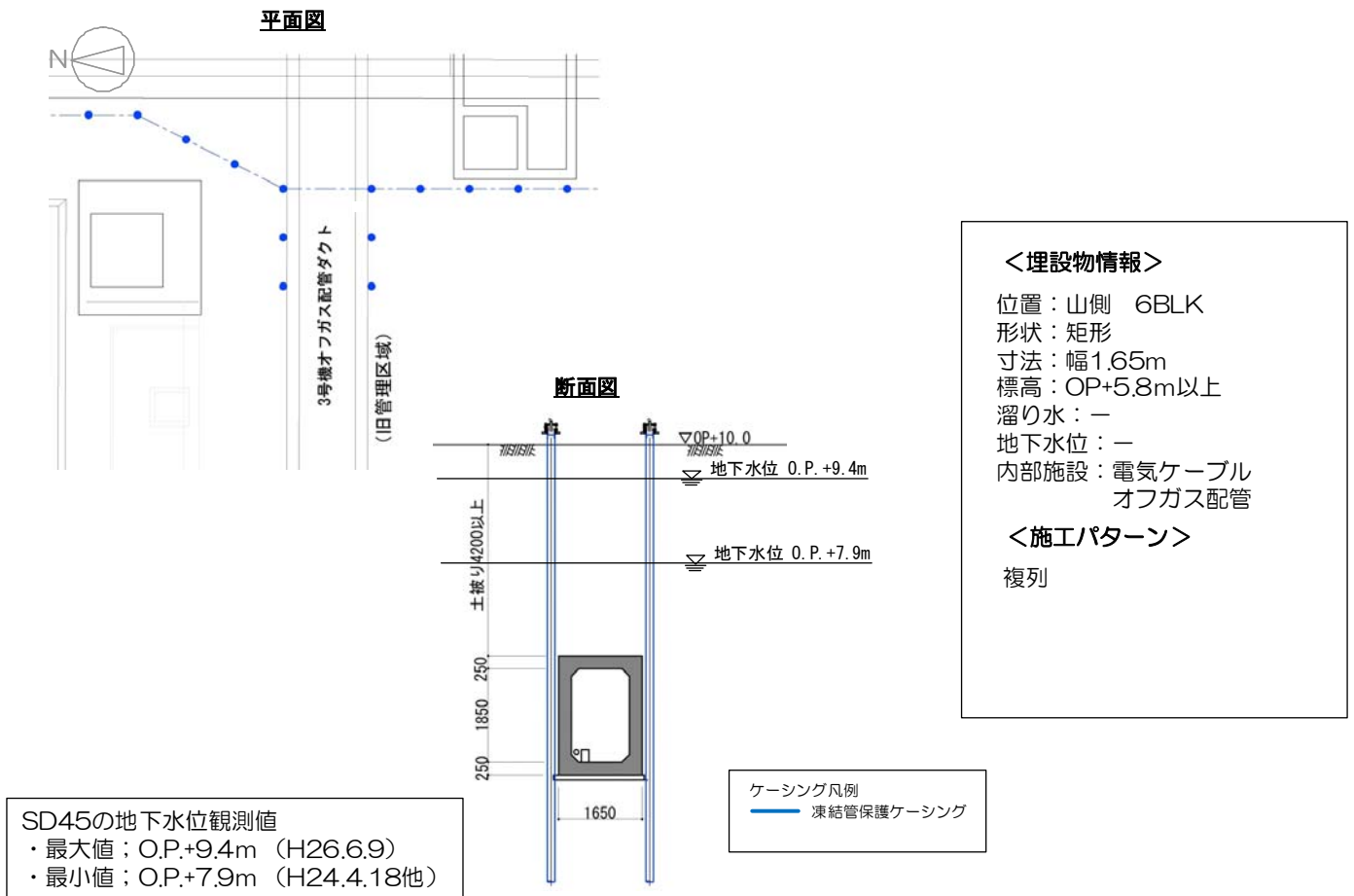
図 1 4 - 1 2 3号機オフガス配管ダクト（北側） 施工方法（複列施工）
