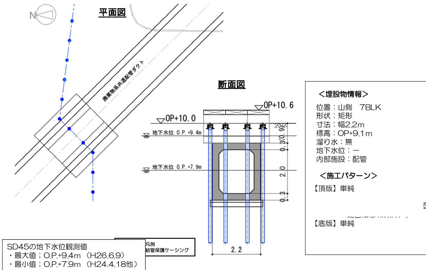
図14-22 廃棄物系共通配管ダクト② 施工方法（貫通施工）
