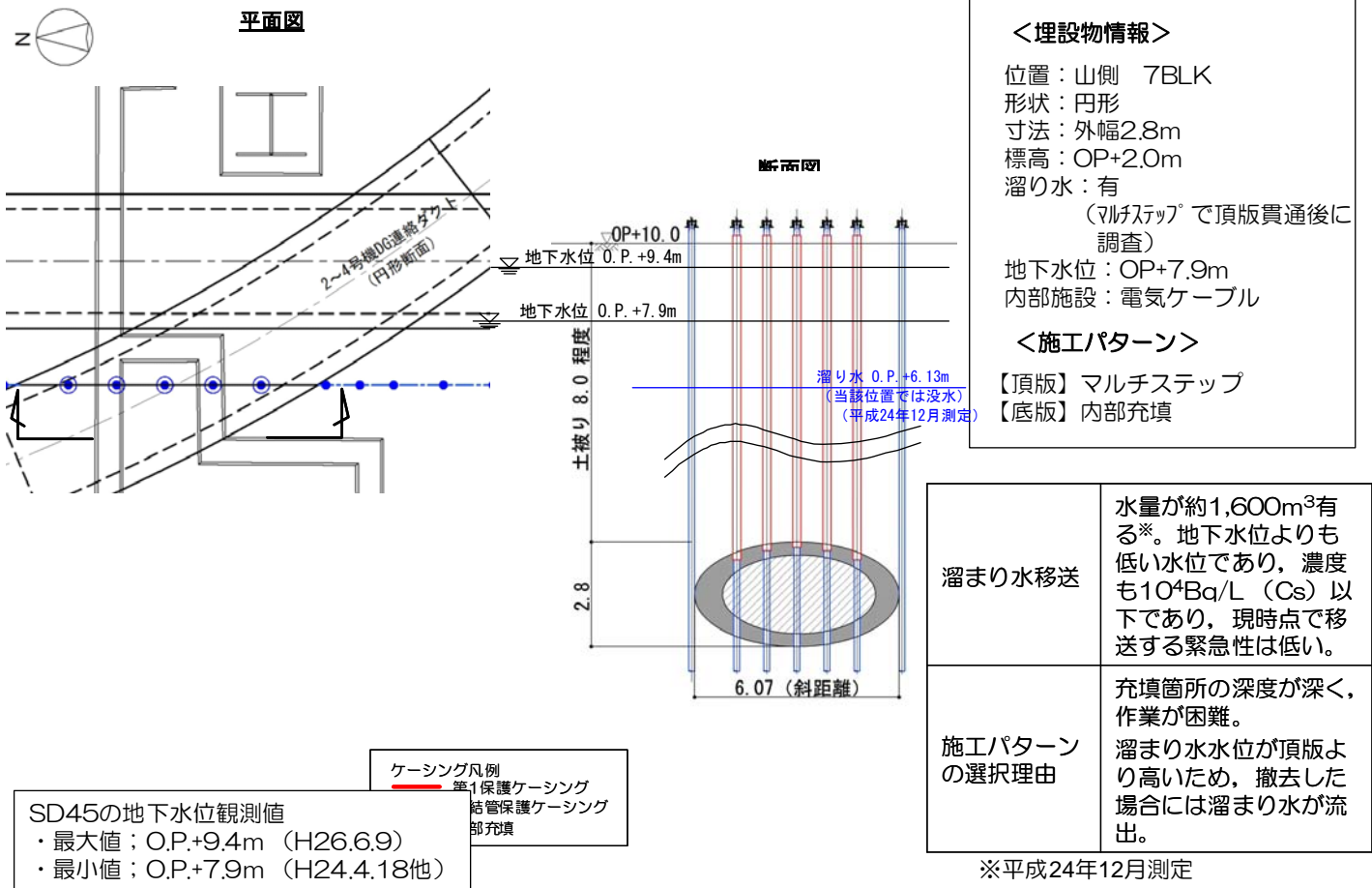
図14-19 2~4号機DG連絡ダクト③ 施工方法(貫通施工)
