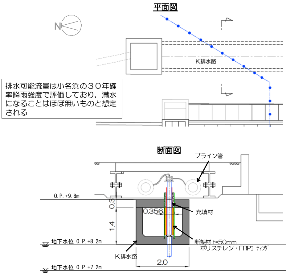
図 1 4 - 4 K排水路① 施工方法（貫通施工）
