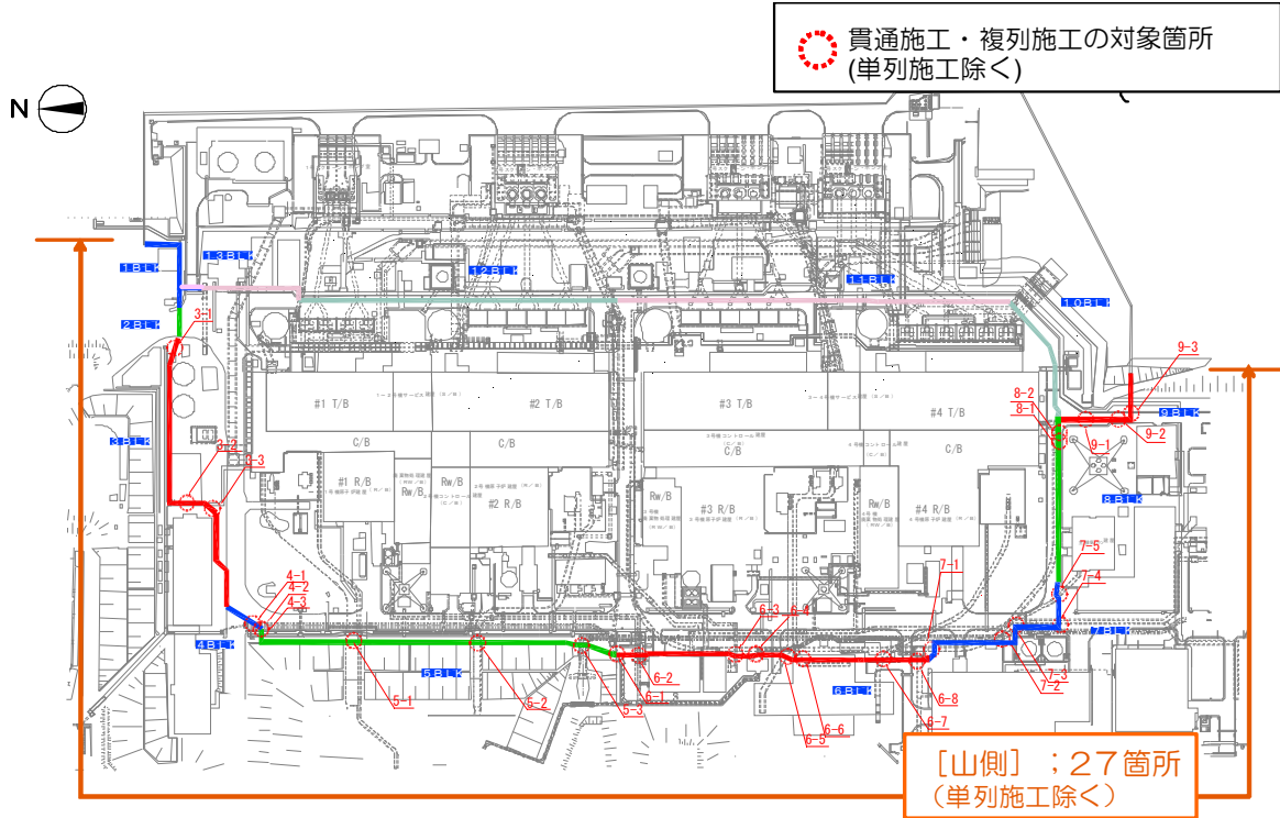
図13-1 貫通施工・複列施工の対象箇所(1)
