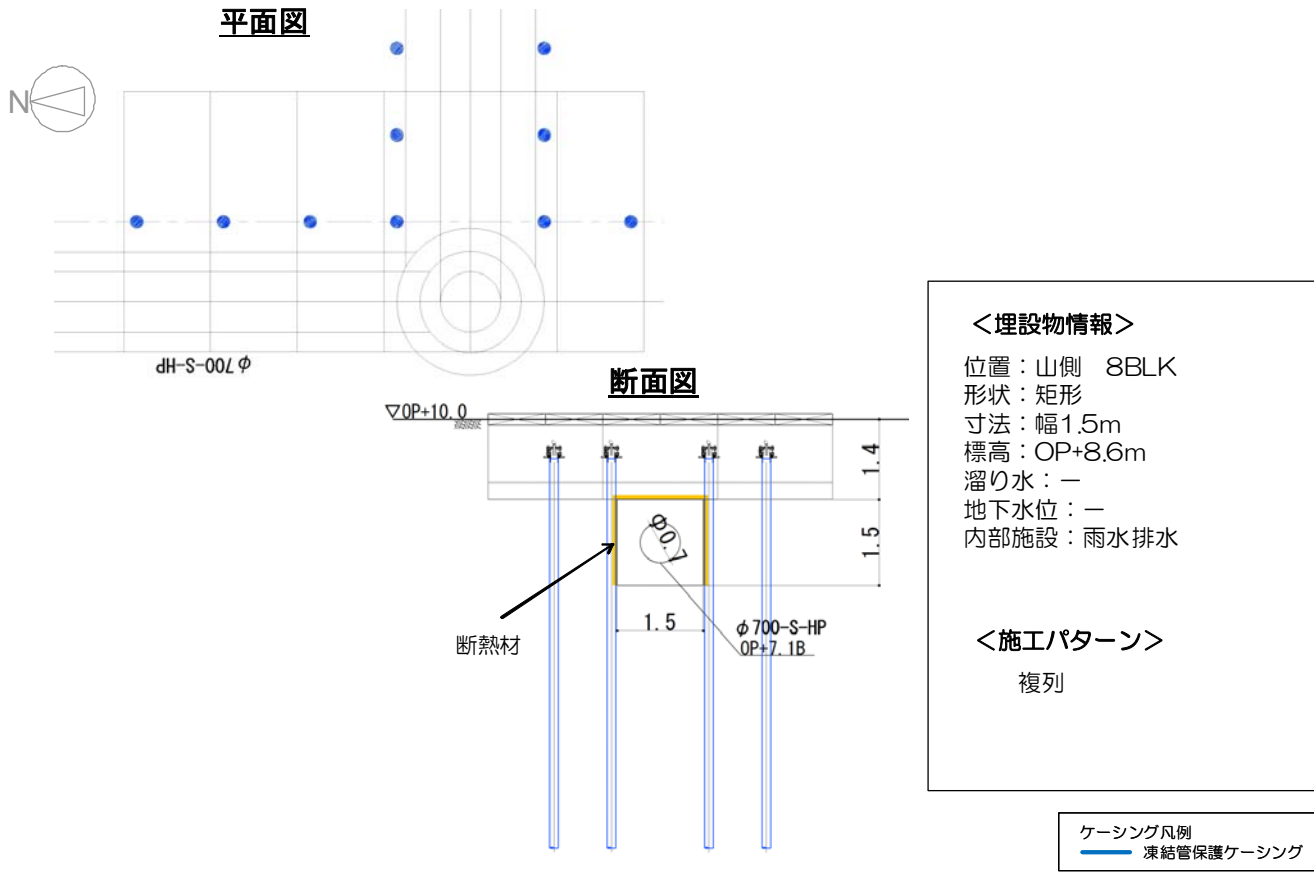
図 1 4 - 2 5 排水ヒューム管③ 施工方法（複列施工）
