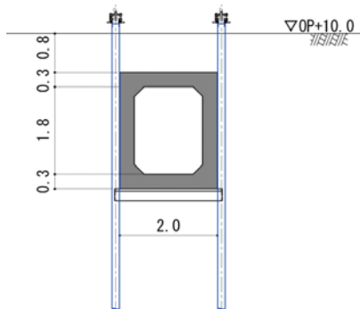
図 1 4 - 3 水処理建屋〜1号機 T/B 連絡ダクト② 施工方法 (複列施工)
