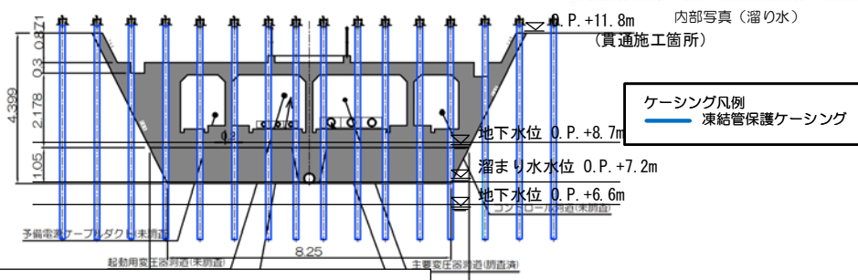
断面図
