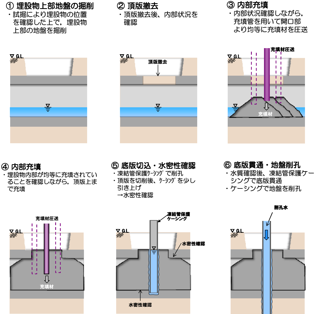
図9 頂版撤去・底版内部充填工法の施工手順
