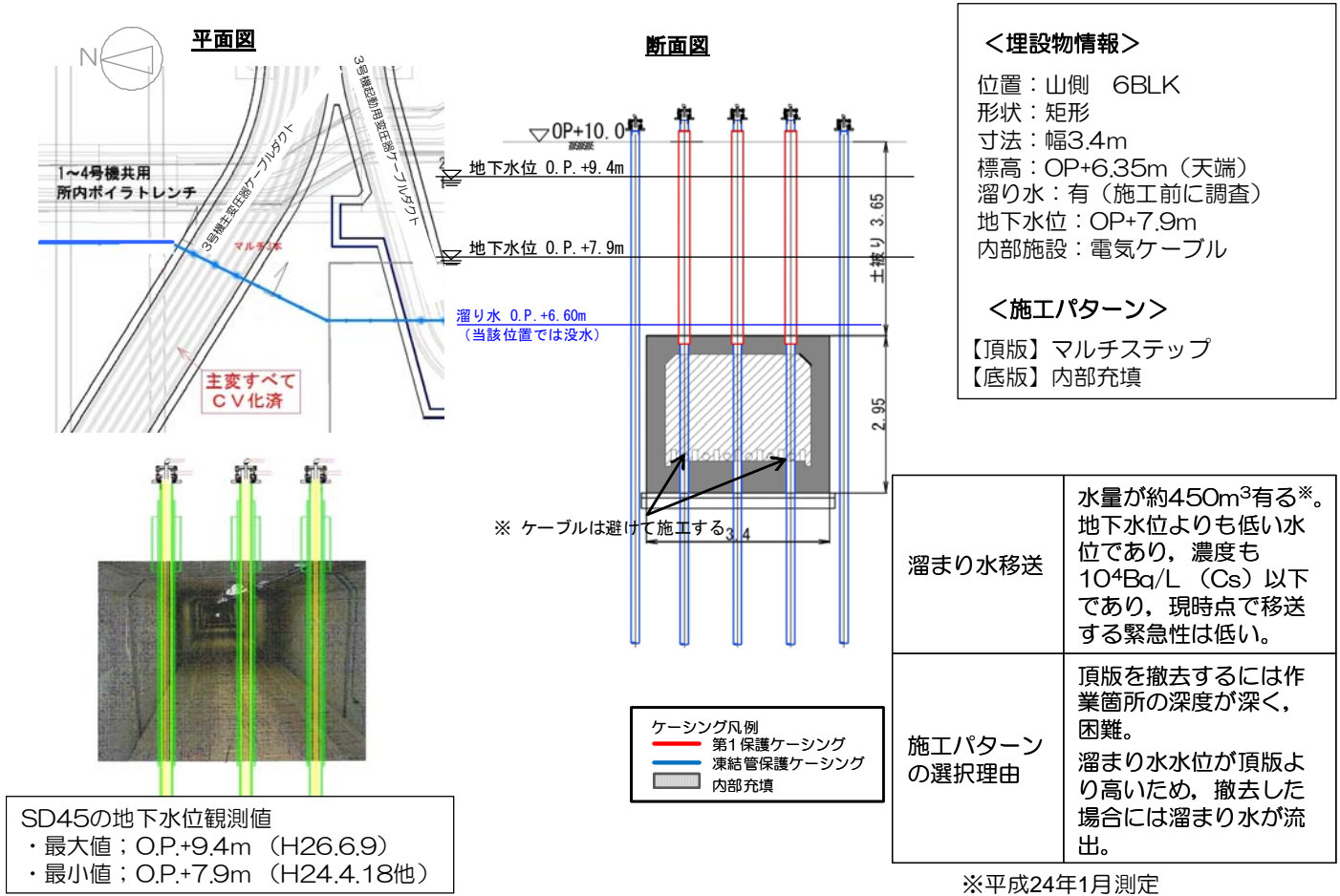
図14-14 3号機主変圧器ケーブルダクト 施工方法（貫通施工）
