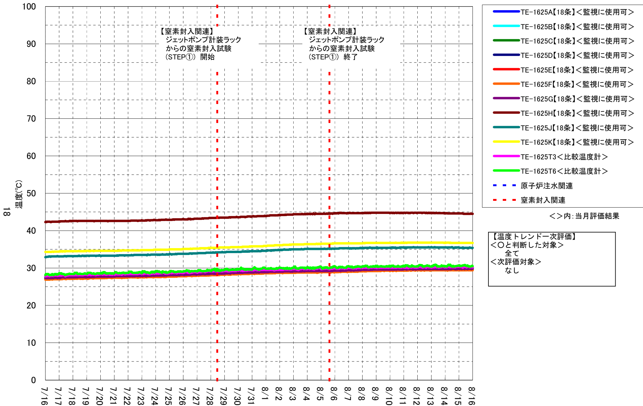
1号機 実施計画関連温度計(PCV)
