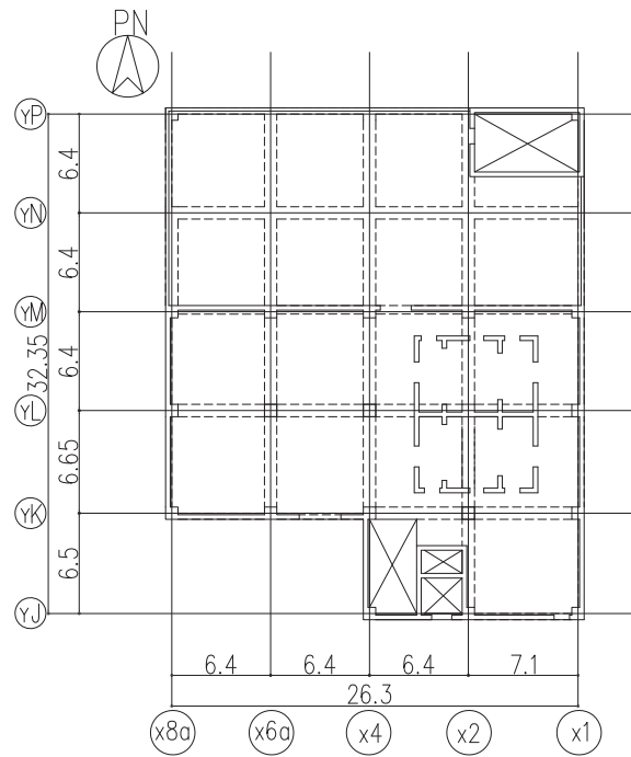
图一 1 5 塔屋階平面図 (G. L. +11.0) (单位 : m)
