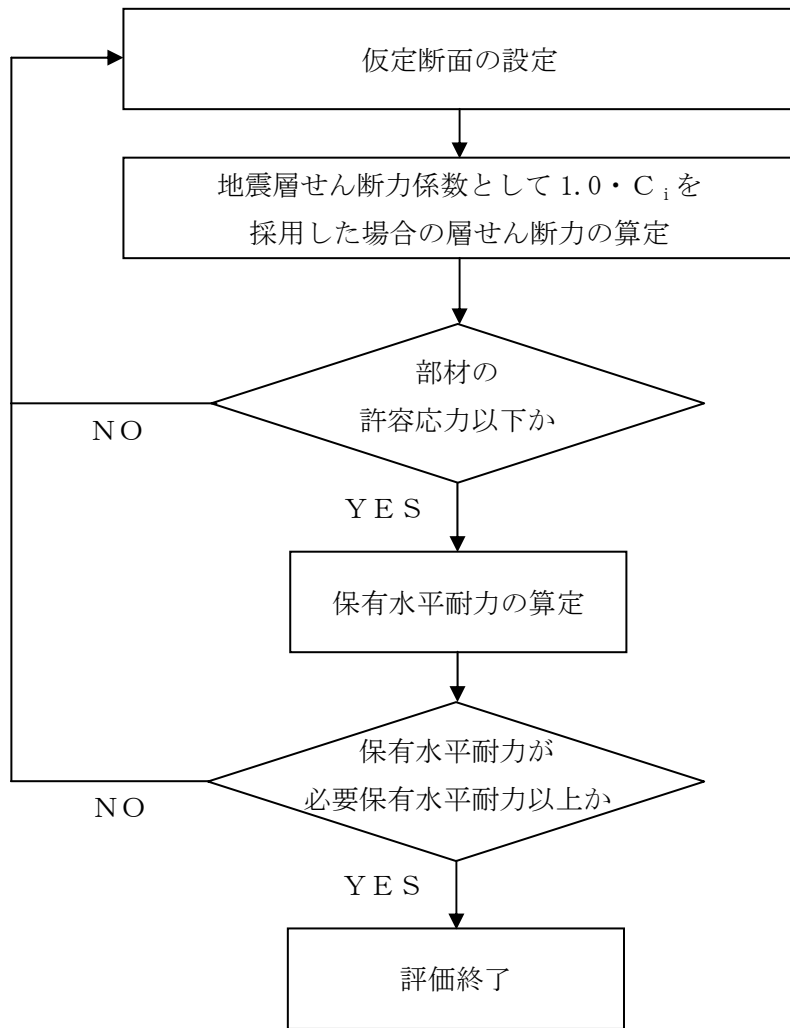
図-19 Cクラス施設としての建屋の耐震安全性評価手順
