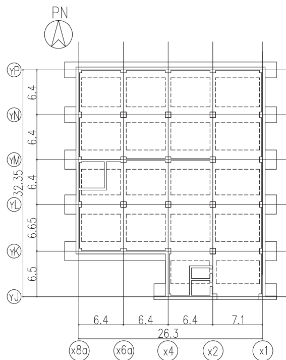
図-11 地下2階平面図 (G.L. -8.7) (単位 : m)
