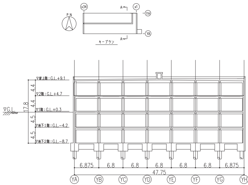
図-7 A-A断面図 (単位: m)
