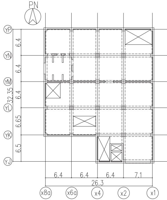
图一 1 4 地上2階平面図 (G. L. +4.7) (单位 : m)
