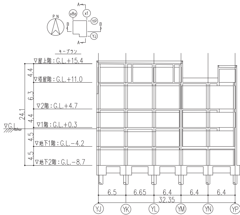
図-17 A-A断面図 (単位: m)
