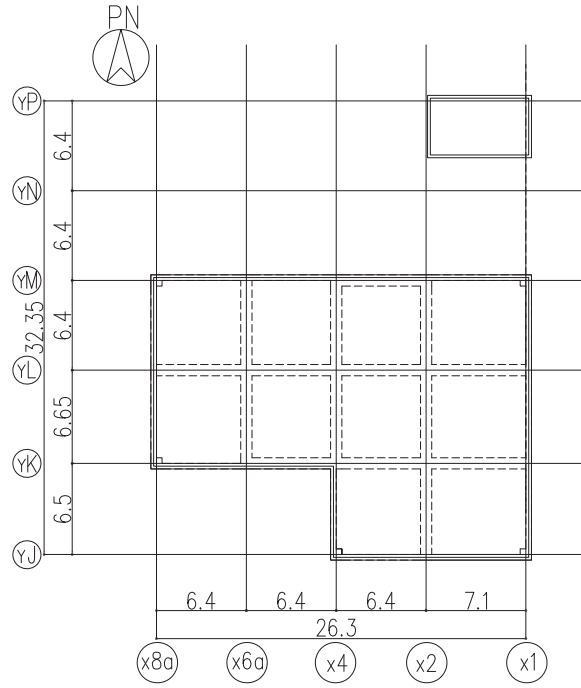
图-16 屋上階平面図 (G. L. +15.4) (单位 : m)
