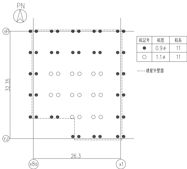
図-10 杭配置図 (G.L. -11.0) (単位 : m)
