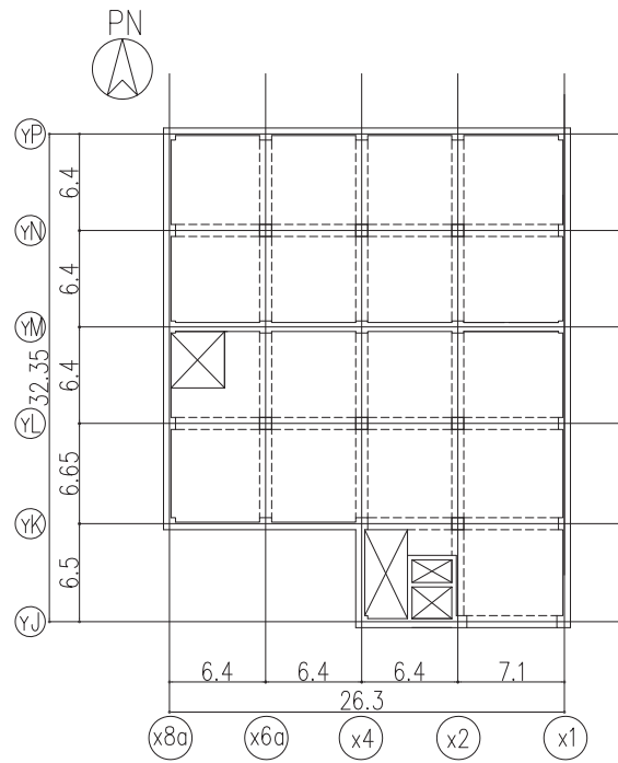
图-1-2 地下1階平面図 (G.L. -4.2) (单位 : m)
