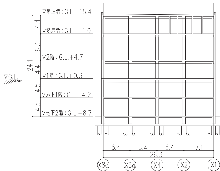
図-18 B-B断面図 (単位: m)
