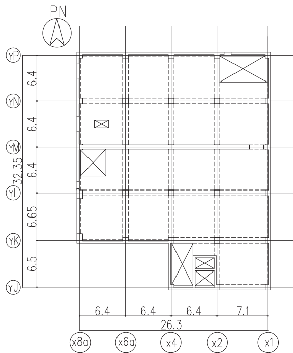
图-1-3 地上1階平面図 (G.L. +0.3) (单位 : m)
