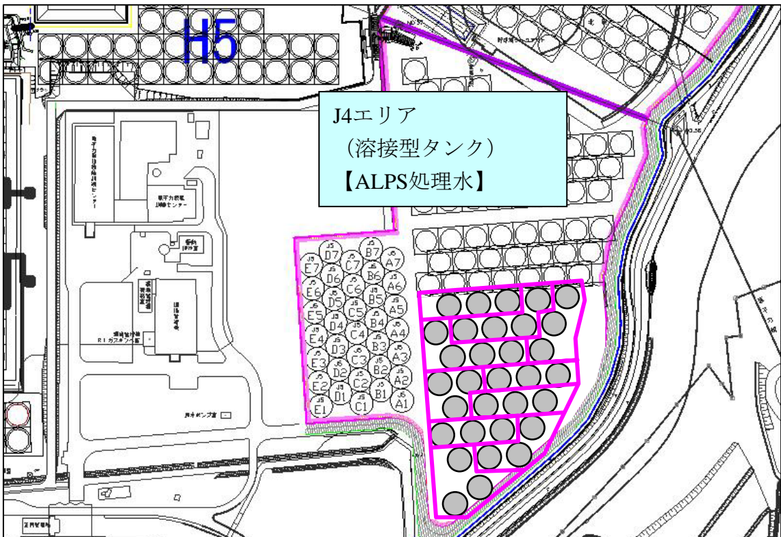
タンクエリア詳細図 (J4)
