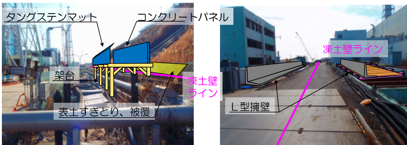
図 1 2 被ばく線量低減対策実施例 1
