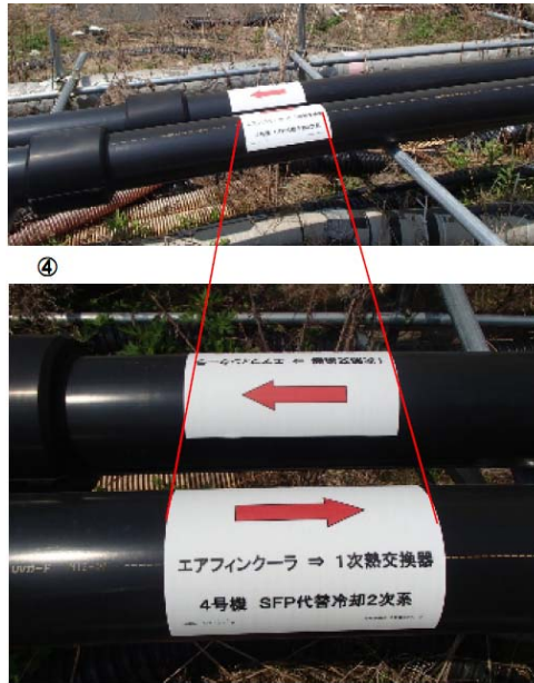
図 1 0 運用中の設備の損傷防止策（注意喚起の表示（例））
