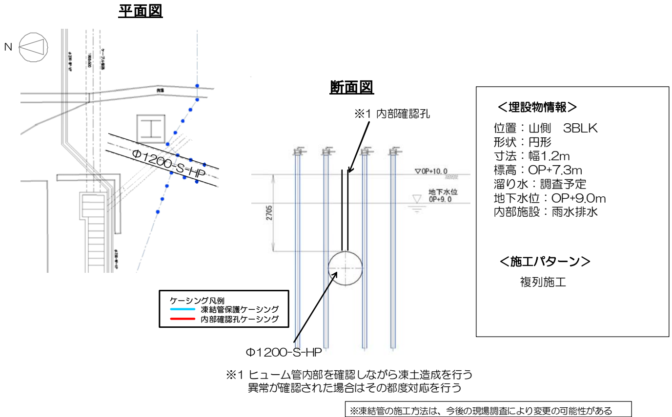
図 1 2 - 1 排水ヒューム管① 施工方法（複列施工）
