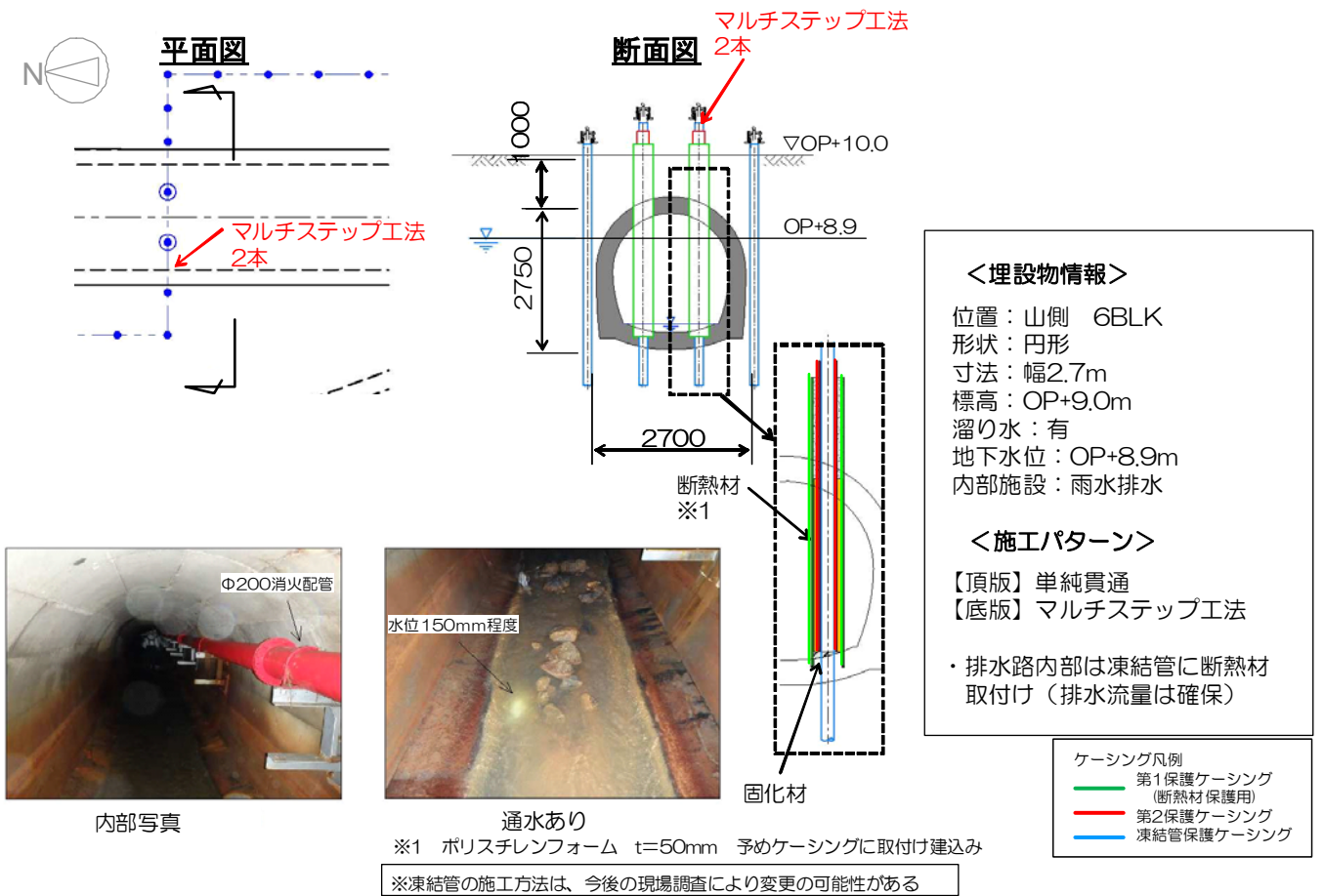
図 1 2 - 1 8 K排水路② 施工方法（貫通施工）
