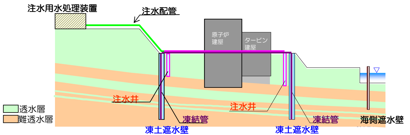
図7 注水機器全体概要図 平面図・断面図
