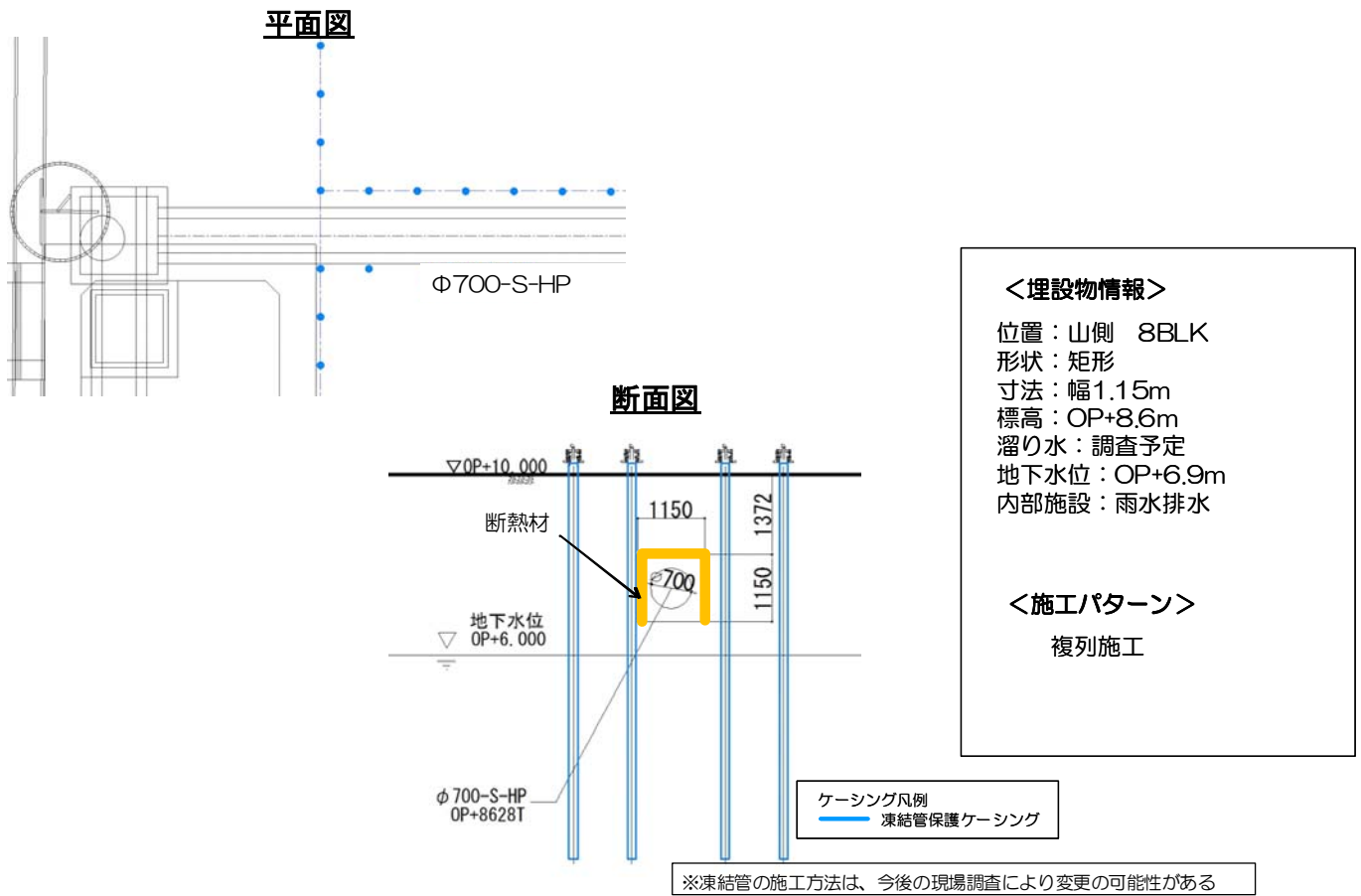
図 1 2 - 2 4 排水ヒューム管② 施工方法（複列施工）
