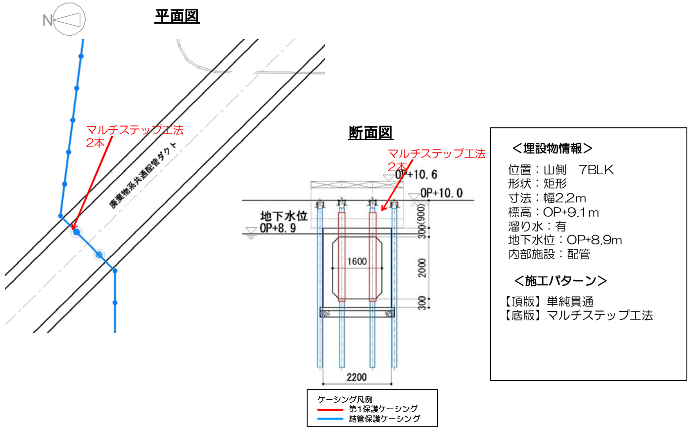
図12-22 廃棄物系共通配管ダクト② 施工方法（貫通施工）
