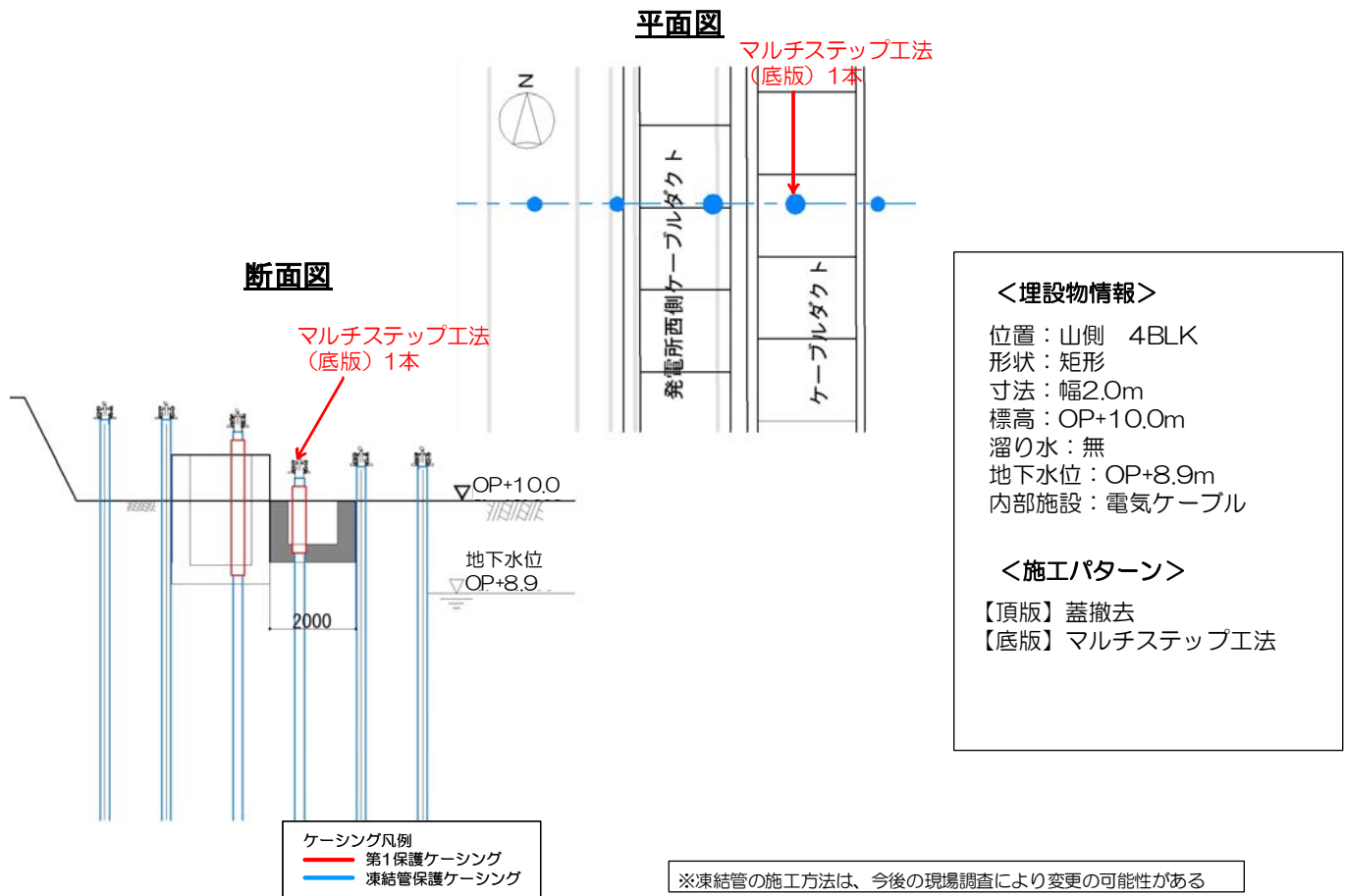
図 1 2 - 5 ケーブルダクト 施工方法 (貫通施工)
