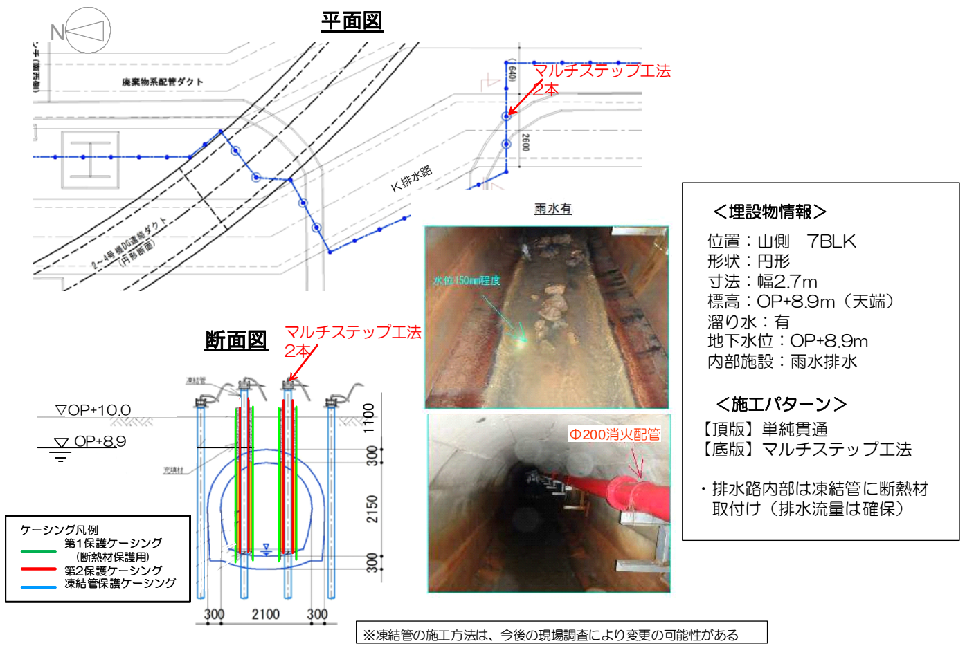
図 1 2 - 2 0 K排水路③ 施工方法 (貫通施工)
