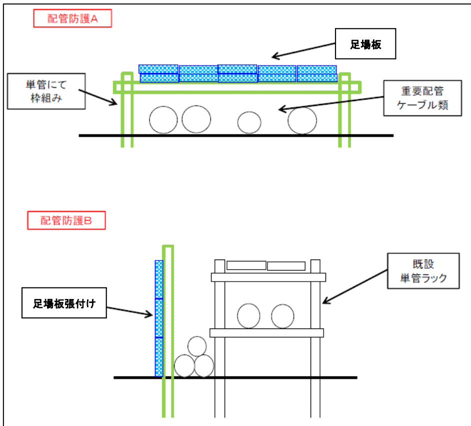
図 1 1 運用中の設備の損傷防止策（配管防護（例））
