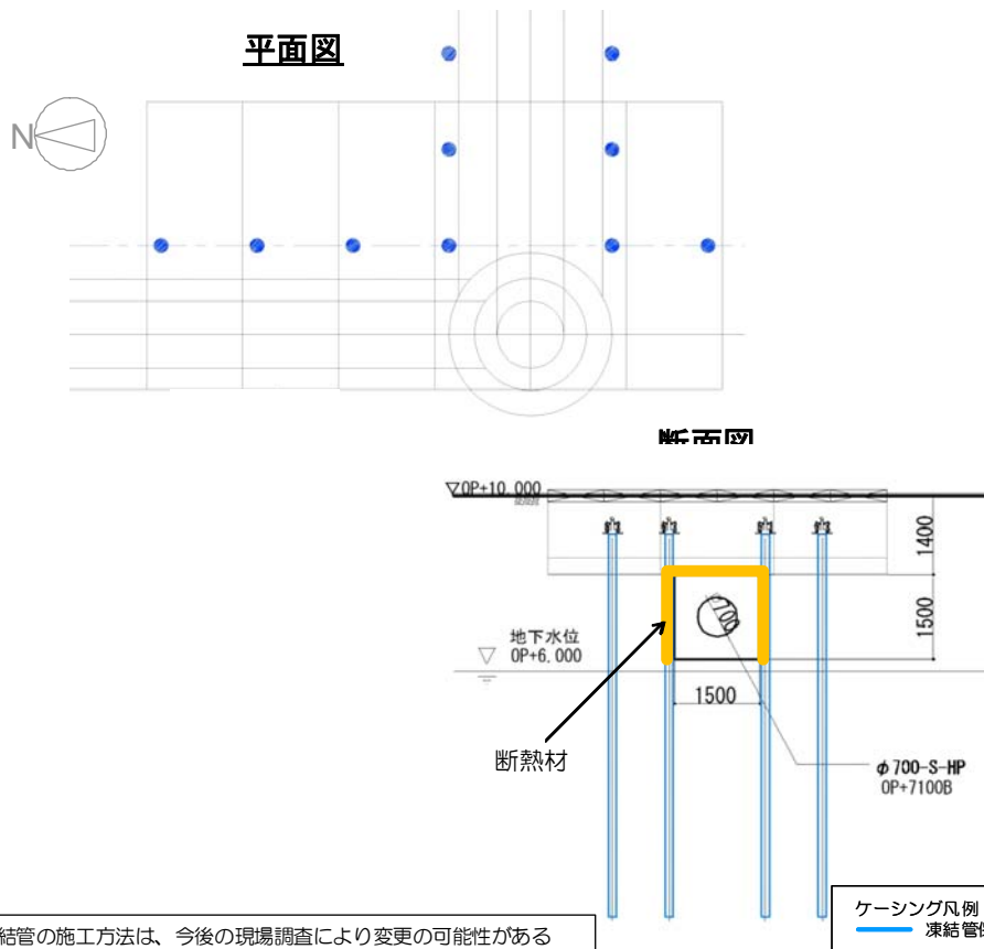
図 1 2 - 2 5 排水ヒューム管③ 施工方法（複列施工）
