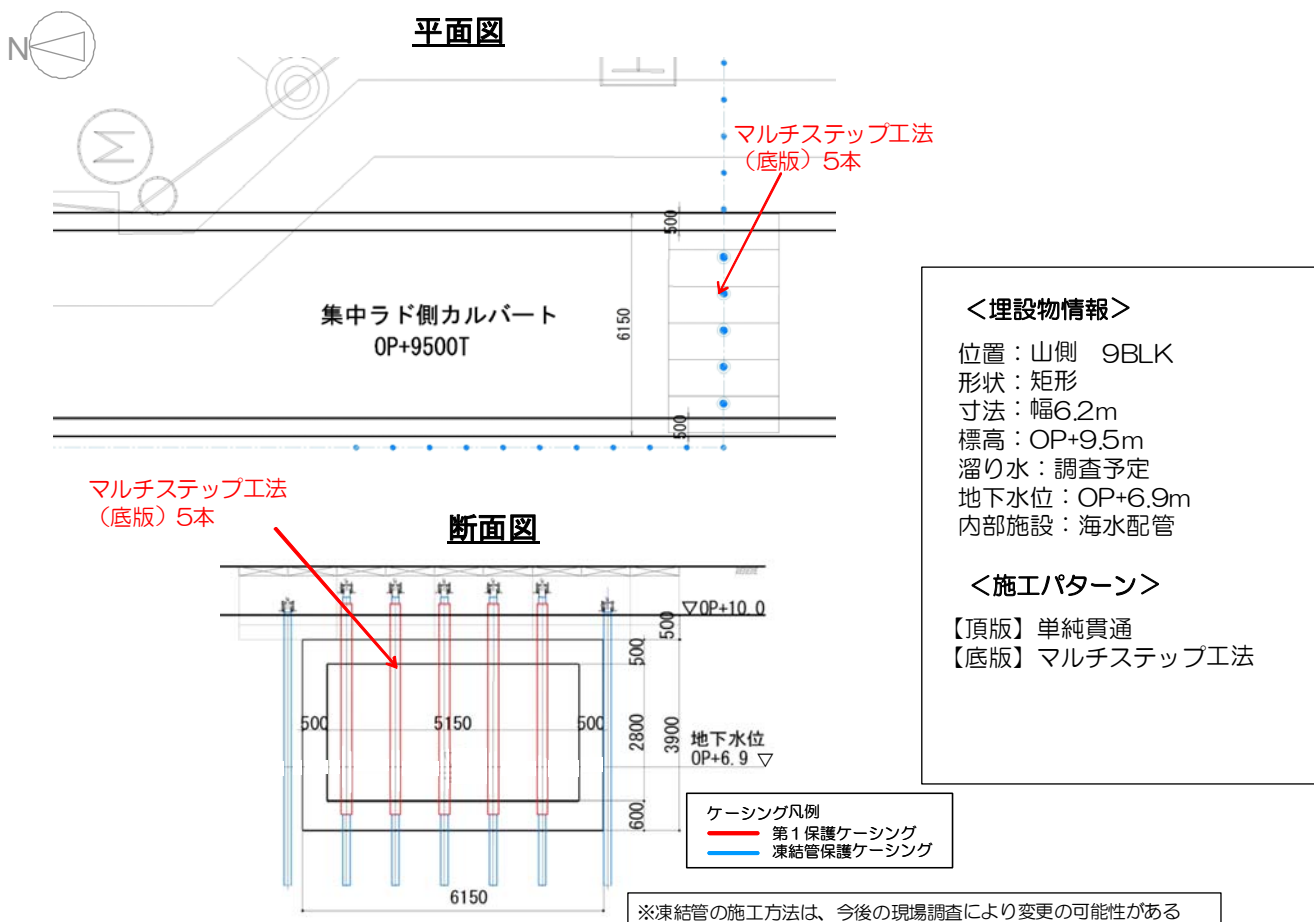
図 1 2 - 2 7 集中ラド側カルバート 施工方法 (貫通施工)
