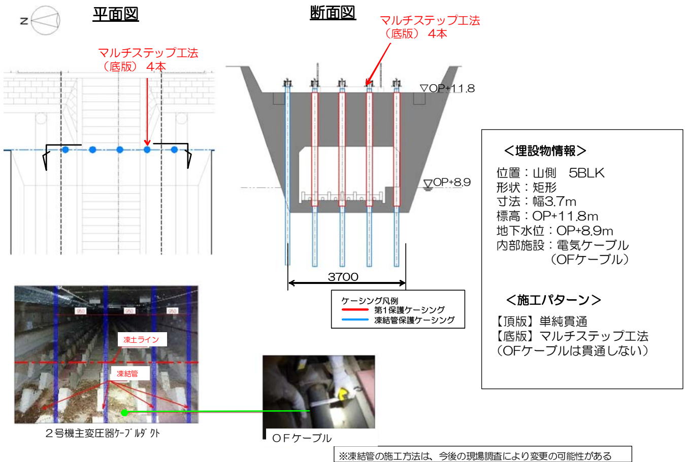
図 1 2 - 8 2号機主変圧器ケーブルダクト 施工方法 (貫通施工)
