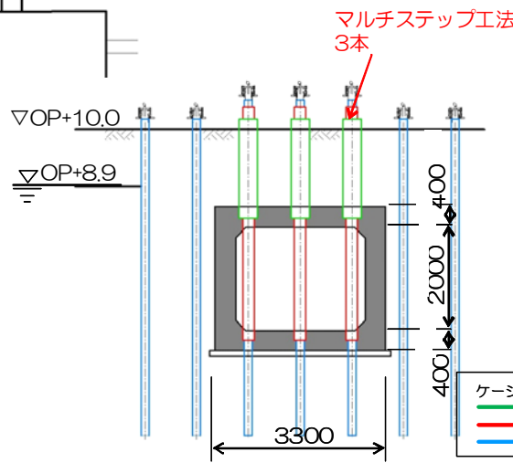
図 1 2 - 1 6 2~4 号機 DG 連絡ダクト① 施工方法 (貫通施工)
