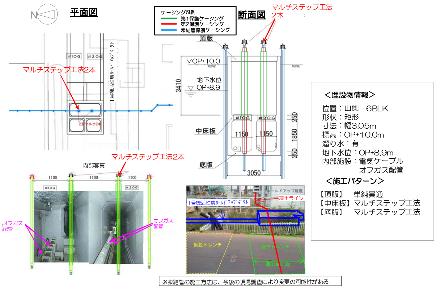
図 1 2 - 1 1 1 号機活性炭ホールドアップダクト 施工方法 (貫通施工)
