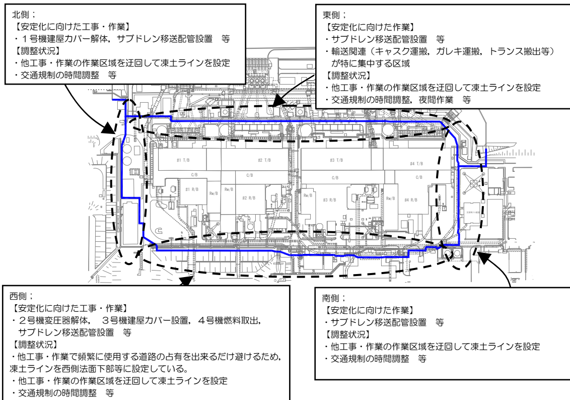
図 1 8 凍土遮水壁と他の安定化に向けた工事・作業との調整状況
