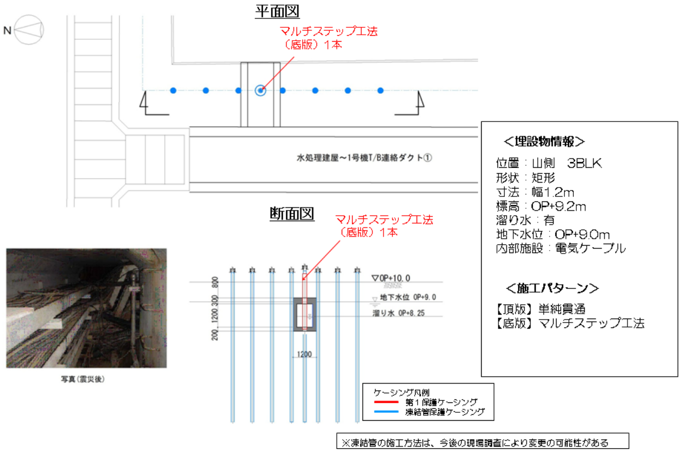
図 1 2 - 2 水処理建屋～1号機 T/B 連絡ダクト① 施工方法 (貫通施工)
