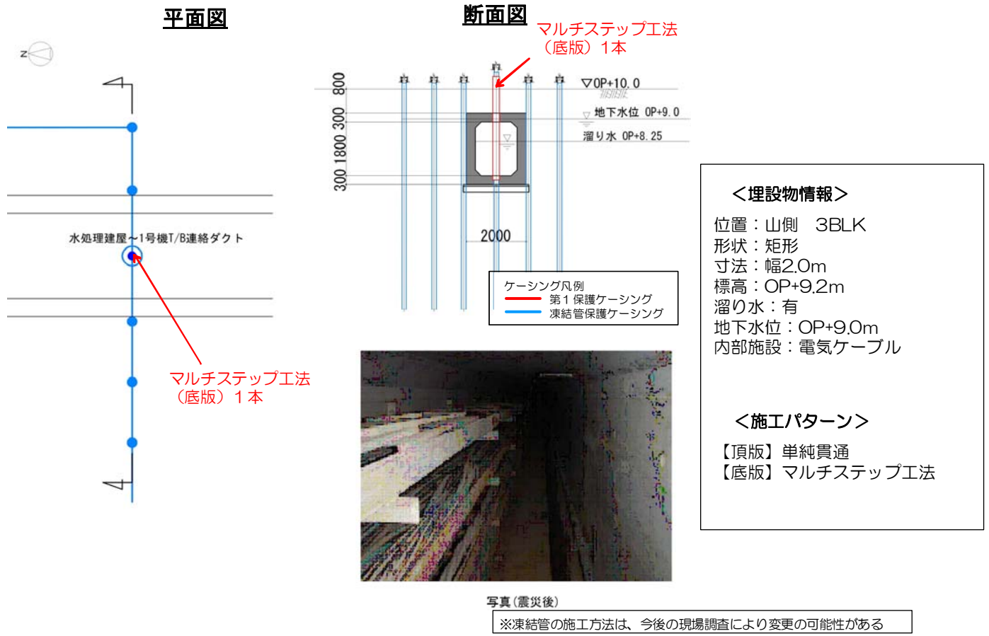
図 1 2 - 3 水処理建屋～1号機 T/B 連絡ダクト② 施工方法（貫通施工）
