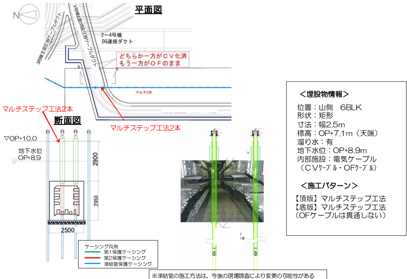
図 1 2 - 1 4 3号機起動用変圧器ケーブルダクト 施工方法（貫通施工）
