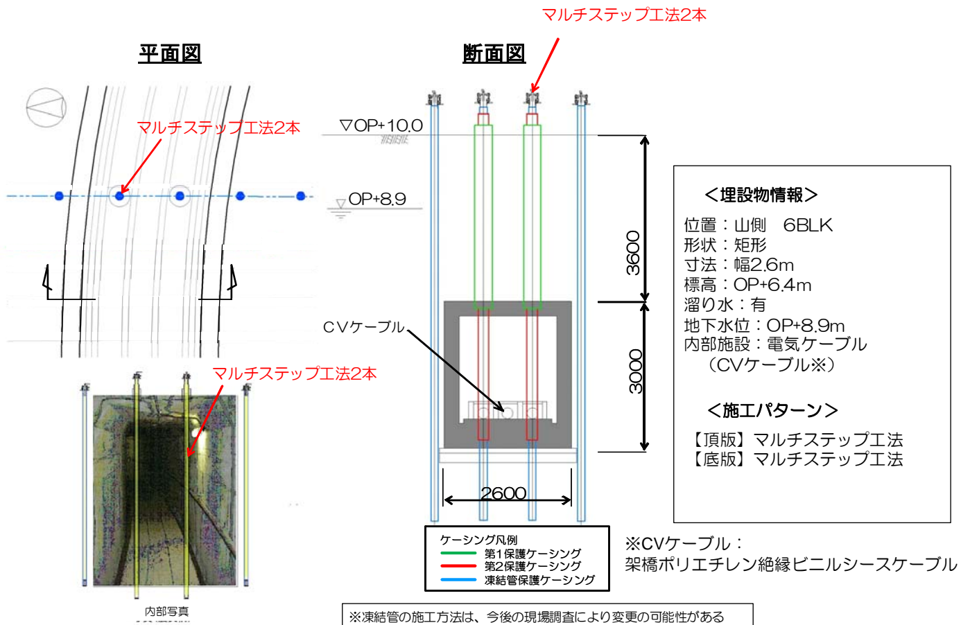
図12-15 4号機主変圧器ケーブルダクト 施工方法（貫通施工）
