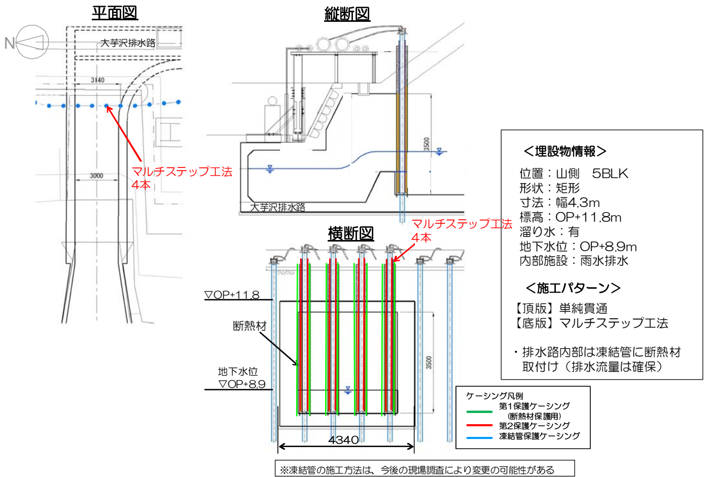
図 1 2 - 9 大芋沢排水路 施工方法（貫通施工）
