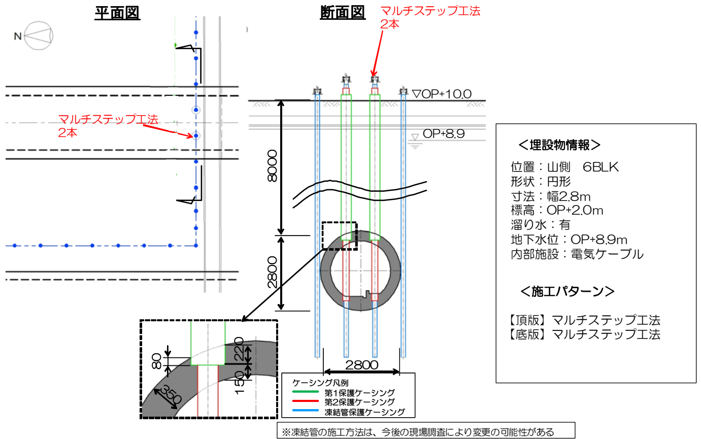
図 1 2 - 1 7 2~4 号機 DG 連絡ダクト② 施工方法 (貫通施工)
