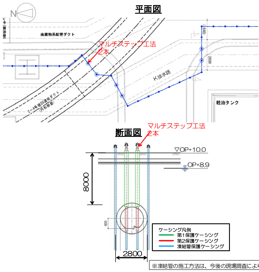
図 1 2 - 1 9 2~4号機 DG 連絡ダクト③ 施工方法 (貫通施工)
