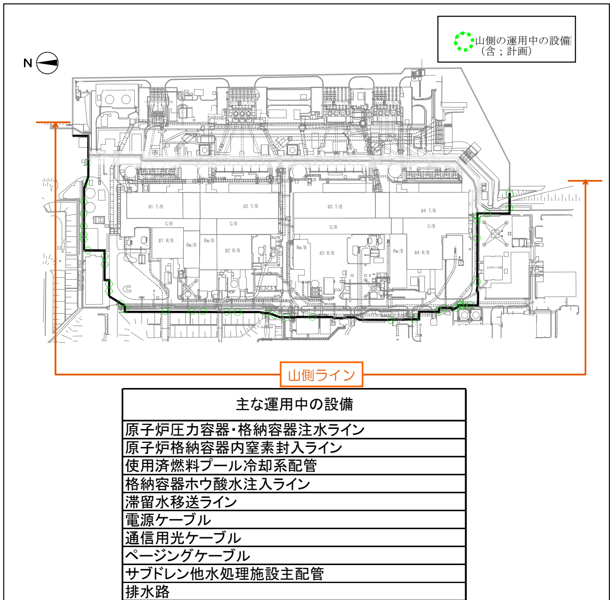
図9 山側ライン上の主な運用中の設備と凍土遮水壁の横断箇所
