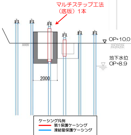
図 1 2 - 6 発電所西側ケーブルダクト 施工方法 (貫通施工)
