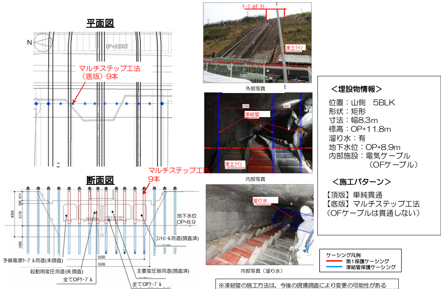
図 1 2 - 7 1号機電気ケーブルダクト 施工方法 (貫通施工)
