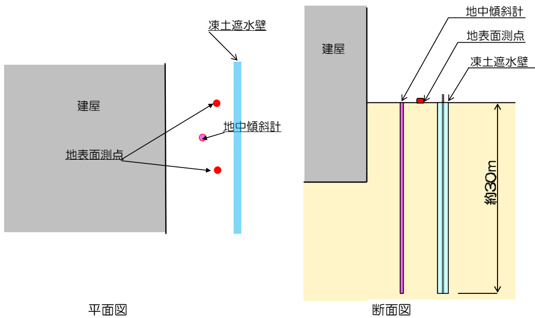
図17 凍結膨張に対するモニタリング
