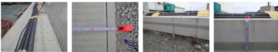
図 1 2 - 2 3 滞留水移送管 施工方法（複列施工）
