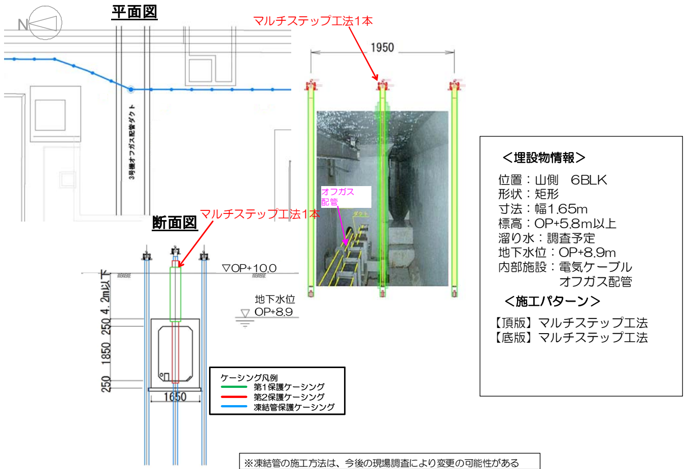
図 1 2 - 1 2 3 号機オフガス配管ダクト（北側） 施工方法（貫通施工）
