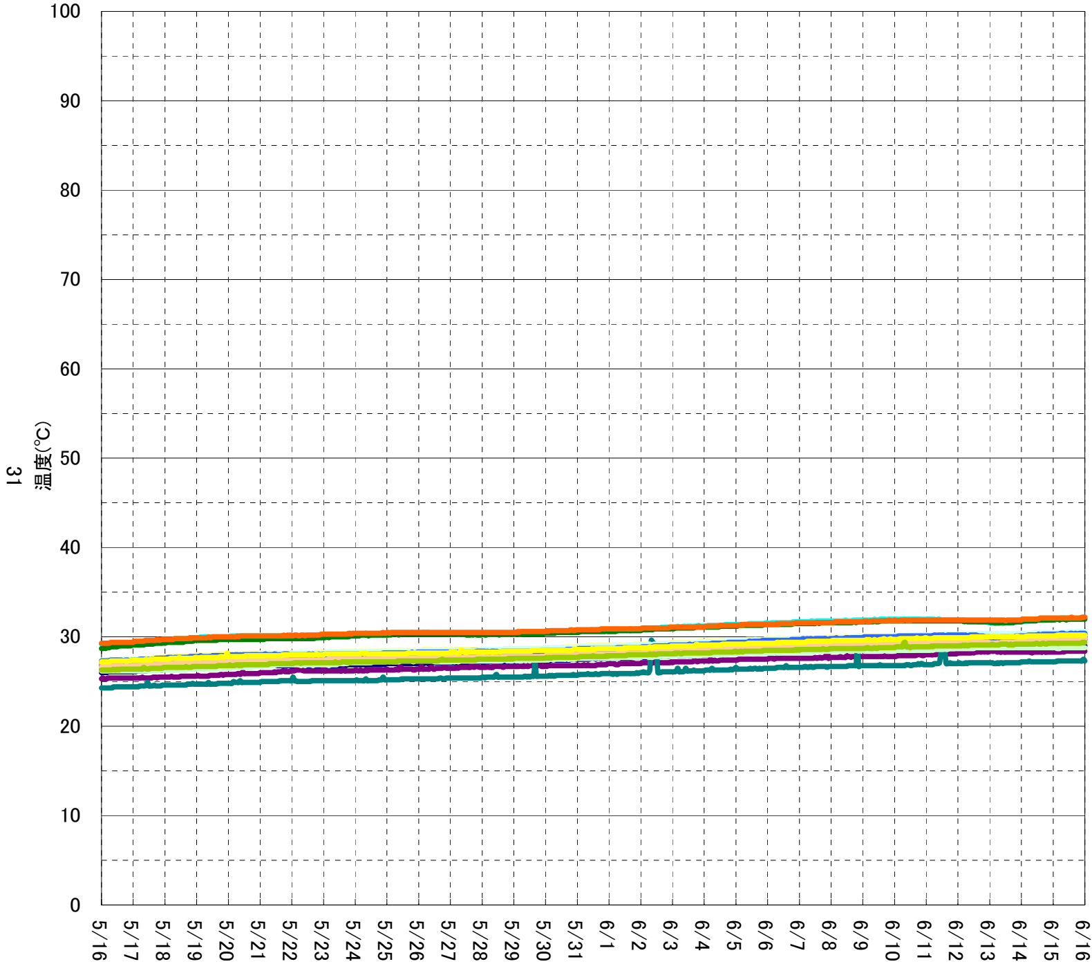
3号機 RPV周辺温度計(上部)
