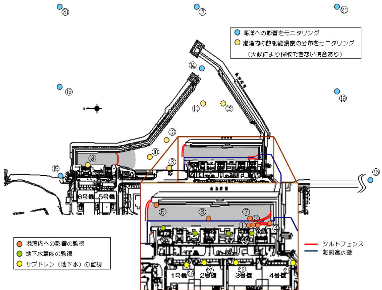
図1 地下水及び港湾内外海水のモニタリング計画 (サンプリング箇所)
