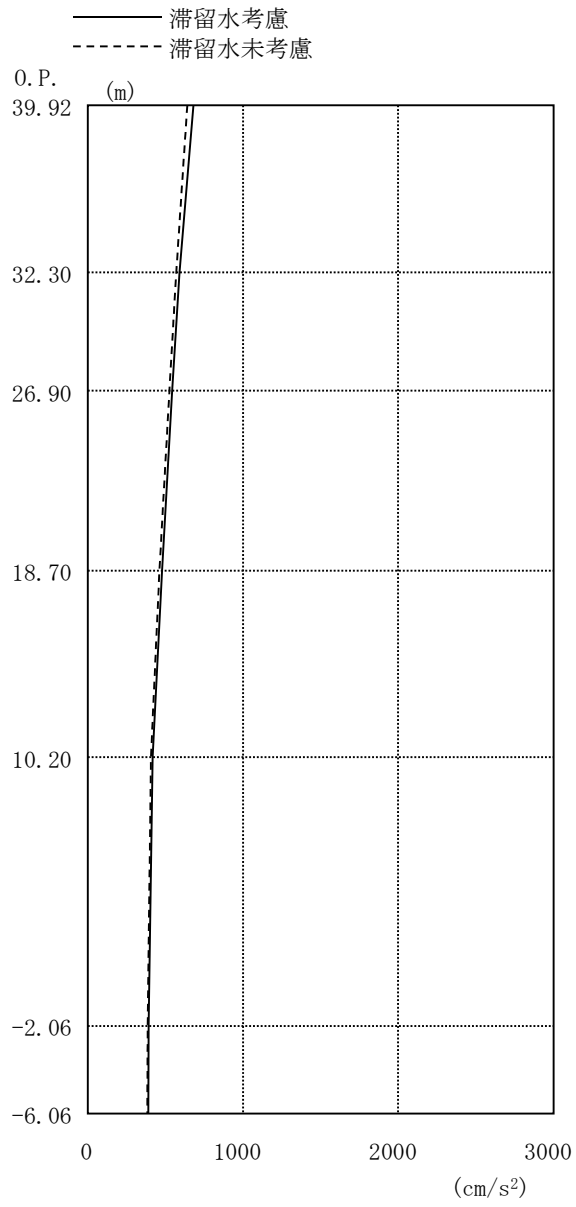
图 2.3.5-6 最大応答加速度 (EW 方向・Ss-3H)
