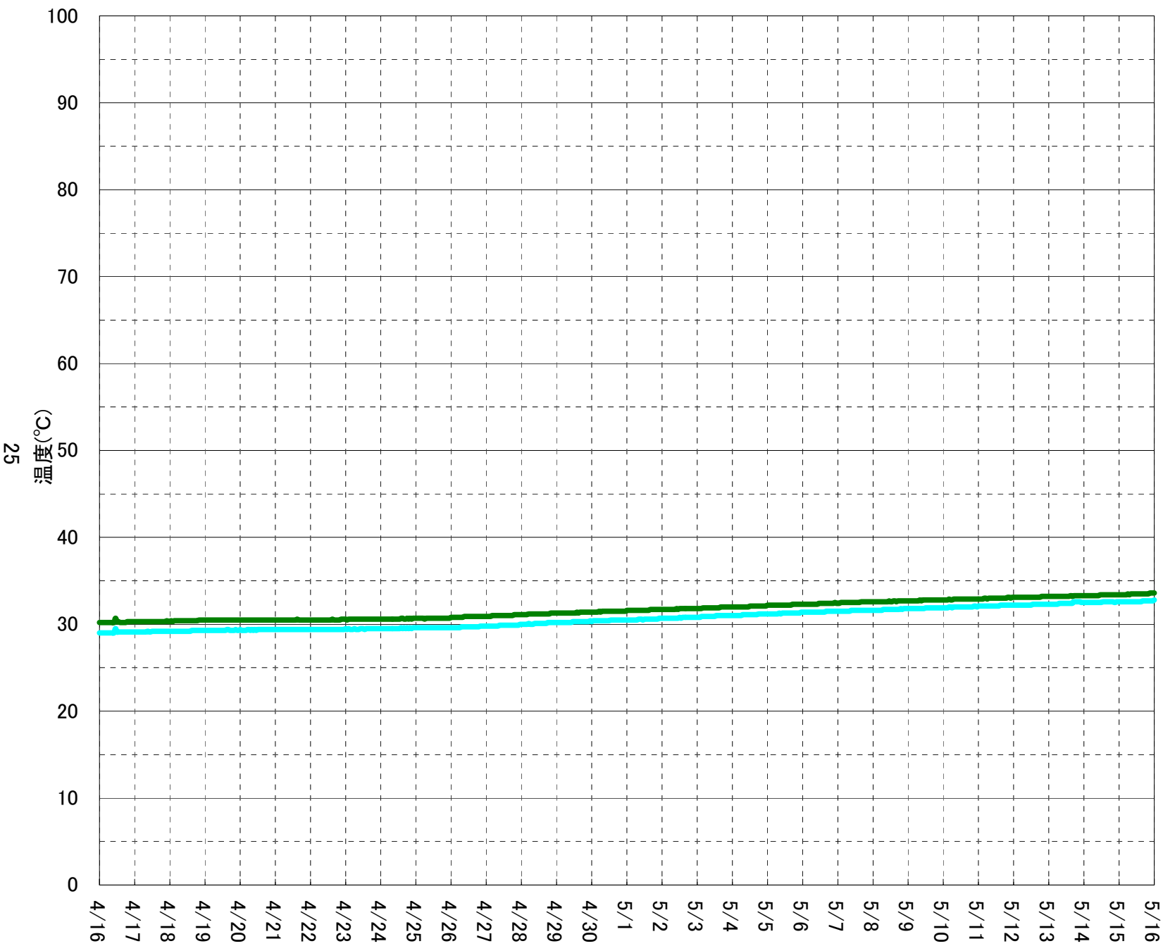
2号機 RPV周辺温度計(上部)②
