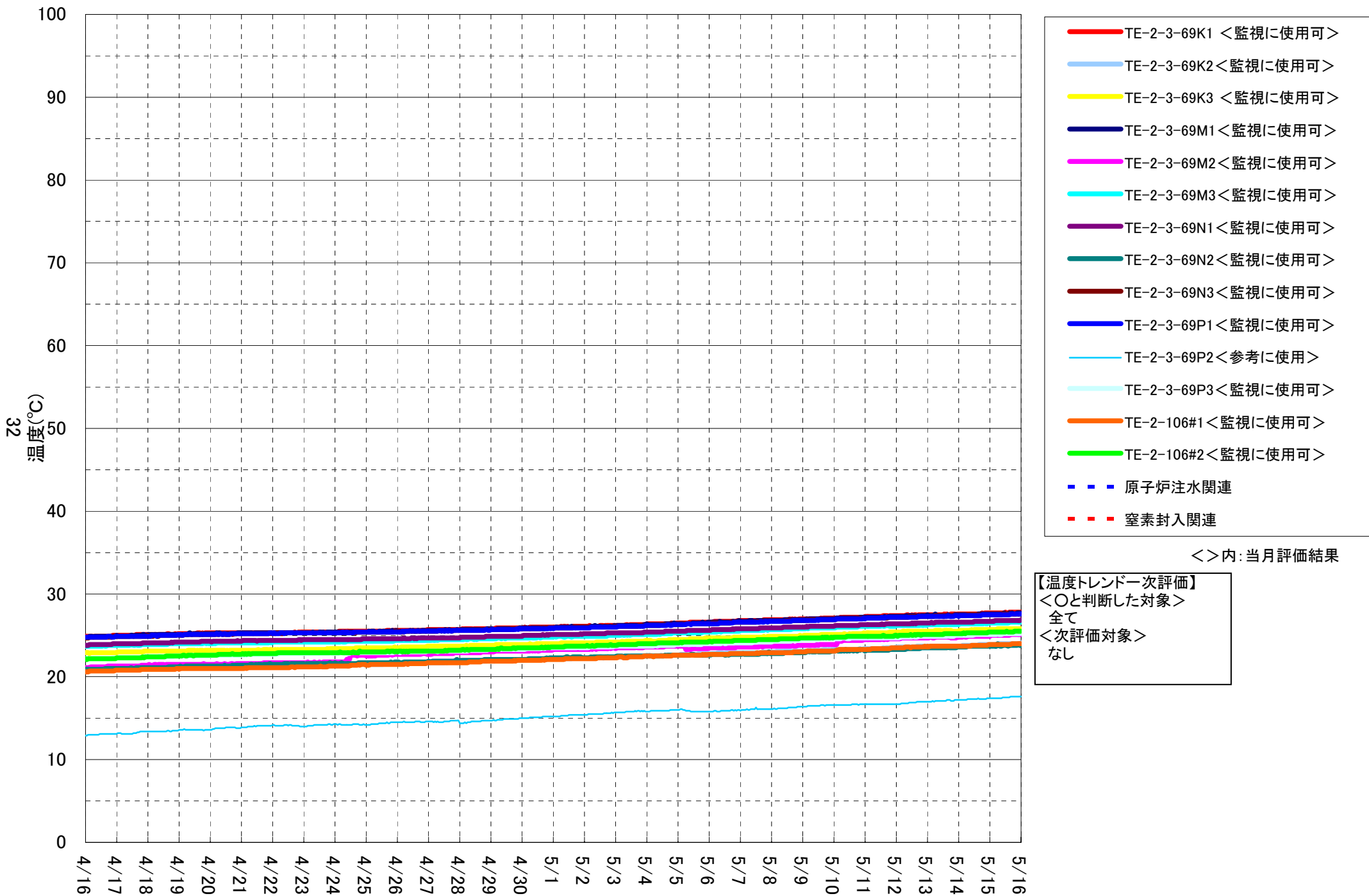
3号機 RPV周辺温度計(下部)
