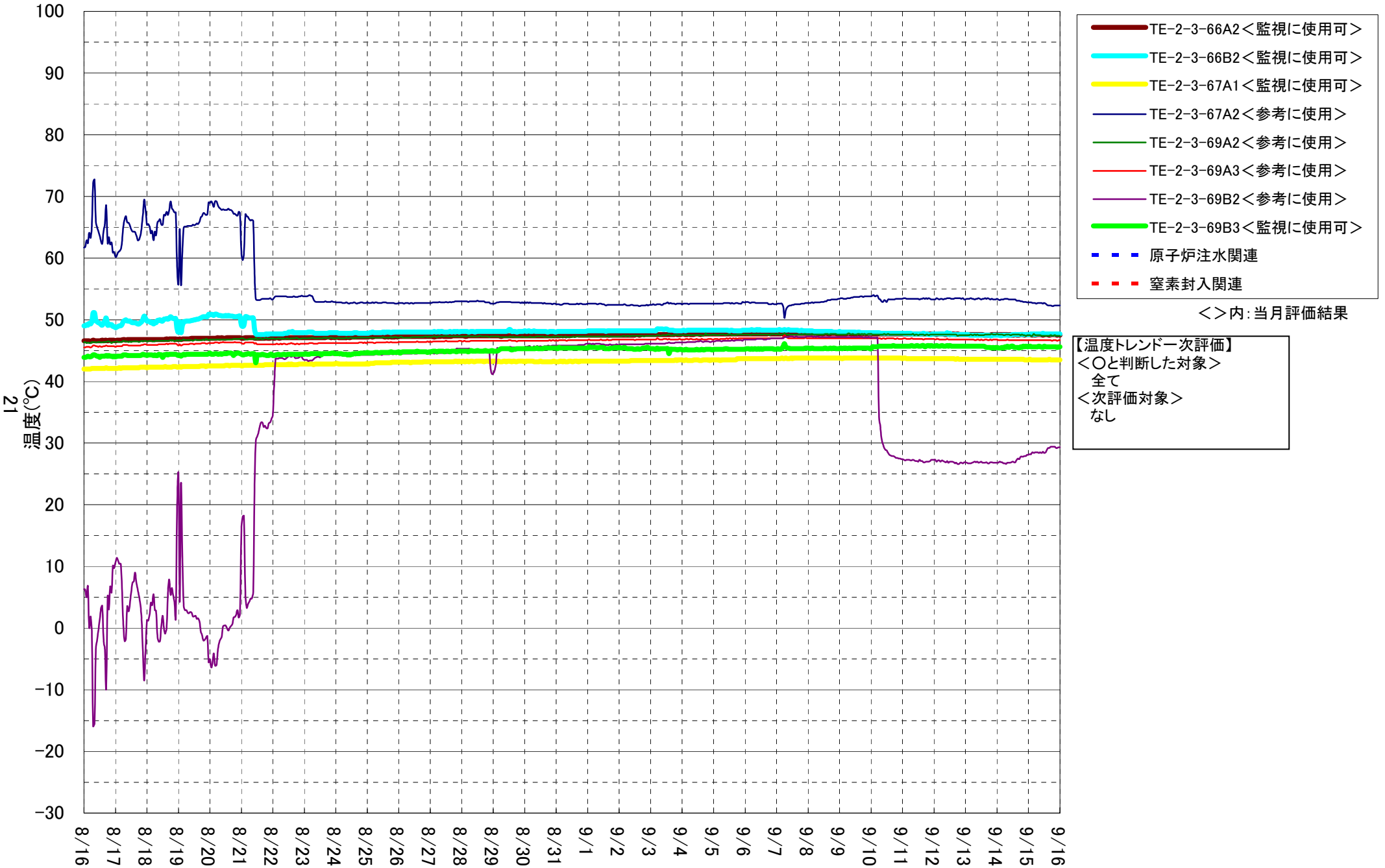
2号機 RPV周辺温度計(上部)①
