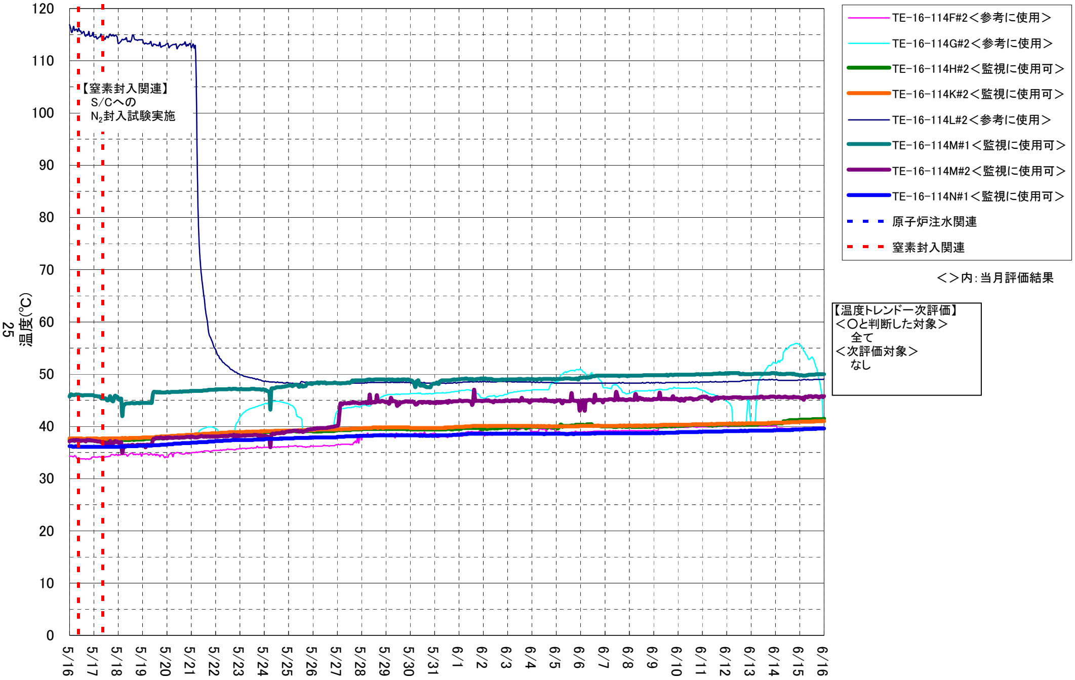
2号機 PCV内温度計②
