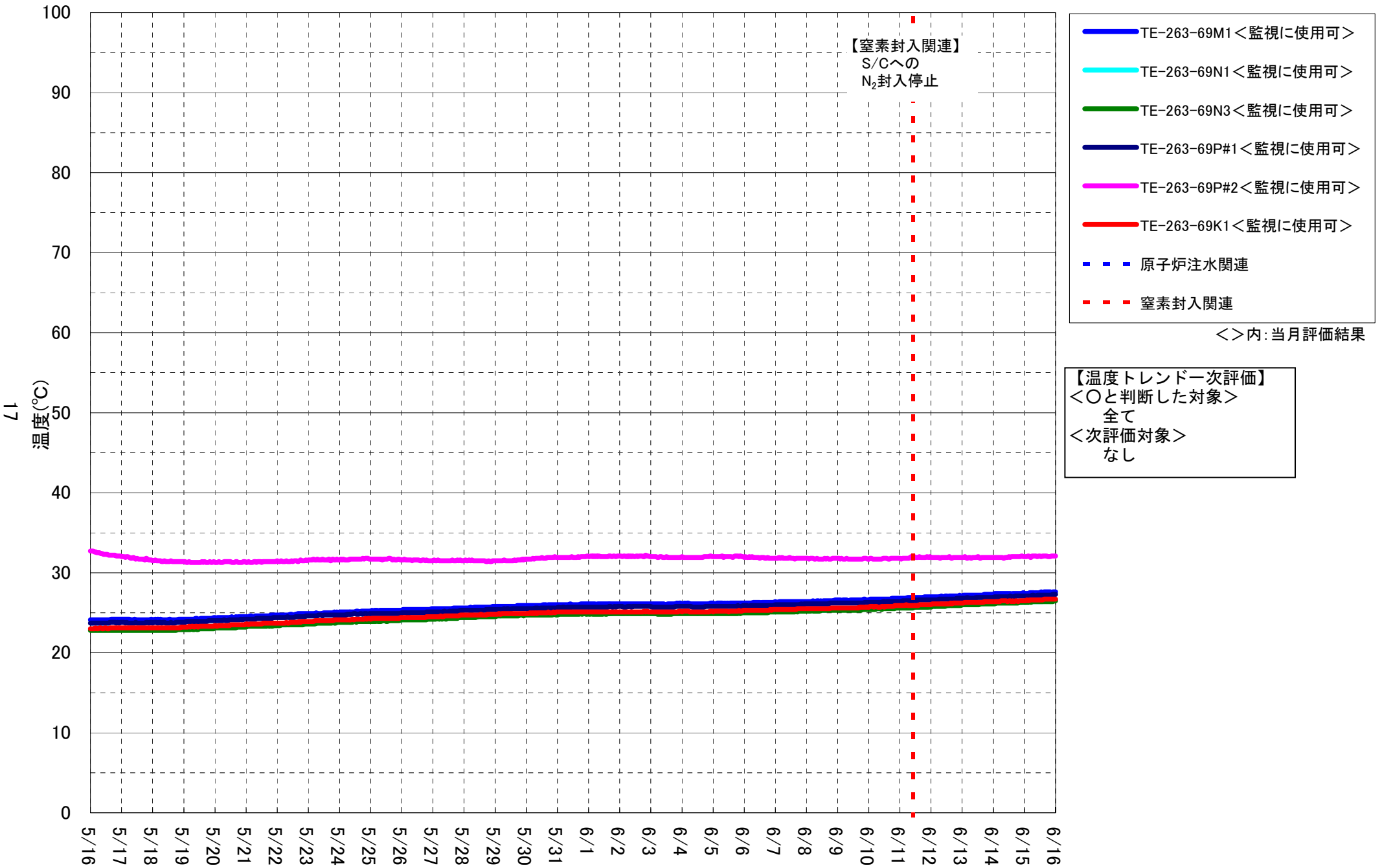
1号機 RPV周辺温度計(下部)
