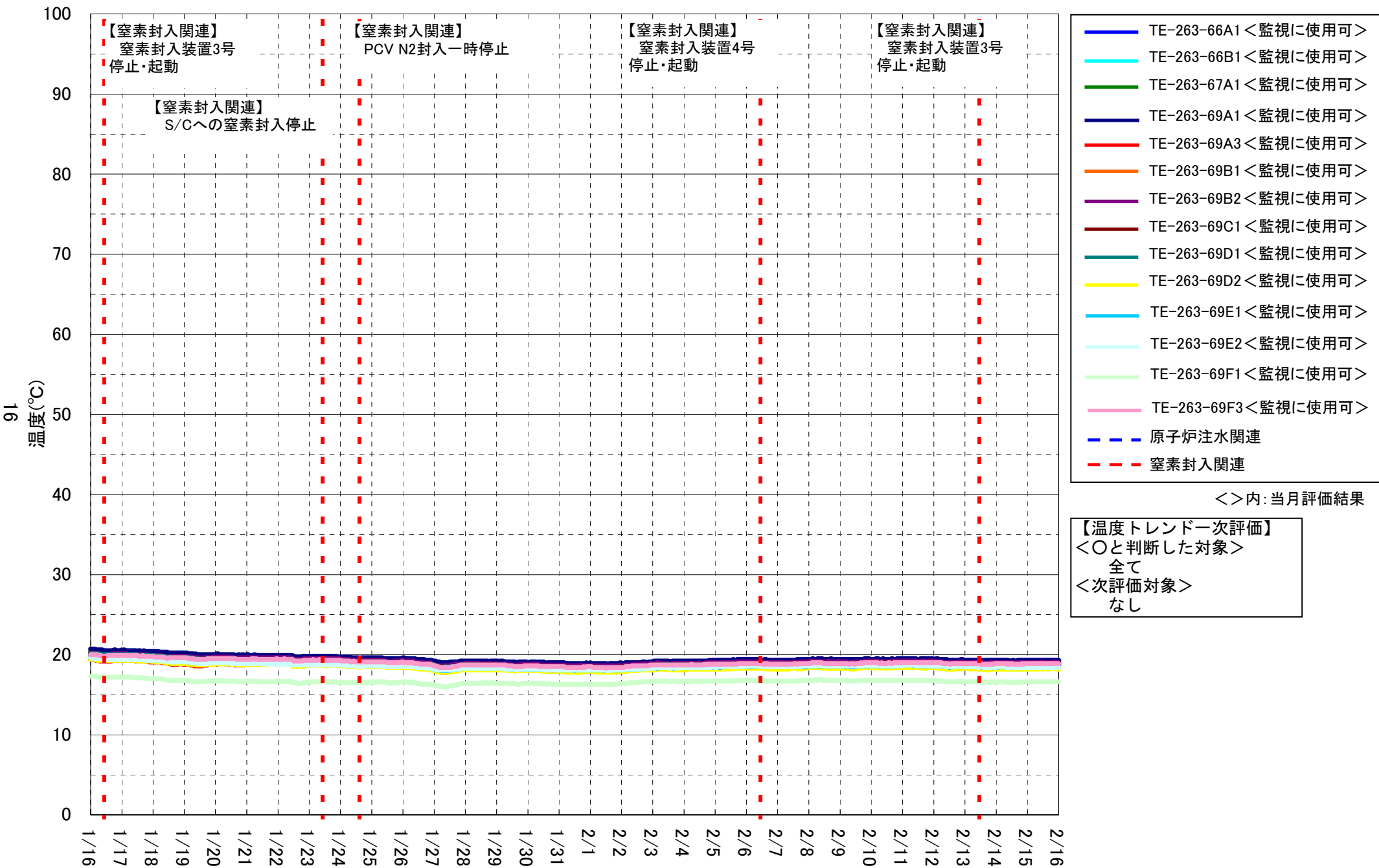
1号機 RPV周辺温度計(上部)
