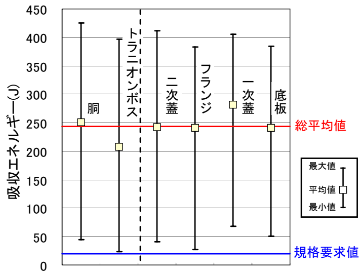
図 2-3 吸収エネルギーデータ (-59.4°C) —シャルピー衝撃試験結果—
