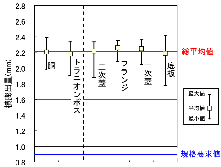
図 2-4 横膨出量データ (-17°C) —シャルピー衝撃試験結果—
