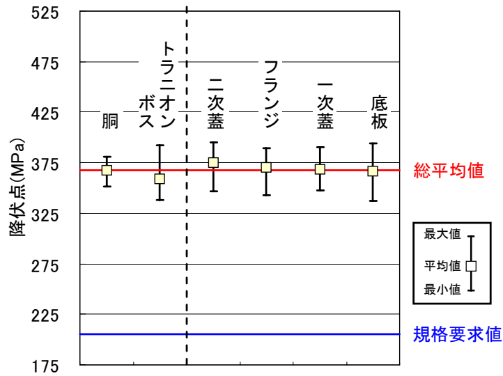
図 2-5 降伏点データ —引張試験結果—
