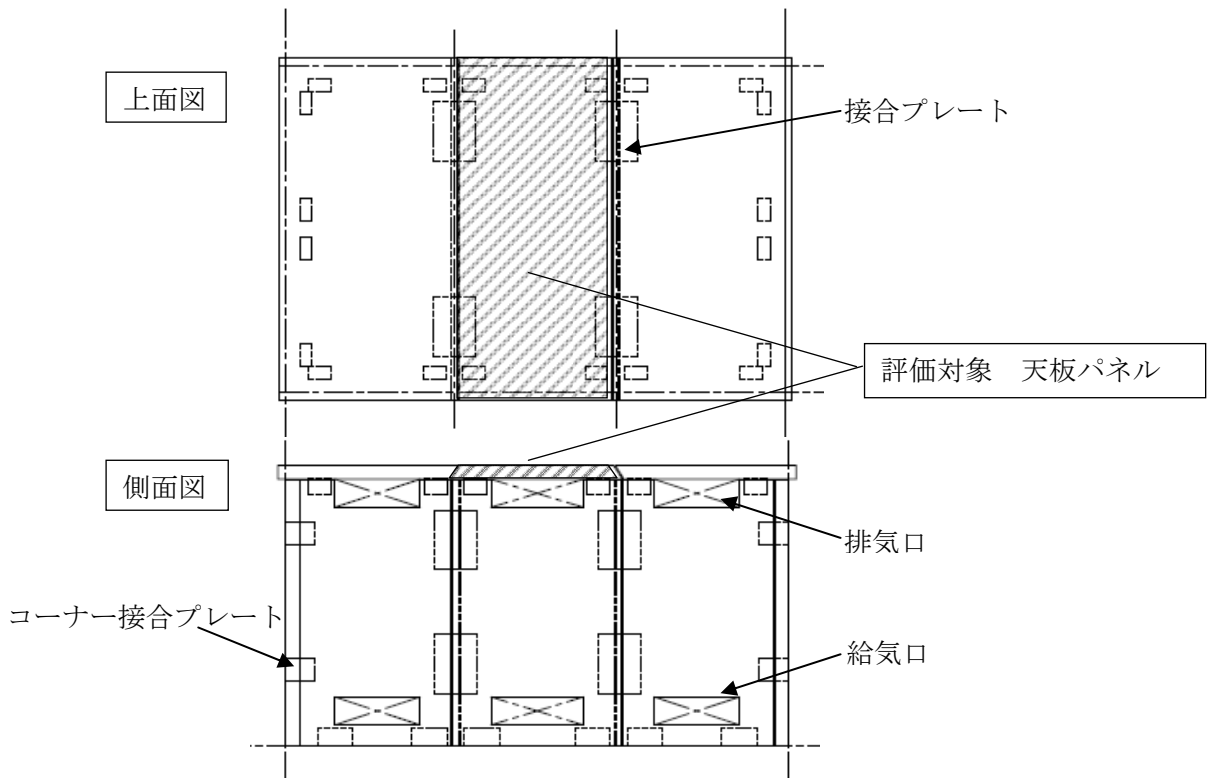
図 3.5.3-4 天板パネル
