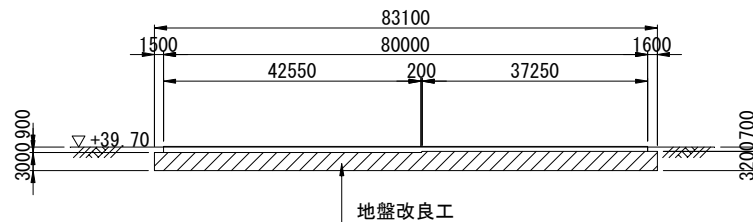
図 3.6.6-13 1-1 断面 (単位: mm)
