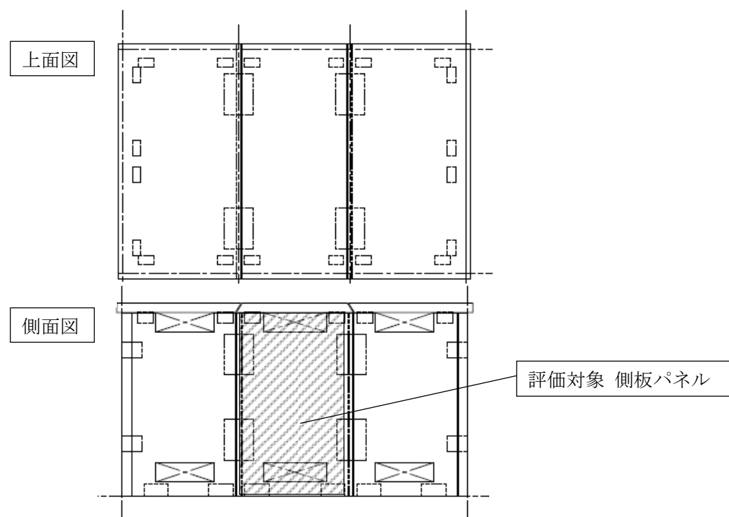
図 3. 5. 3-5 側板パネル
