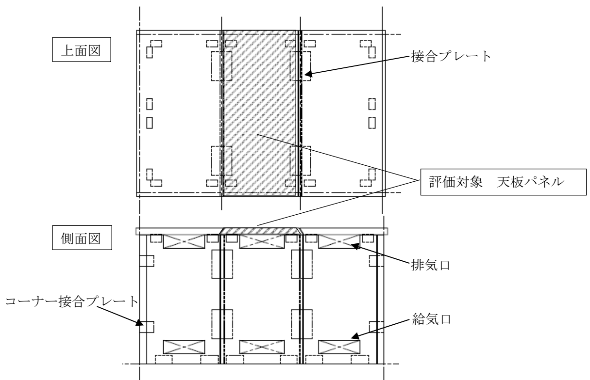
図 3.6.4-7 天板パネル
