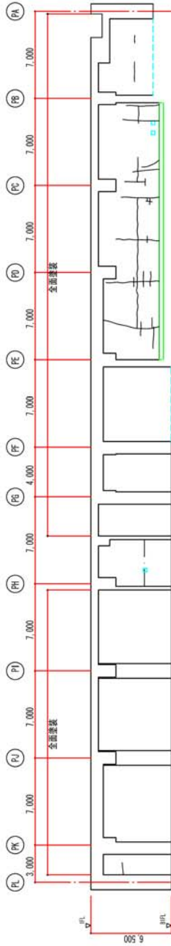
F1-7 地下建屋-B1F-N (P14通り)
