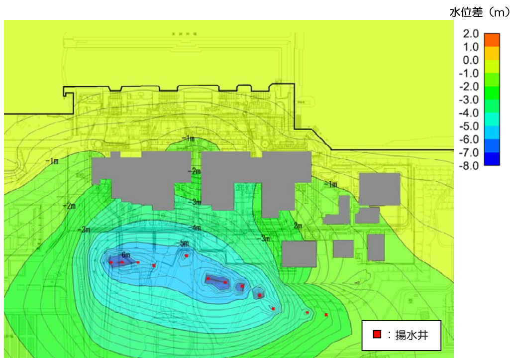
図－5 浸透流解析結果（現状と稼働後の差分）
