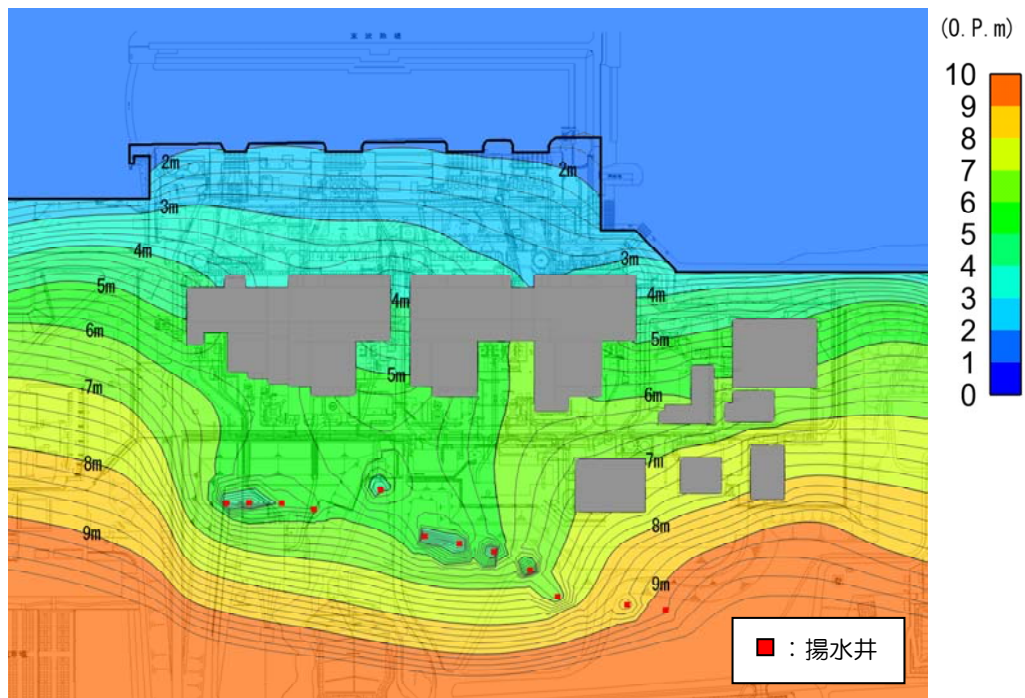
図-4 浸透流解析結果（地下水バイパス稼働後）
