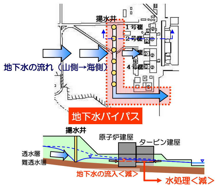
図一 地下水バイパス (イメージ)
