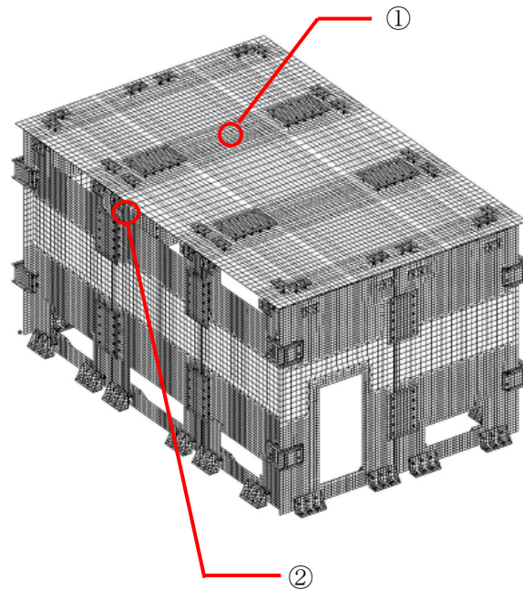
図 3.5.3-3 応力評価箇所
