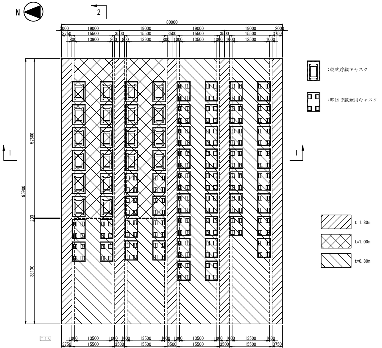
図 3. 5. 4-2 基礎平面図 (単位 : mm)
