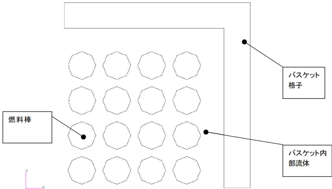
図 3. 1. 1-7 燃料集合体断面モデル(乾式貯蔵キャスク(大型キャスク))
