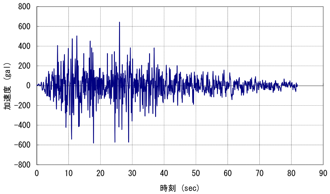
图 3.6.5-10 地表面時刻歷波形水平方向 Ss-1
