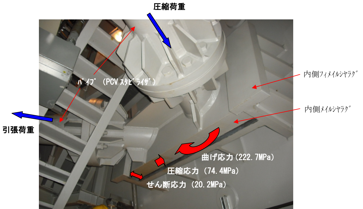
図2 内側メイルシヤラグの応力状態
