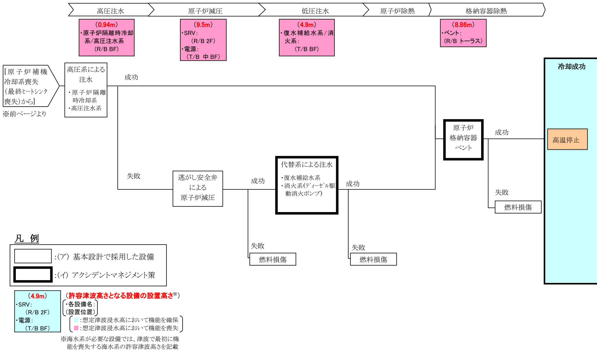
図 4-3(2/3) 津波の起因事象に対するイベントツリーと津波浸水高 15m 時の事象進展(1F5 原子炉)
