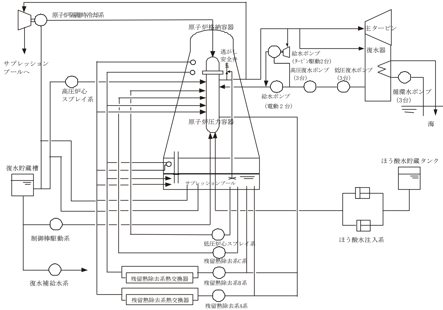
図 2 - 2 柏崎刈羽 1 号機の設備構成の概要図
