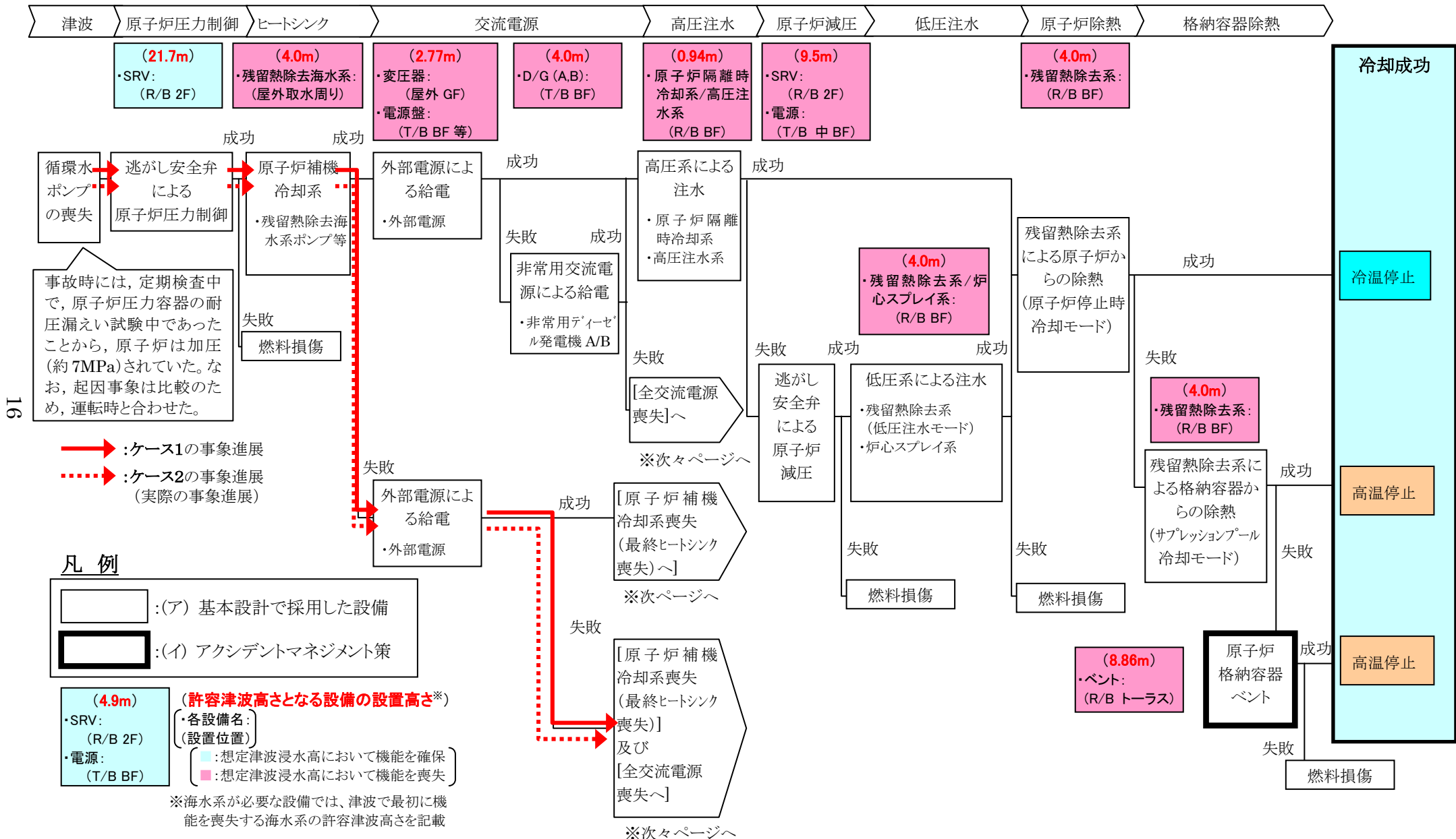
図 4-3(1/3) 津波の起因事象に対するイベントツリーと津波浸水高 15m 時の事象進展 (1F5 原子炉)
