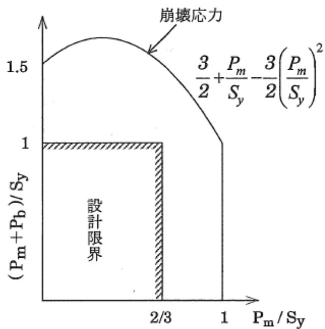
図3 引張りおよび曲げによる崩壊応力および設計限界 (設計・建設規格 解説図 PVB-3111-2)
