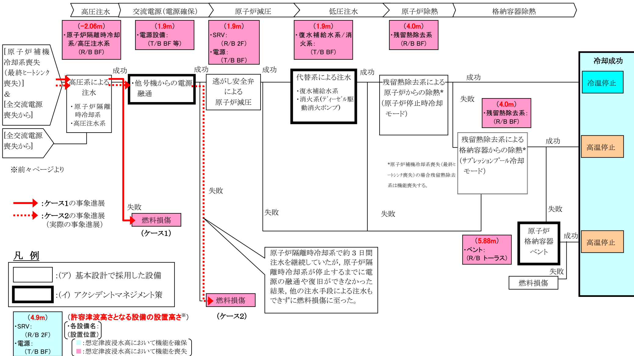
図 4-2(3/3) 津波の起因事象に対するイベントツリーと津波浸水高 17m 時の事象進展 (1F2 原子炉)
