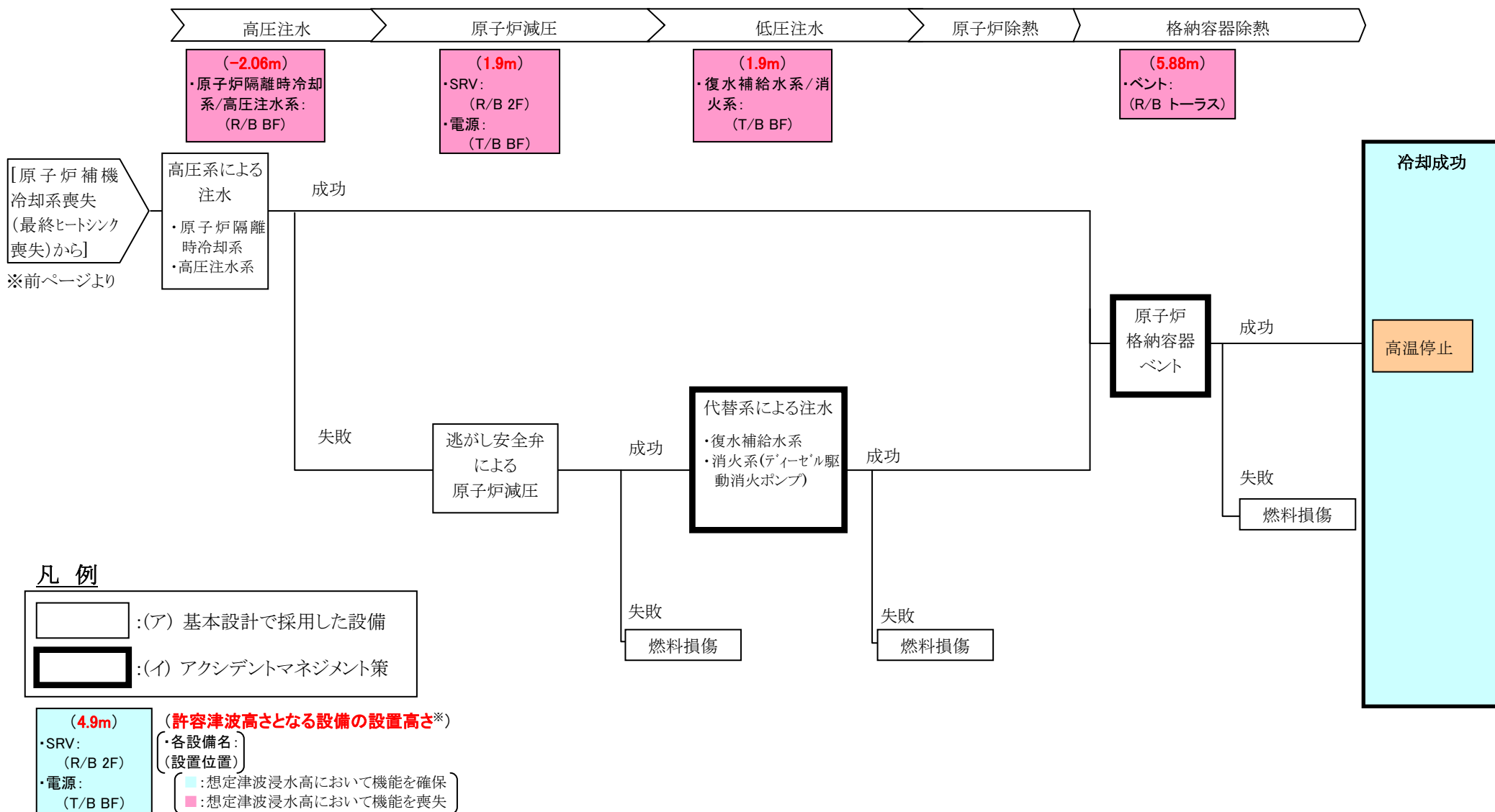
図 4-2(2/3) 津波の起因事象に対するイベントツリーと津波浸水高 17m 時の事象進展 (1F2 原子炉)
