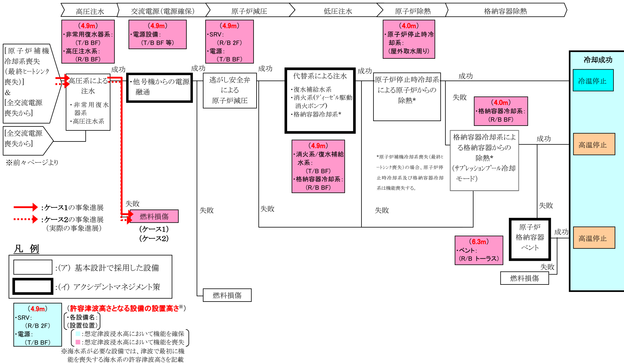
図 4-1(3/3) 津波の起因事象に対するイベントツリーと津波浸水高 17m 時の事象進展(1F1 原子炉)
