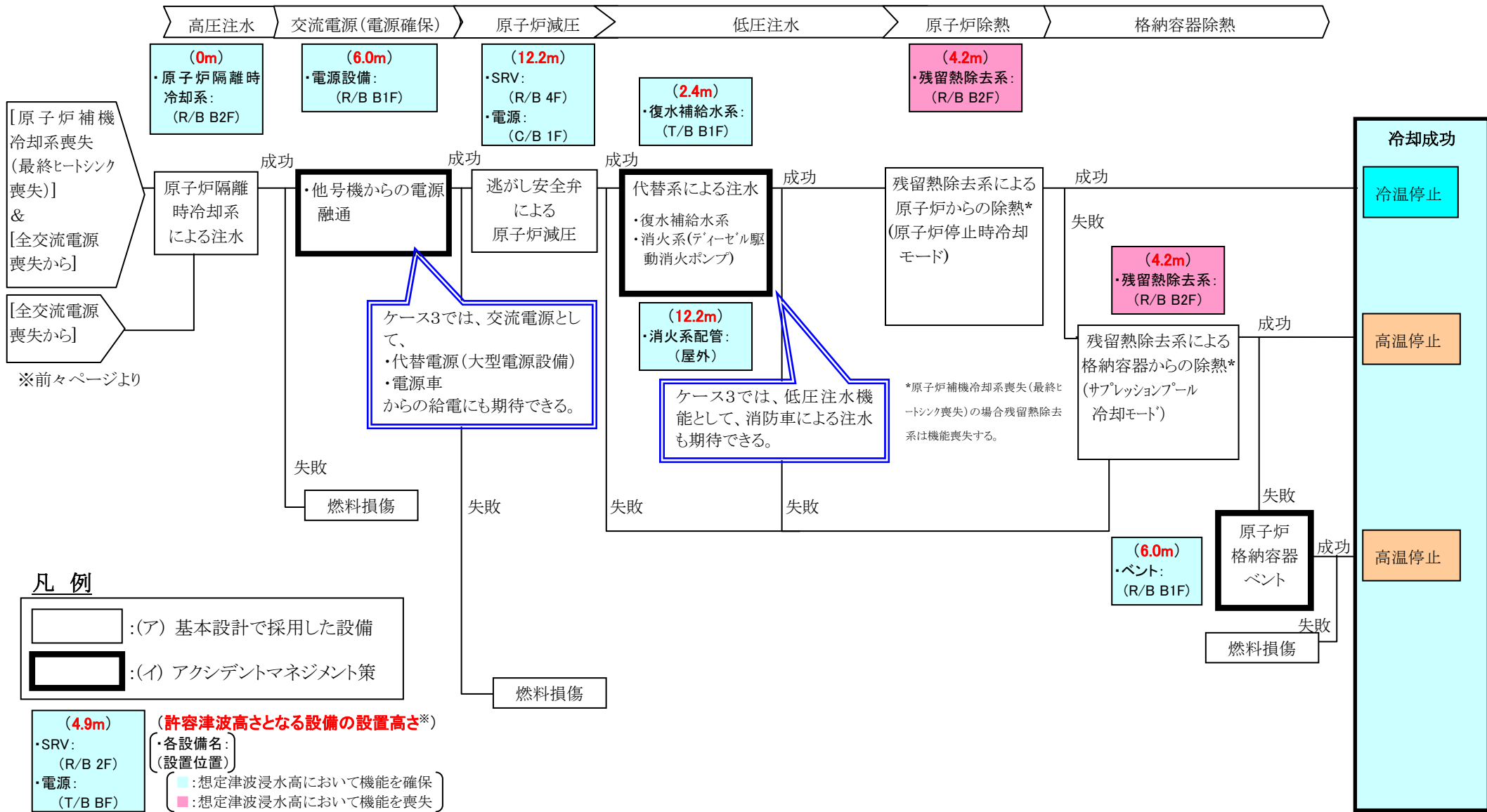
図 4-4(3/3) 津波の起因事象に対するイベントツリーと津波浸水高 7m 時の事象進展(2F1 原子炉)
