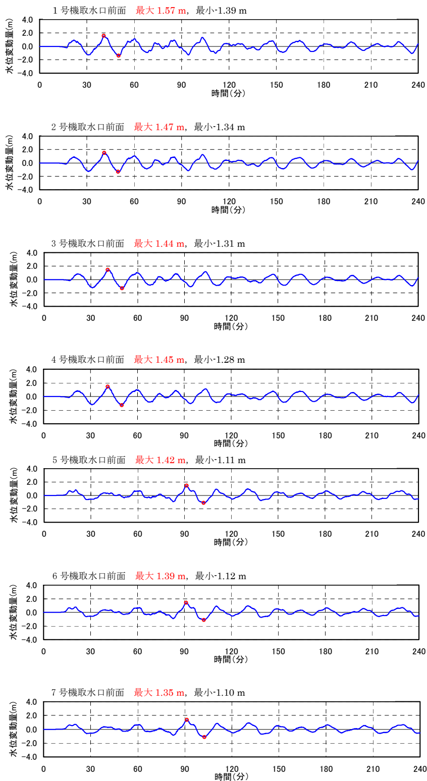
第2. 2-4 図(1) 海域活断層による津波の取水口前面における 水位時刻歴 (最大水位上昇量ケース)
