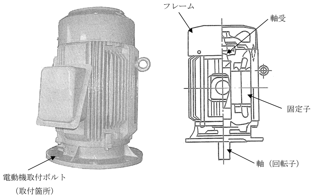
図 1 立形ころがり軸受電動機構造図の例
