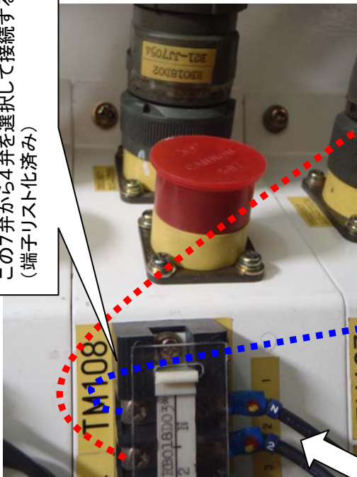
SRV電磁弁回路 (PCVより)
