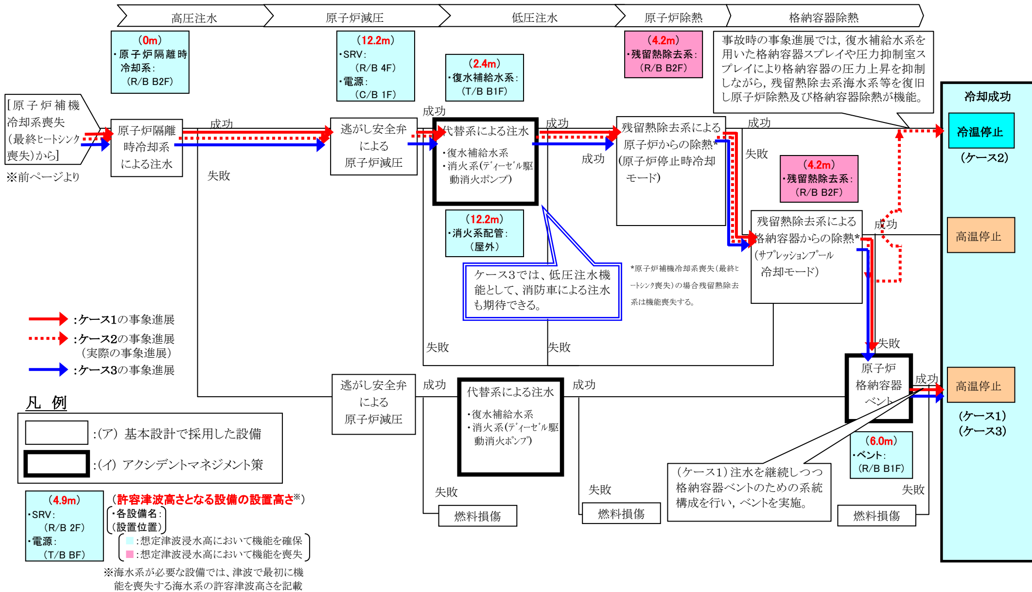
図 4-4(2/3) 津波の起因事象に対するイベントツリーと津波浸水高 7m 時の事象進展 (2F1 原子炉)
