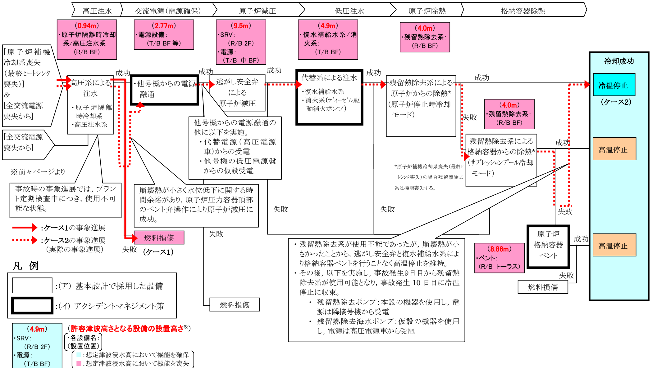
図 4-3(3/3) 津波の起因事象に対するイベントツリーと津波浸水高 15m 時の事象進展(1F5 原子炉)
