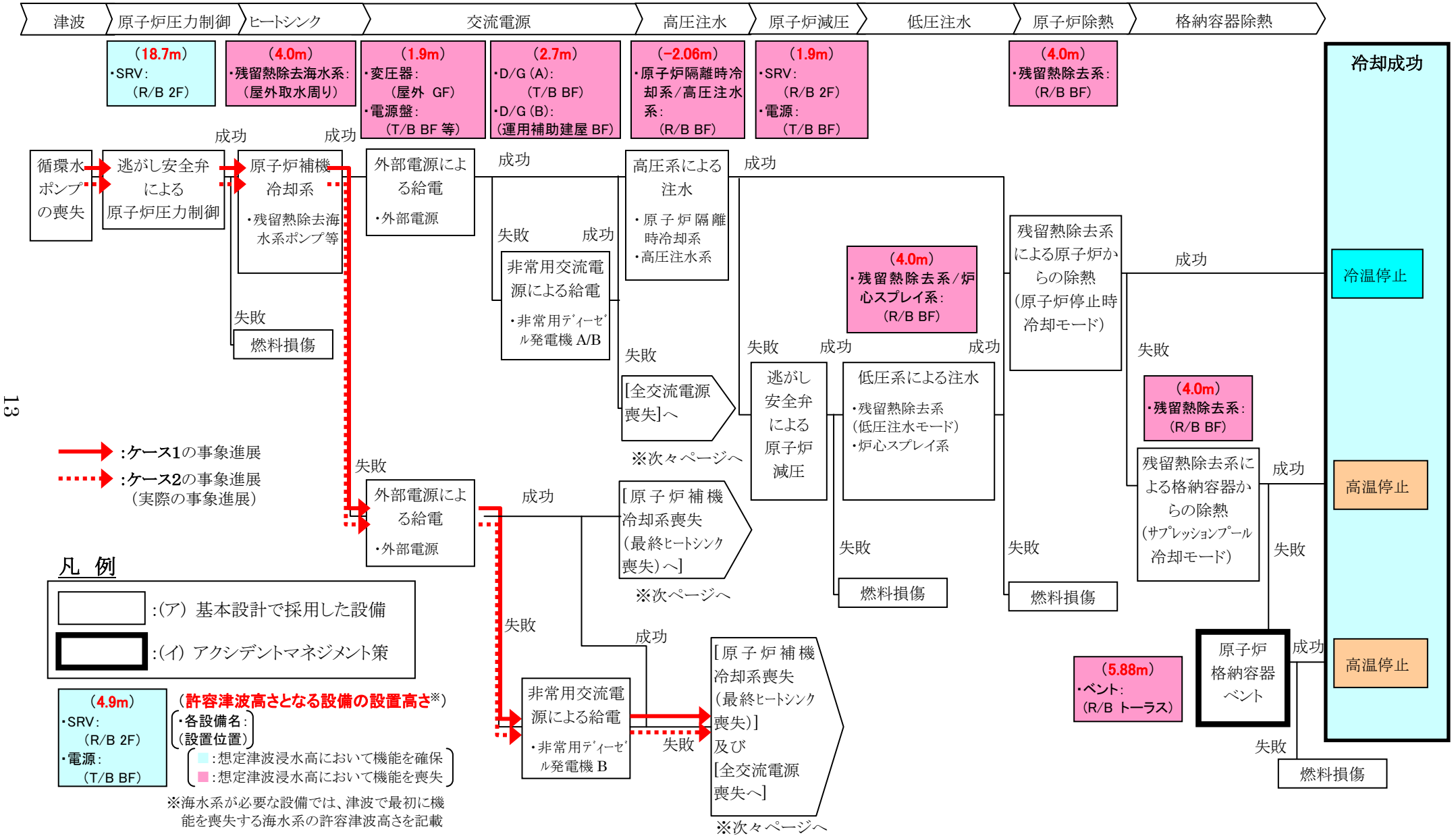
図 4-2(1/3) 津波の起因事象に対するイベントツリーと津波浸水高 17m 時の事象進展 (1F2 原子炉)
