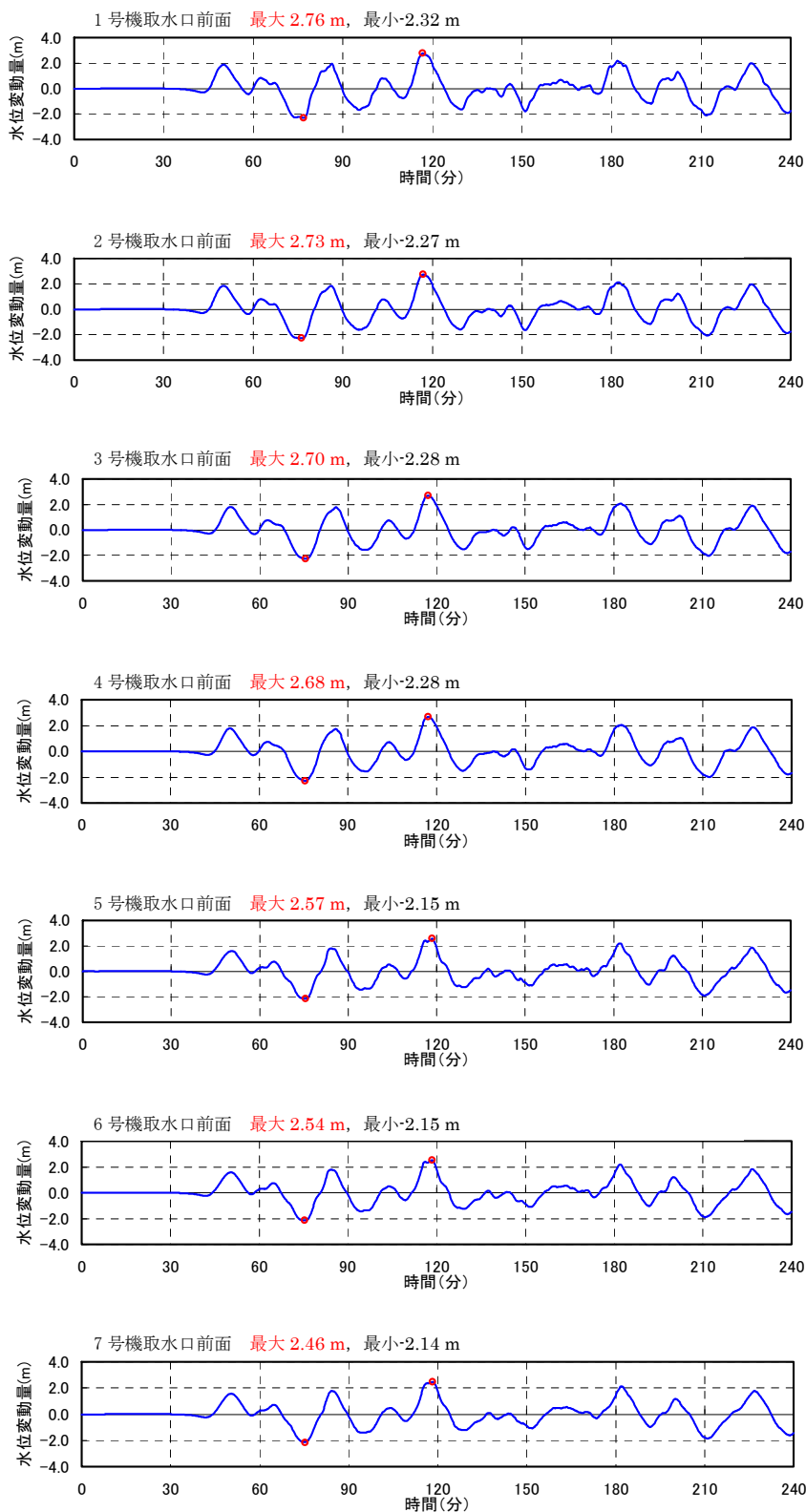
第2. 3-8 図(1) 日本海東縁部の想定津波による取水口前面の 水位時刻歴 (最大水位上昇量ケース)
