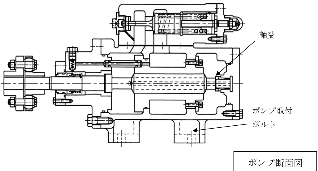
図2 燃料移送ポンプ構造図及び評価部位
