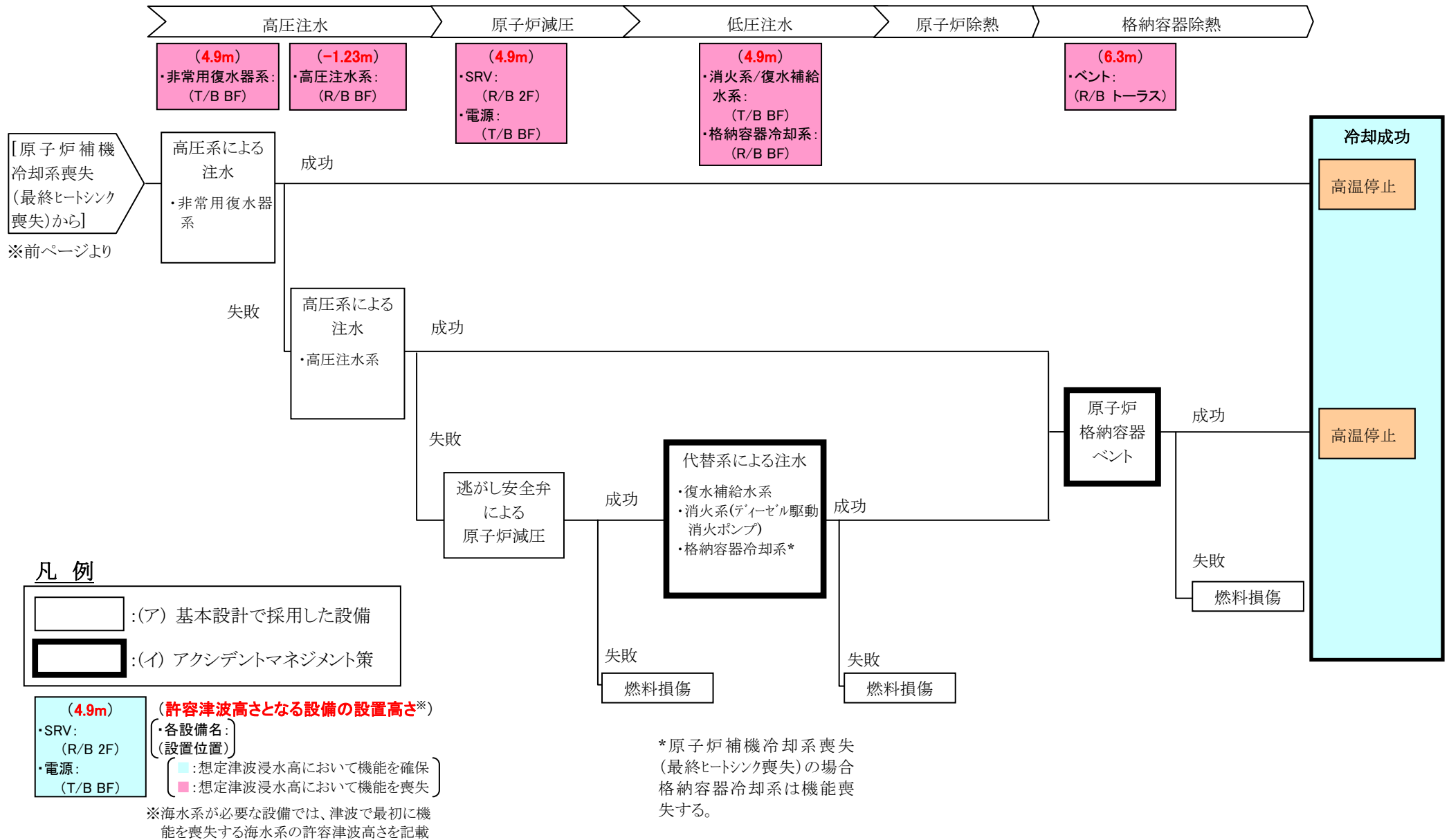
図 4-1(2/3) 津波の起因事象に対するイベントツリーと津波浸水高 17m 時の事象進展(1F1 原子炉)
