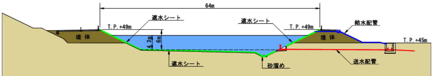
貯水池断面
