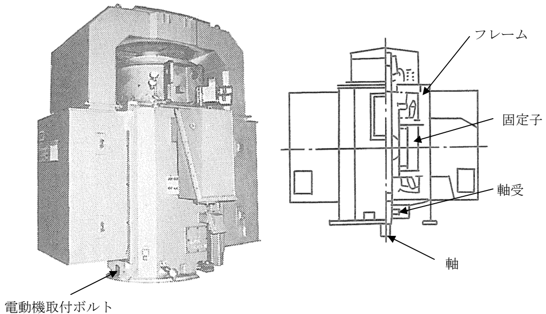
図2 立形すべり軸受電動機構造図の例
