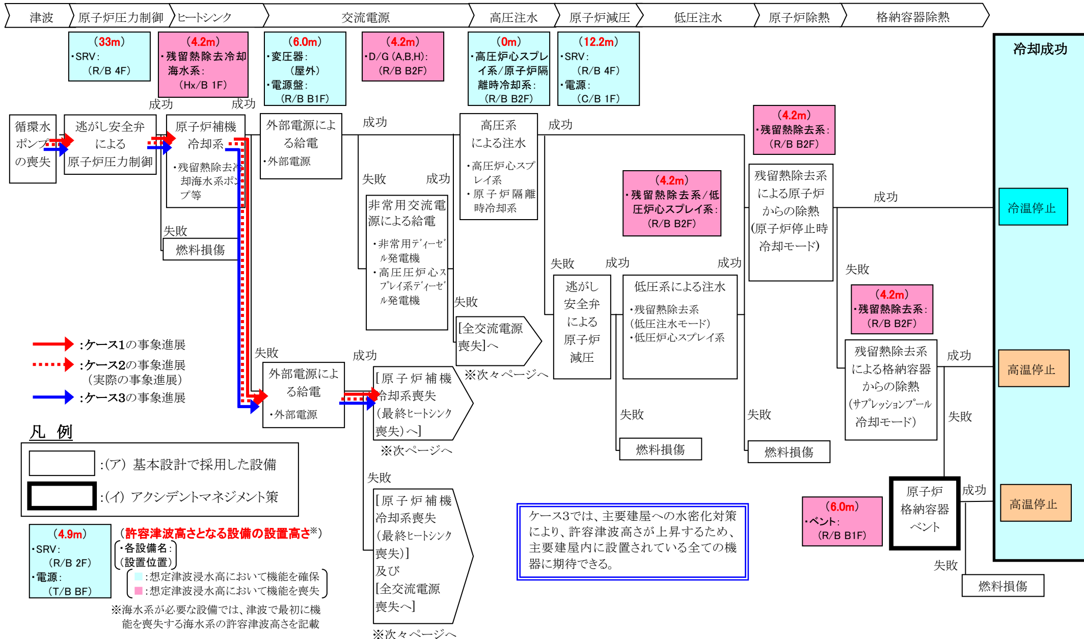
図 4-4(1/3) 津波の起因事象に対するイベントツリーと津波浸水高 7m 時の事象進展 (2F1 原子炉)
