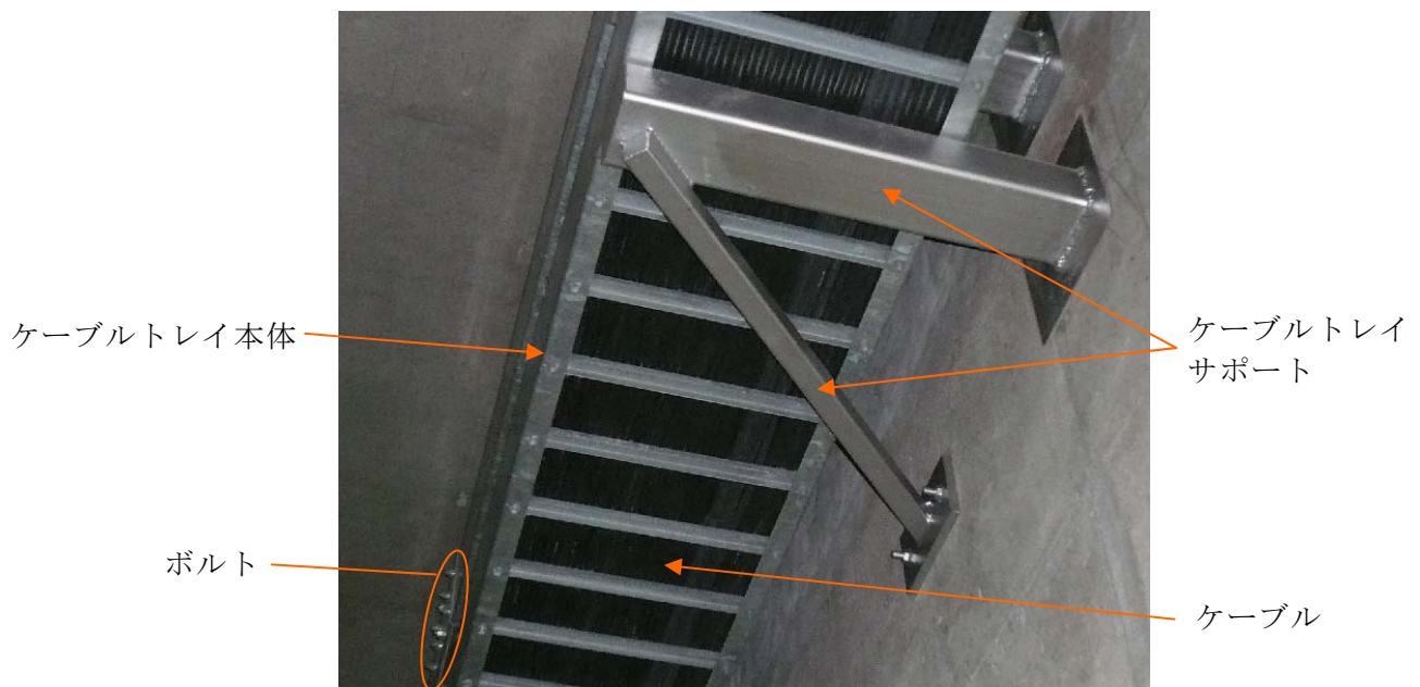
図1 ケーブルトレイの例 (ケーブルトレイ下からの写真)
