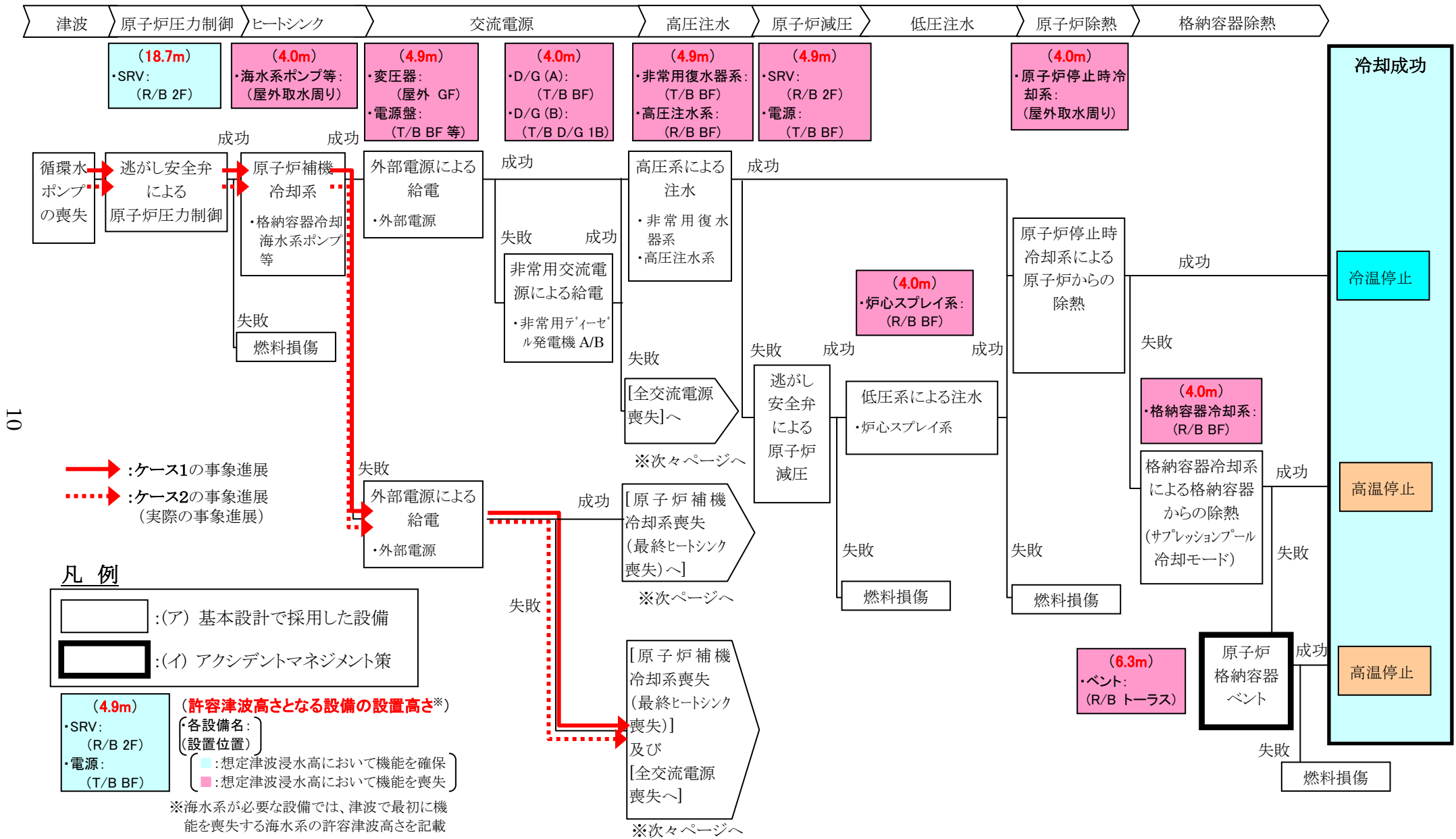
図 4-1(1/3) 津波の起因事象に対するイベントツリーと津波浸水高 17m 時の事象進展 (1F1 原子炉)
