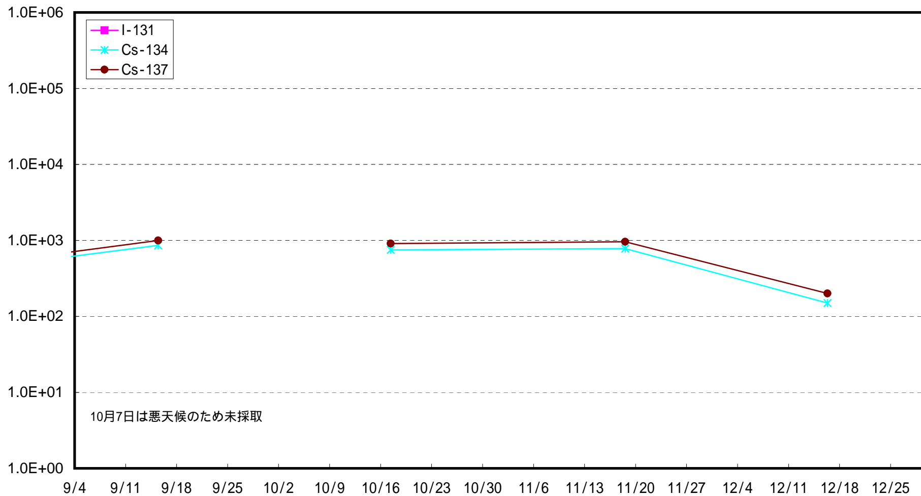
岩沢海岸沖合3km海底土放射能濃度 (Bq / kg・湿土)
