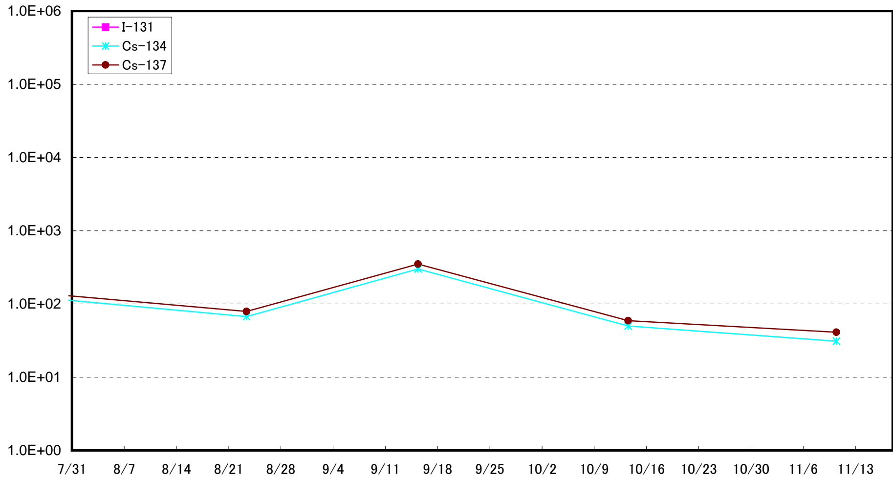
小高区冲合3km海底土放射能濃度(Bq/kg·湿土)
