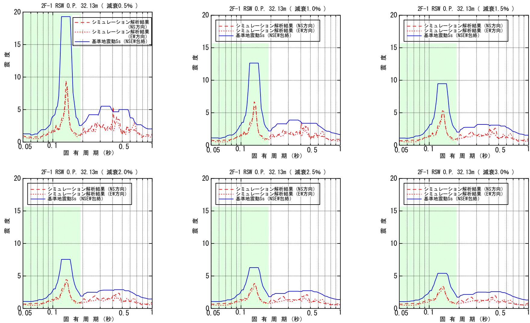
図-4.4.3.8 原子炉遮へい壁 O.P. 32.13m 床応答スペクトル (水平方向)
