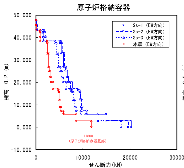
図-4.4.2.2.1 最大応答せん断力 (NS, EW 方向) (原子炉格納容器, 原子炉圧力容器 及び原子炉本体基礎)
