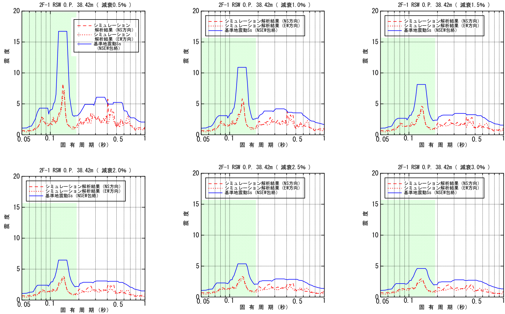
図-4.4.3.7 原子炉遮へい壁 O.P. 38.42m 床応答スペクトル (水平方向)
