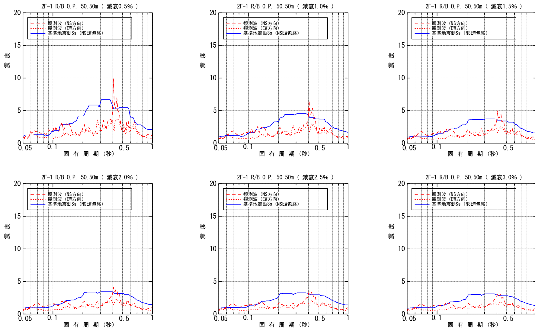
図-4.4.3.1 原子炉建屋 O.P. 50.50m 床応答スペクトル (水平方向)
