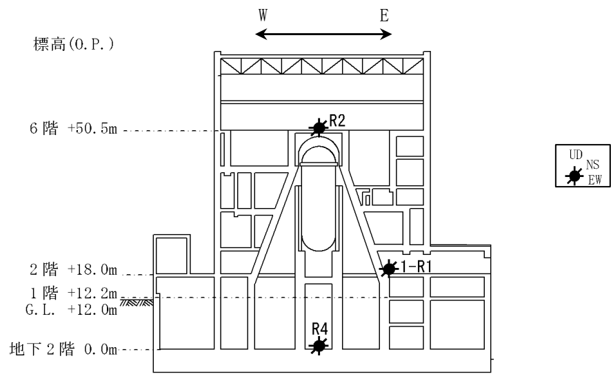
(a) 断面図
