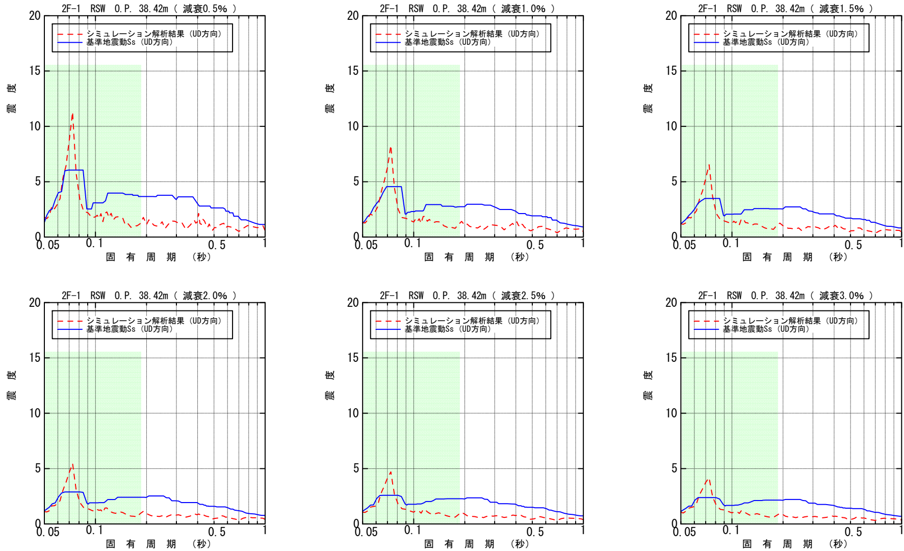
図-4.4.3.10 原子炉遮へい壁 O.P. 38.42m 床応答スペクトル (鉛直方向)
