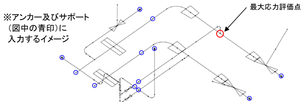
残留熱除去系配管モデル (一部)
