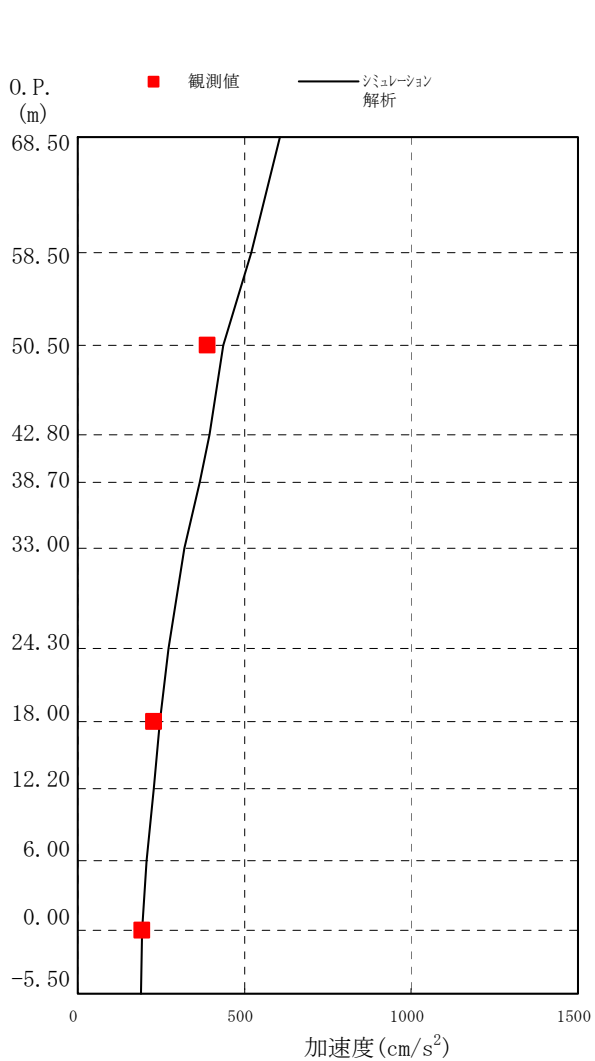
図-3. 5. 1 (3) 最大応答加速度 (鉛直方向)
