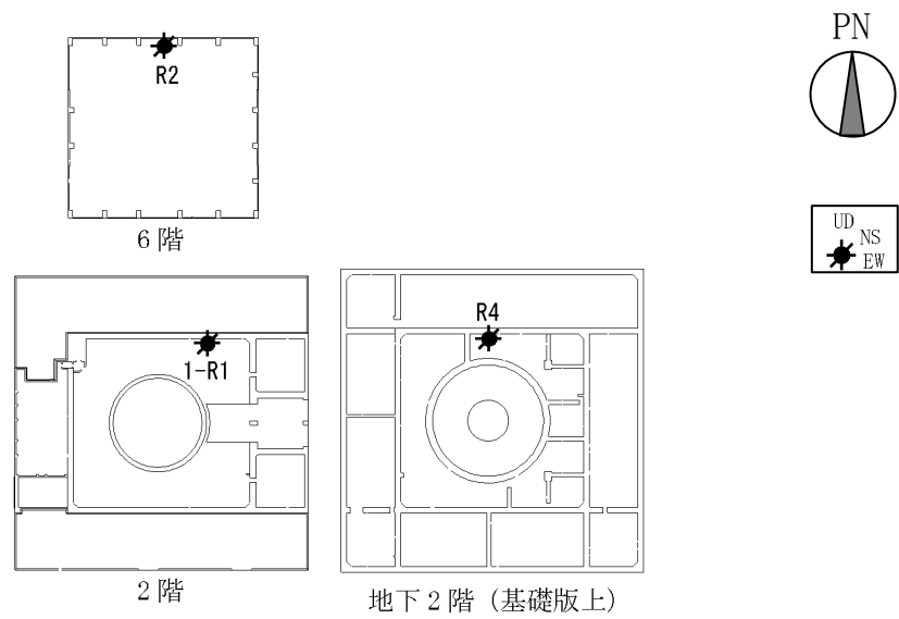
(b) 平面図
