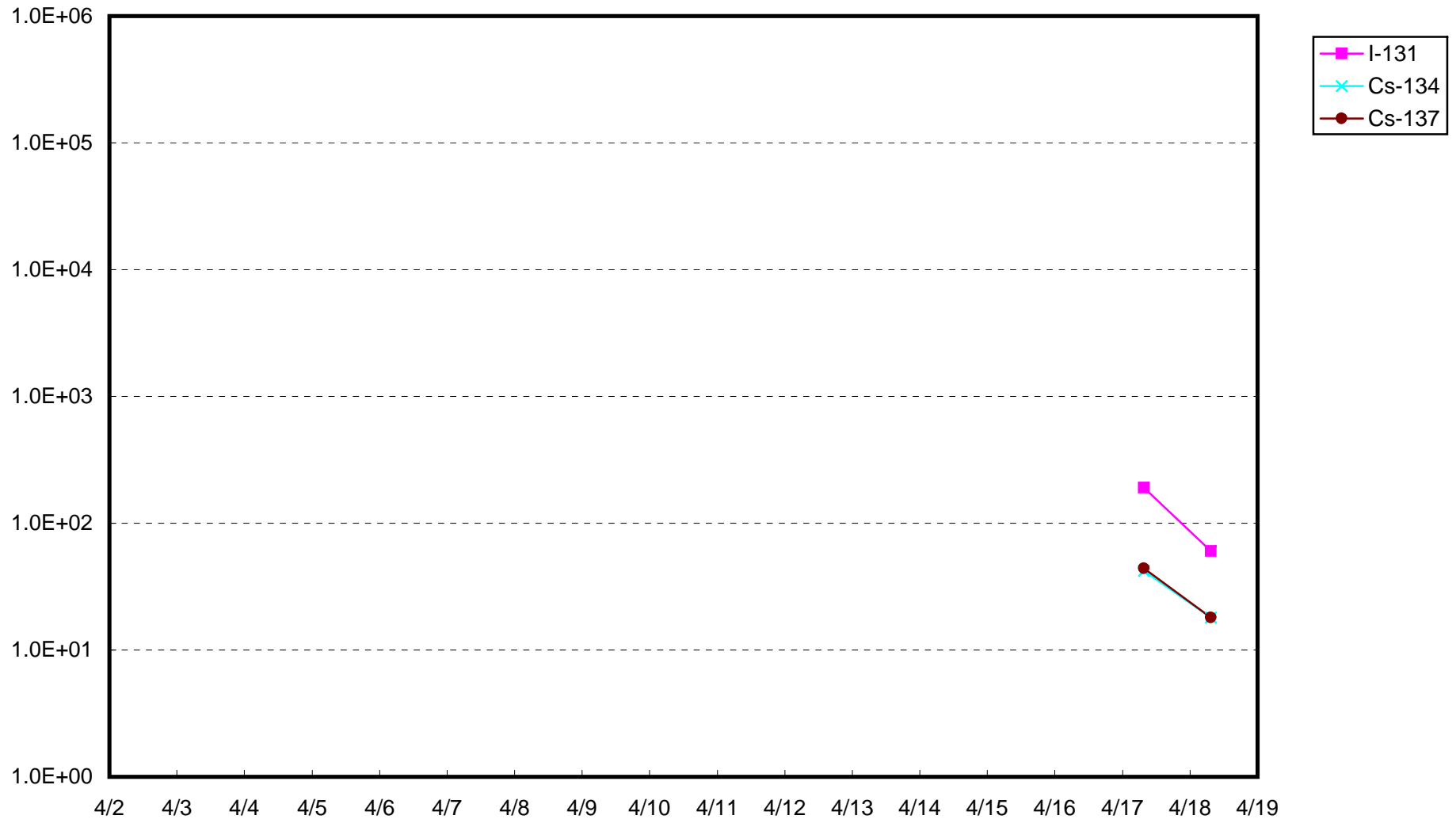
福島第一 2号機バースクリーン付近海水放射能濃度(シルトフェンス外側) (Bq / cm 3 )
