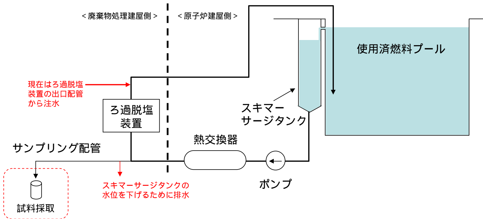
【燃料プール冷却浄化系統図】
