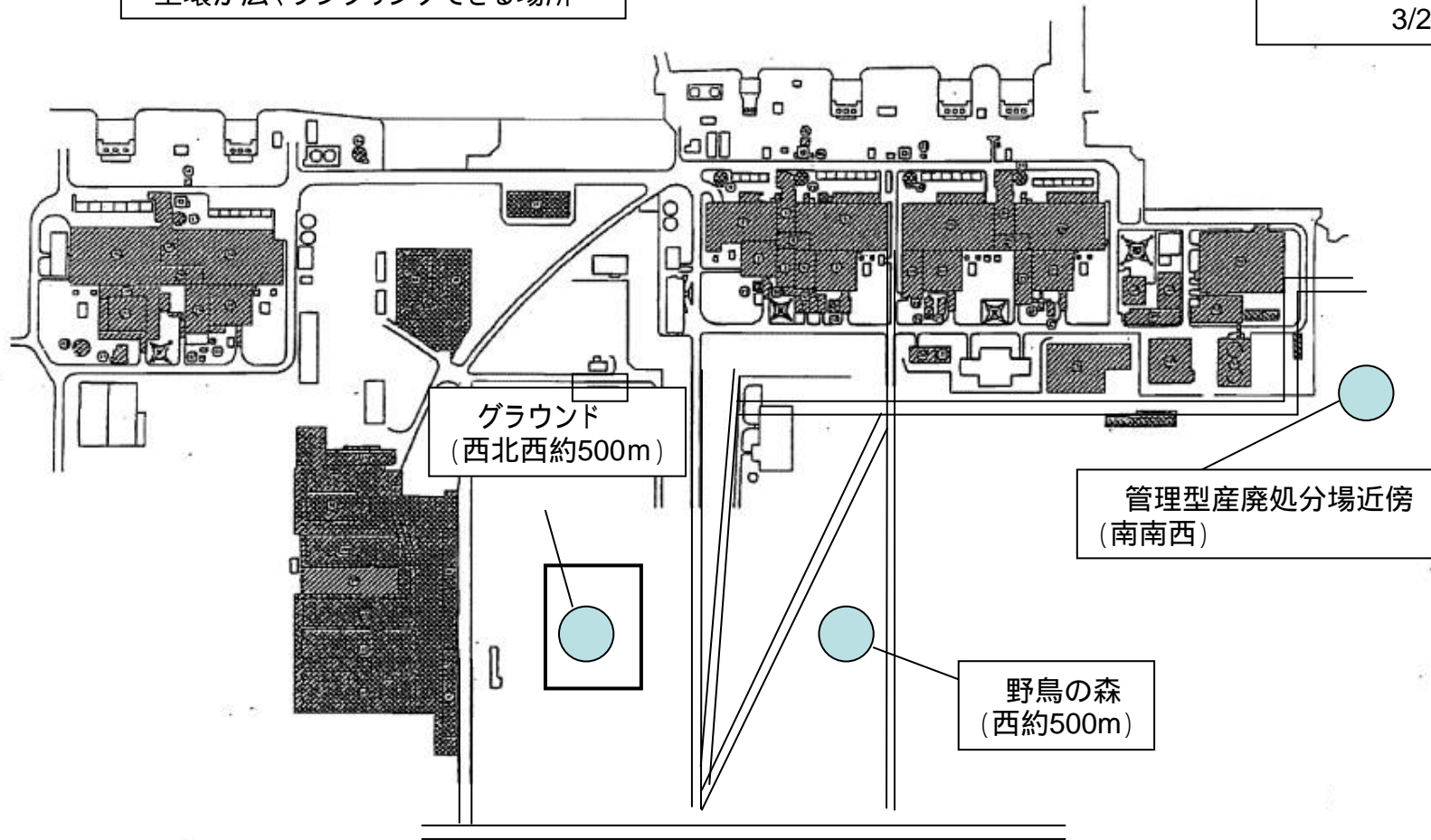
図面名称 福島第一原子力発電所 管理区域全体図
