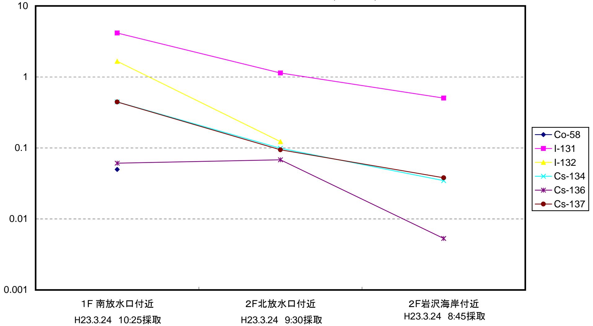
海水放射能濃度(Bq/cm 3 ) (H23.3.24)
