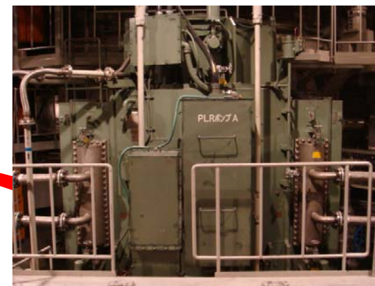
原子炉冷却材再循環ポンプ 電動機(2台)
