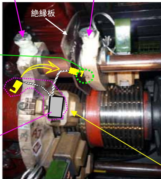
励磁機点検口内部
