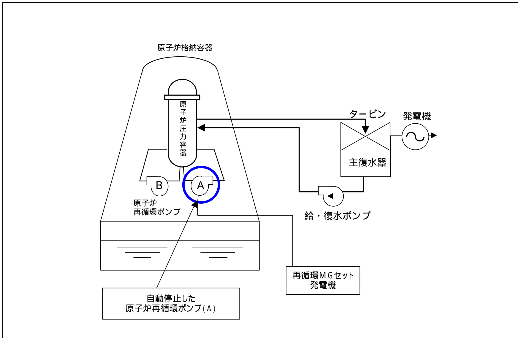
4号機系統概略図
