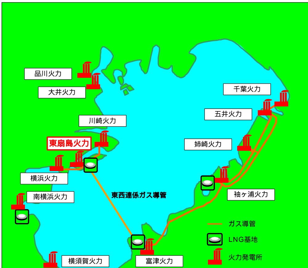
東扇島火力発電所と東京湾岸の当社火力発電所の位置関係
