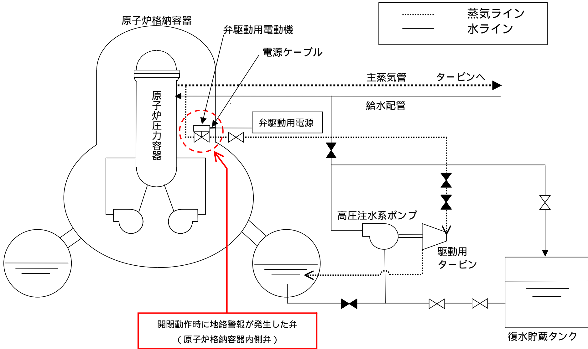
福島第一原子力発電所 3号機 高圧注水系系統概略図
