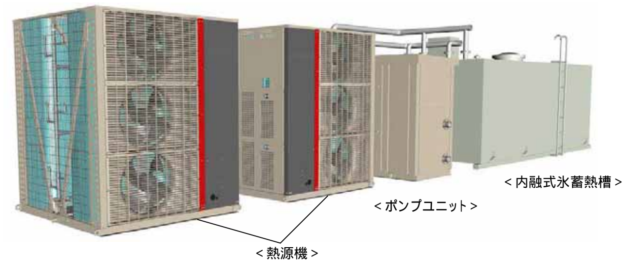
機器設置例(120馬力ユニットの場合)
