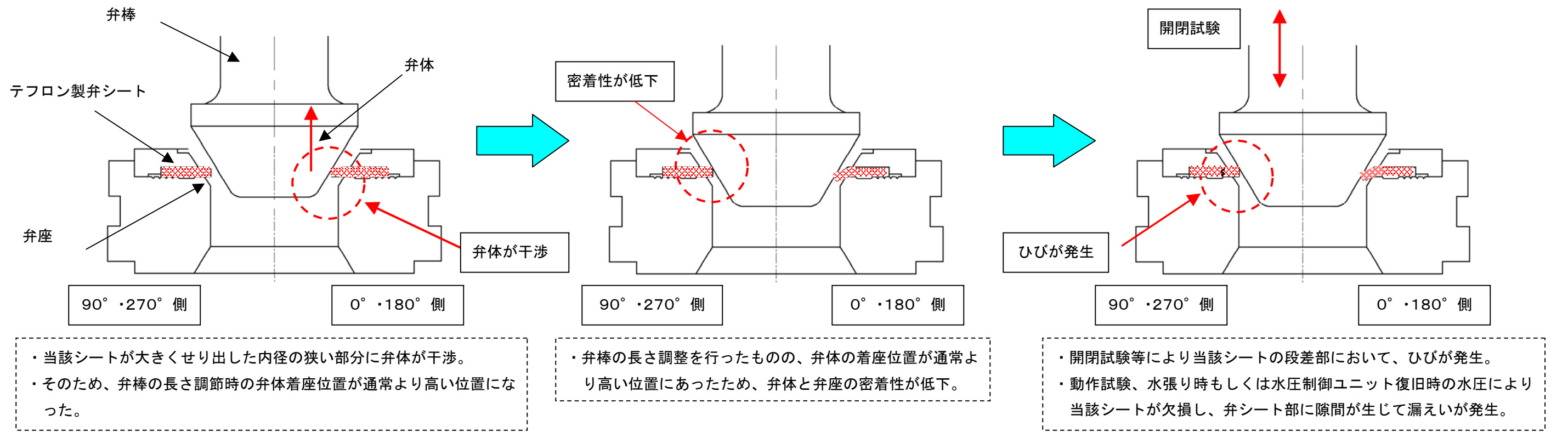
弁シート部漏えいのメカニズム
