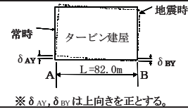
参表-5.4.13 (2) タービン建屋基礎底面の鉛直方向の相対変位・傾斜 (汀線直交断面)
