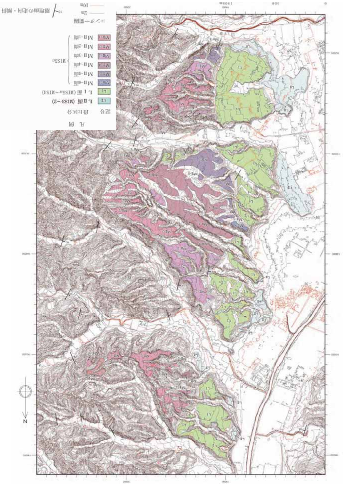
参图-3.1.7 渡海川右岸の段丘面分布図
