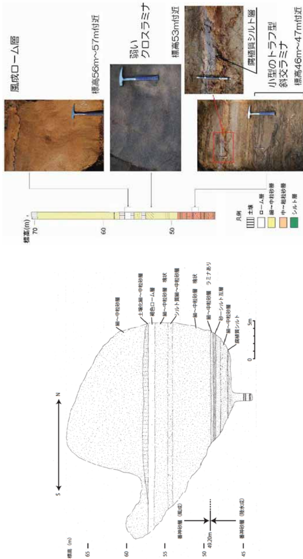
参図-3.4.4.2 Loc. f (大塚山露頭) 調査結果
