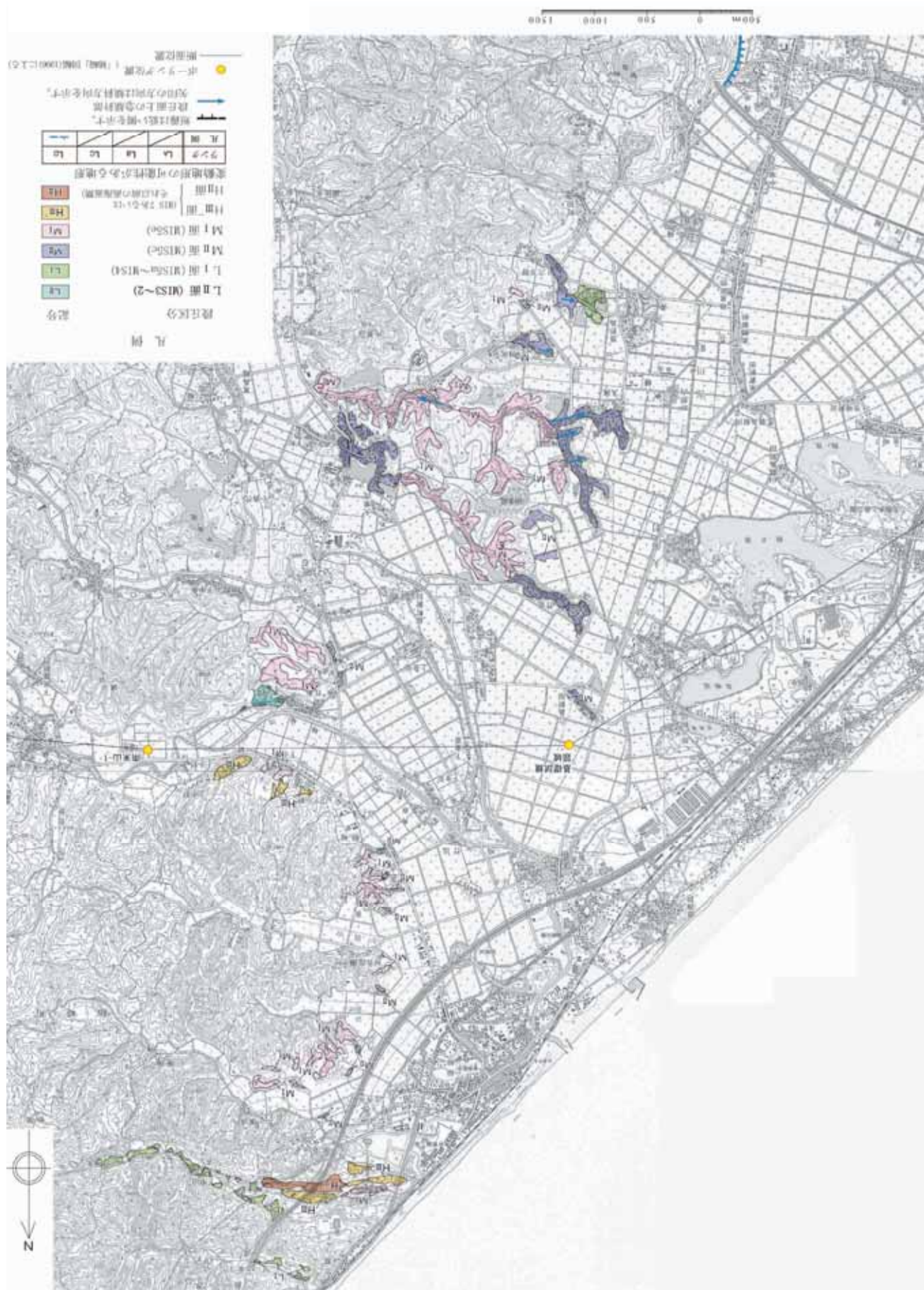
参図-3.2.5 高田平野東縁断層北方延長部の空中写真判読結果
