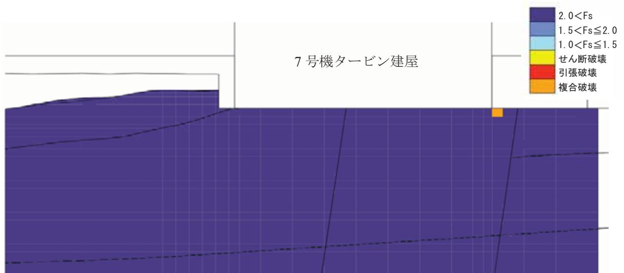
要素ごとの安全係数 (破壊表示は当該時刻で判定)
