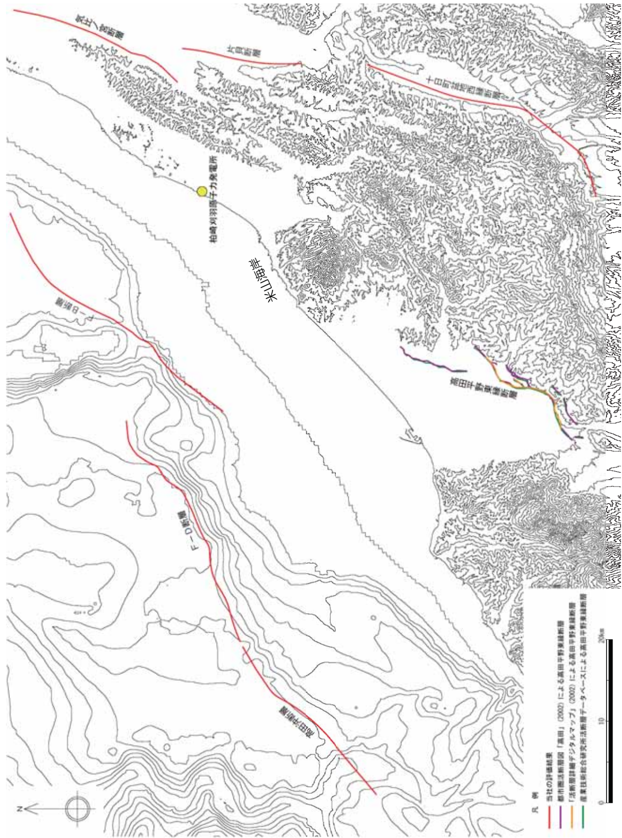
参図-3.2.3 米山海岸周辺の主な活断層
