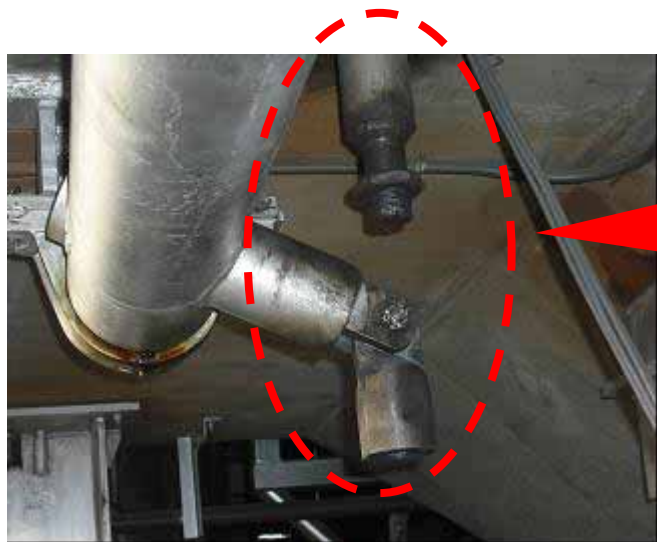
弁駆動部の外れた連結部
