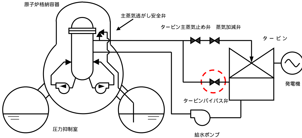
系統概略図
