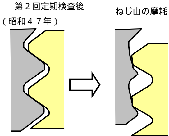
ゆるみ防止用ナットの締め付け不足による差込側のねじ山の摩耗
