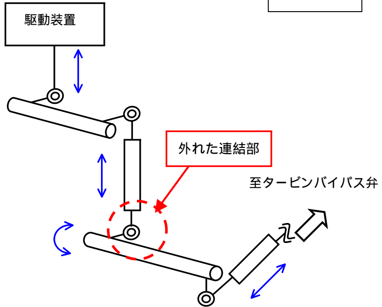
タービンバイパス弁駆動部の連結部
