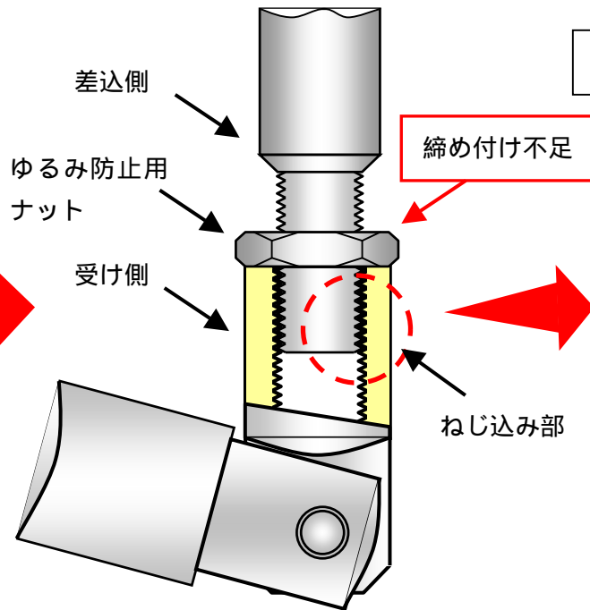
接続状態の連結部
