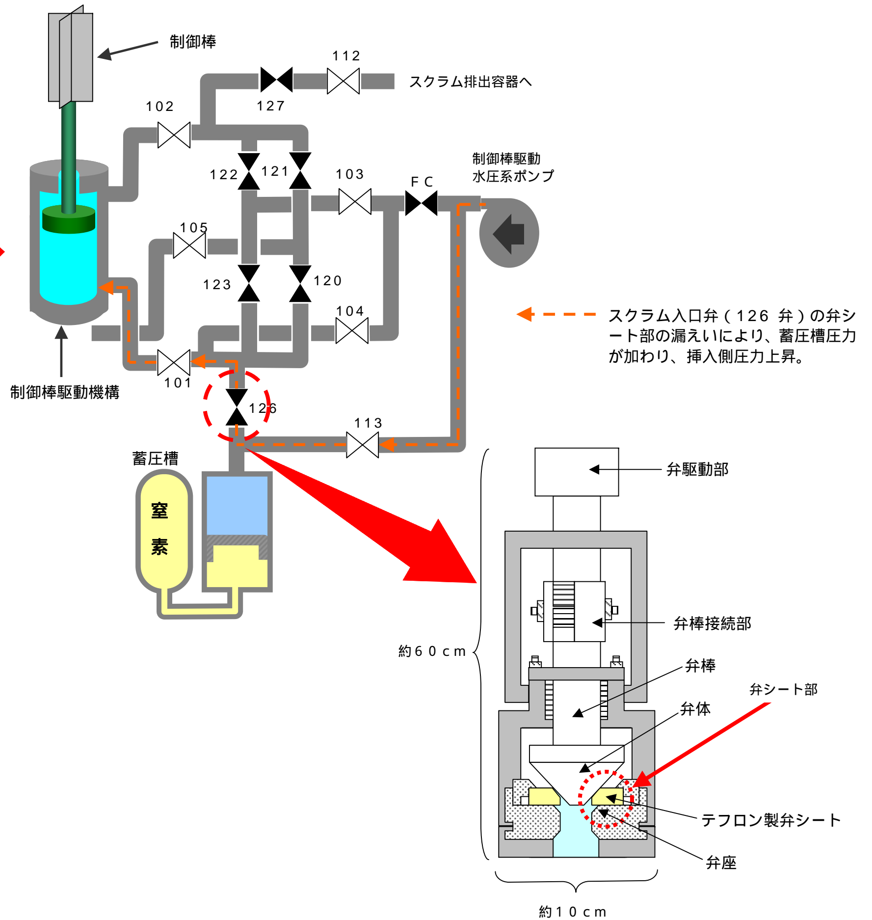
制御棒駆動水圧系およびスクラム入口弁の概略図
