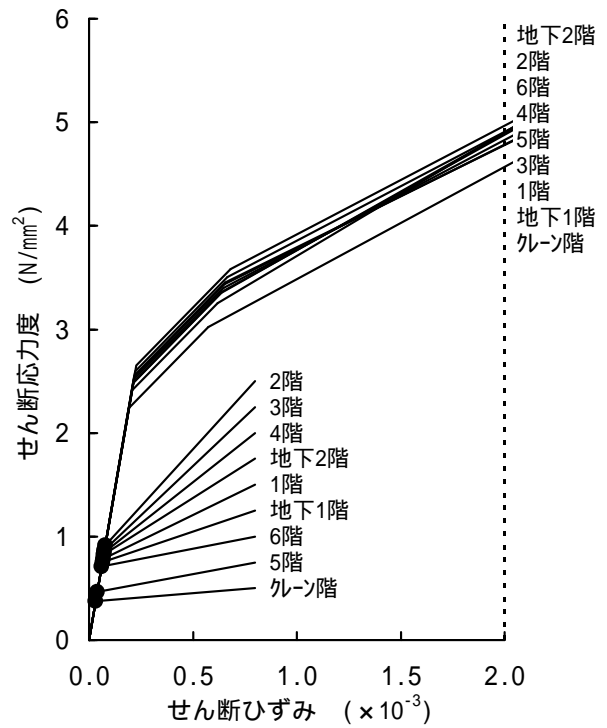
図 3-9 4号機 耐震壁のせん断ひずみ (Sd-1H 東西方向)
