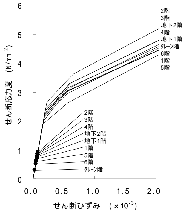
図 3-7 3号機 耐震壁のせん断ひずみ (Sd-1H 東西方向)
