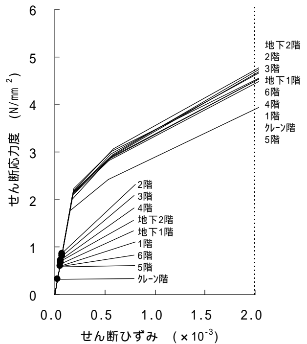
図 3-5 2号機 耐震壁のせん断ひずみ (Sd-1H 東西方向)
