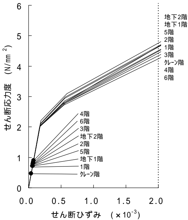
図 3-4 2号機 耐震壁のせん断ひずみ (Sd-2H 南北方向)
