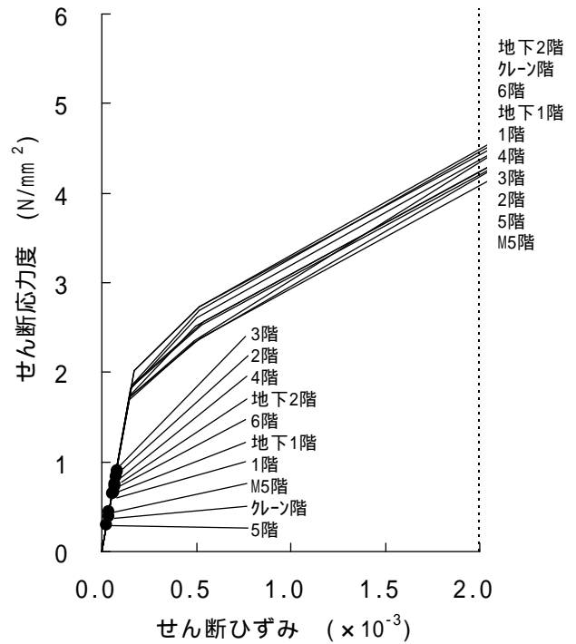
図 3-3 1号機 耐震壁のせん断ひずみ (Sd-2H 東西方向)
