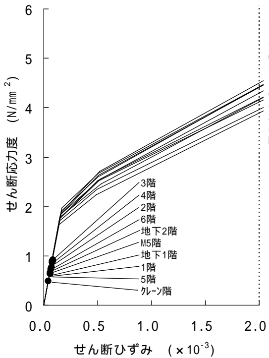
図 3-2 1号機 耐震壁のせん断ひずみ (Sd-2H 南北方向)
