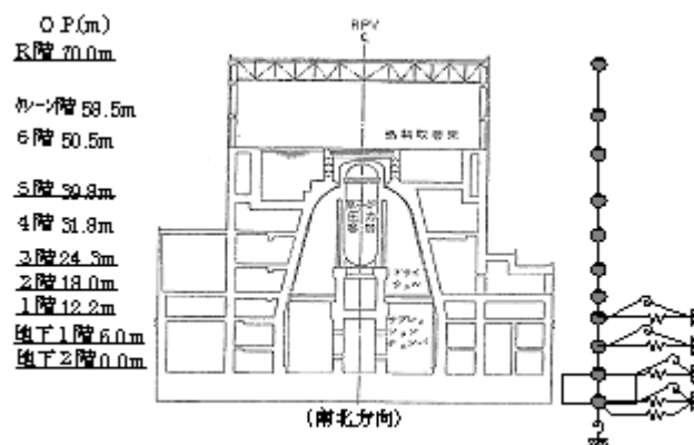
図 3-1 原子炉建屋 (モデル図：3号機例示)
