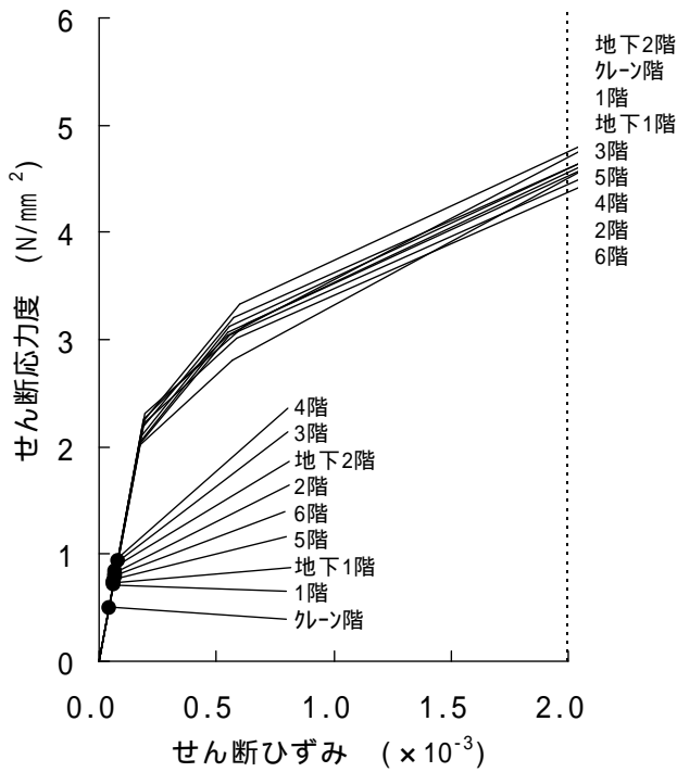
図 3-6 3号機 耐震壁のせん断ひずみ (Sd-2H 南北方向)
