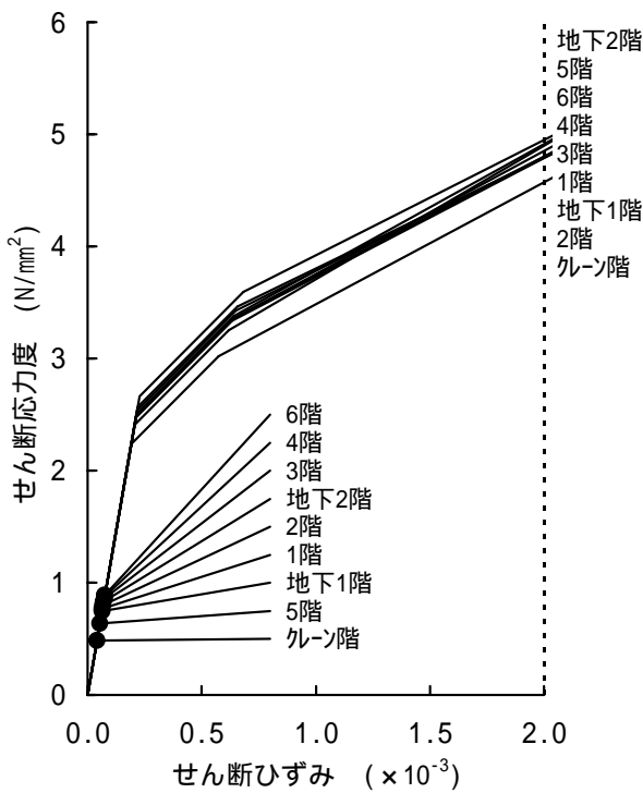
図 3-8 4号機 耐震壁のせん断ひずみ (Sd-2H 南北方向)
