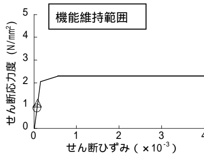
参図-12.5 せん断スケルトン曲線上の最大応答値(東西方向)
