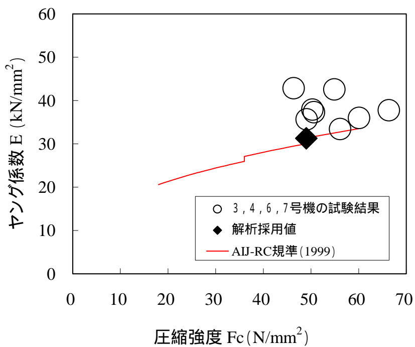
参図-1.3 ヤング係数の分布図 (K3、K4、K6、K7)
