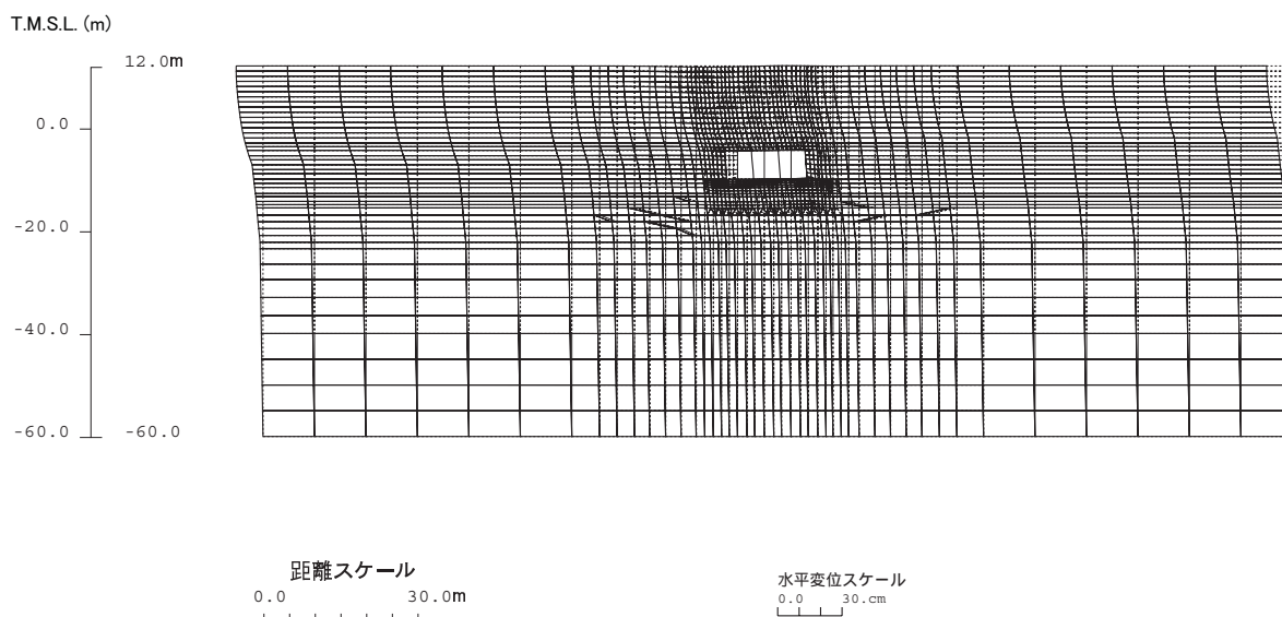
参図-15.8 取水路変形図 (8.21 秒)
