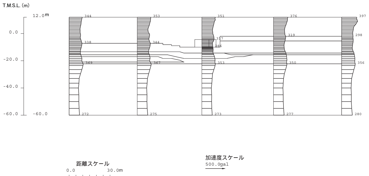
参図-15.4 取水路最大加速度分布図
