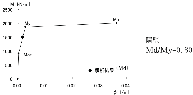
参図-15. 16 取水路 M-\phi スケルトン
