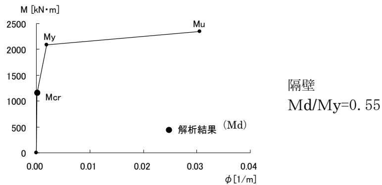
参図-15. 15 スクリーン室 M-\phi スケルトン
