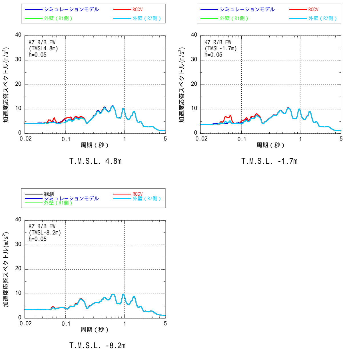
参図-6.4(a) K7-R/B 加速度応答スペクトル (EW 方向)
