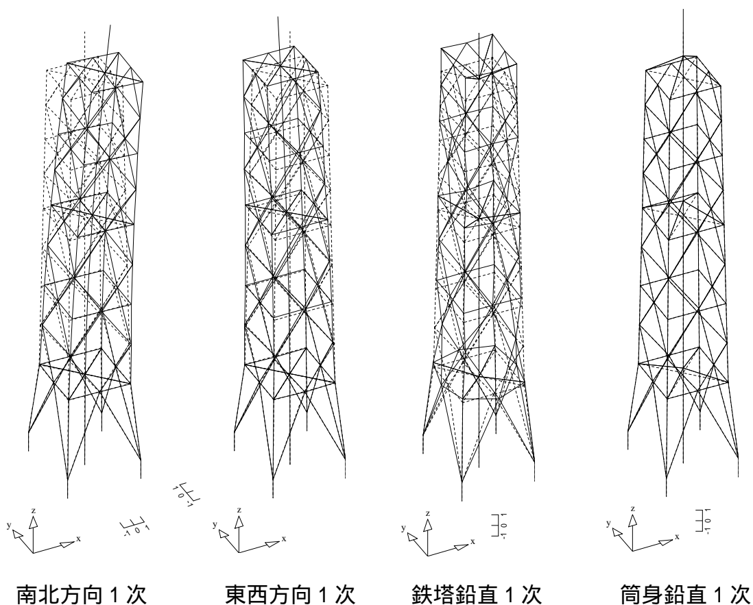
図-5.3.4 固有値解析結果（刺激関数）
