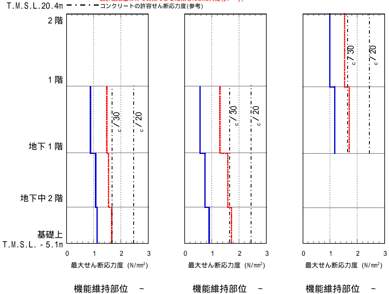
図-5.2.18 機能維持部位のせん断応力度 (東西方向)
