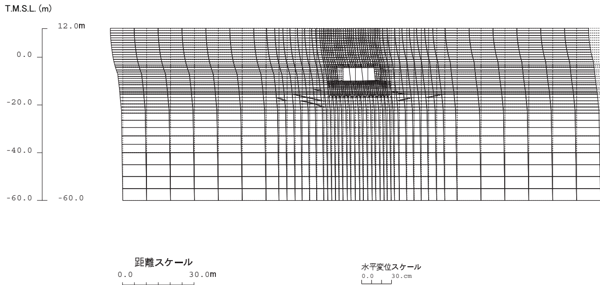
図-5.4.20 取水路変形図 (8.21 秒)
