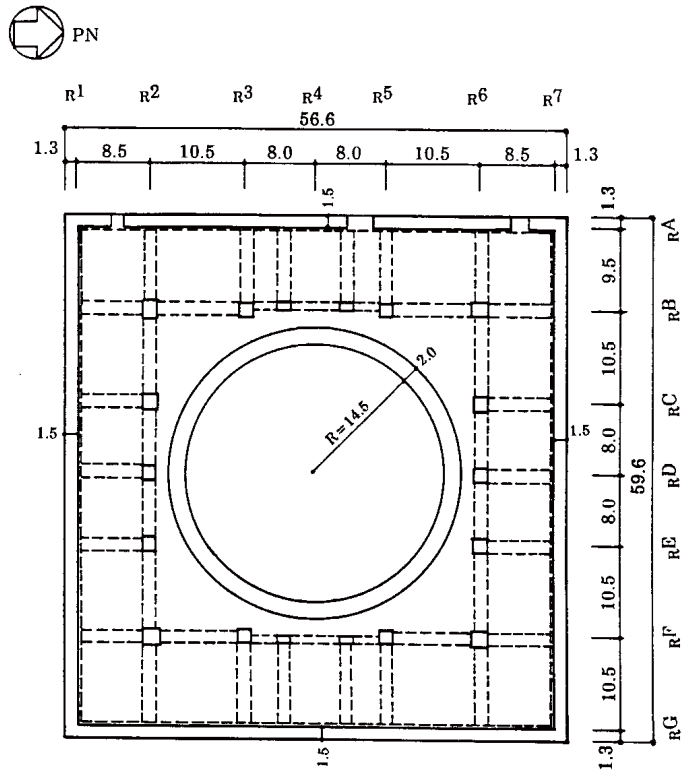
图-3.3.4 地下1階 (T.M.S.L. 4.8m)
