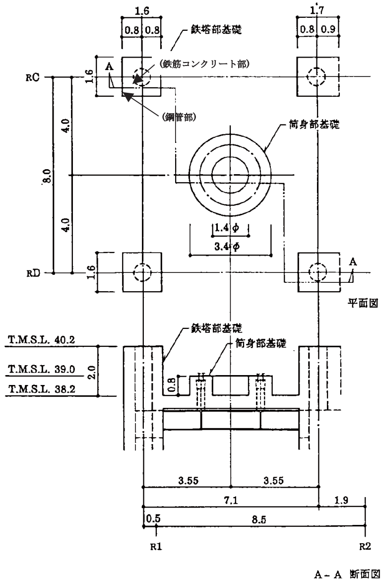
図-5.3.10 排気筒の基礎の概要図
