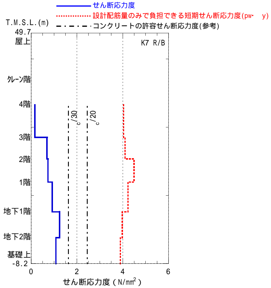
図-5.1.20 RCCVの鉄筋コンクリート部のせん断応力度 (南北方向) c = コンクリートの実強度
