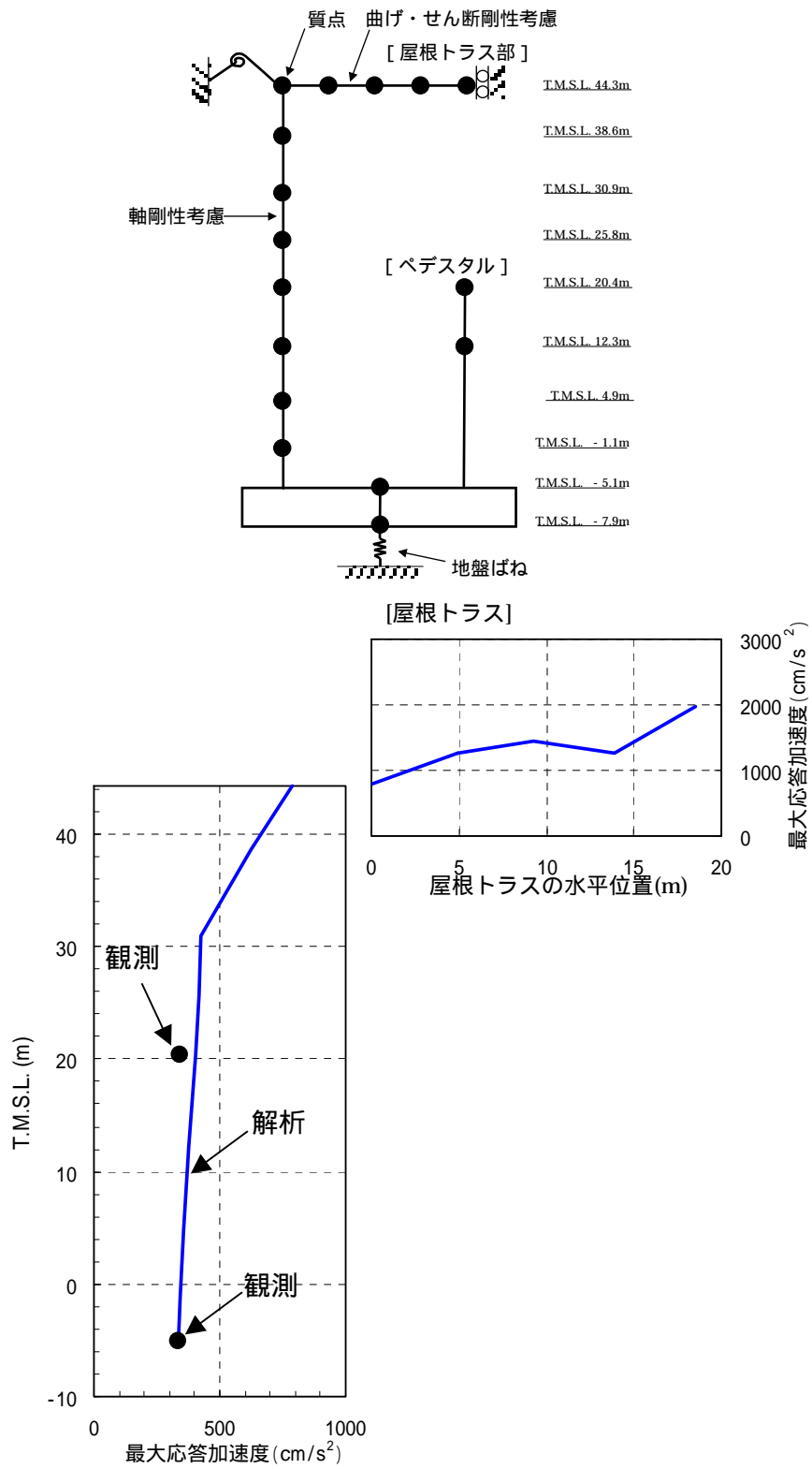
図-5.2.13 最大応答加速度 (鉛直方向)
