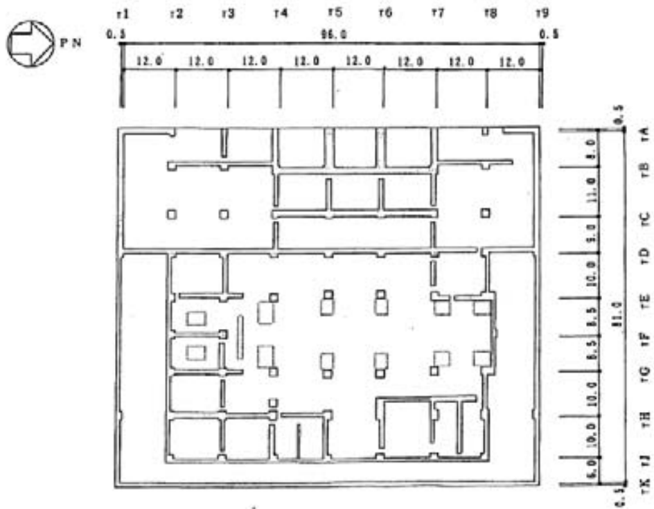
図-3.3.11 地下2階 (T.M.S.L. 5.1m)
