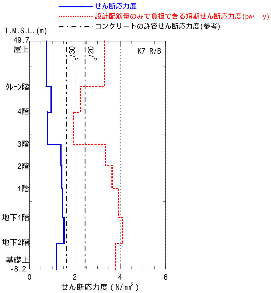
図-5.1.16 原子炉建屋 耐震壁のせん断応力度 (南北方向)
