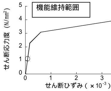
図-5.2.22 せん断スケルトン曲線上の最大応答値（東西方向）
