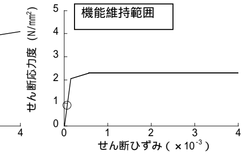
図-5.2.22 せん断スケルトン曲線上の最大応答値（東西方向）
