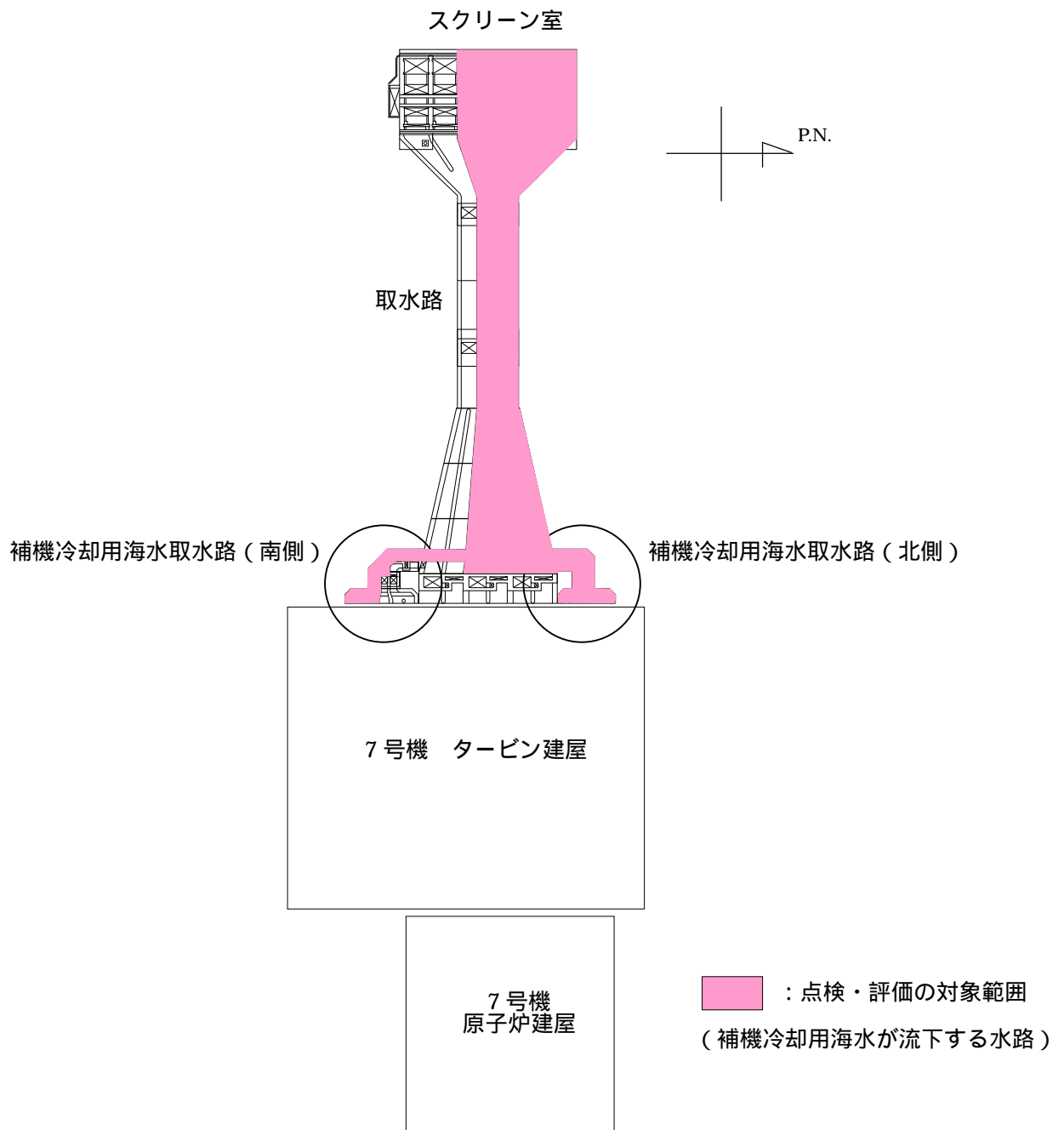
図-3.3.21 屋外重要土木構造物の配置図
