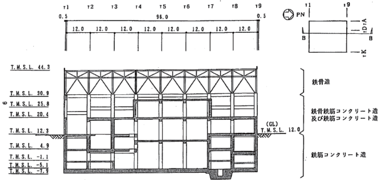
図-3.3.16 NS方向断面図
