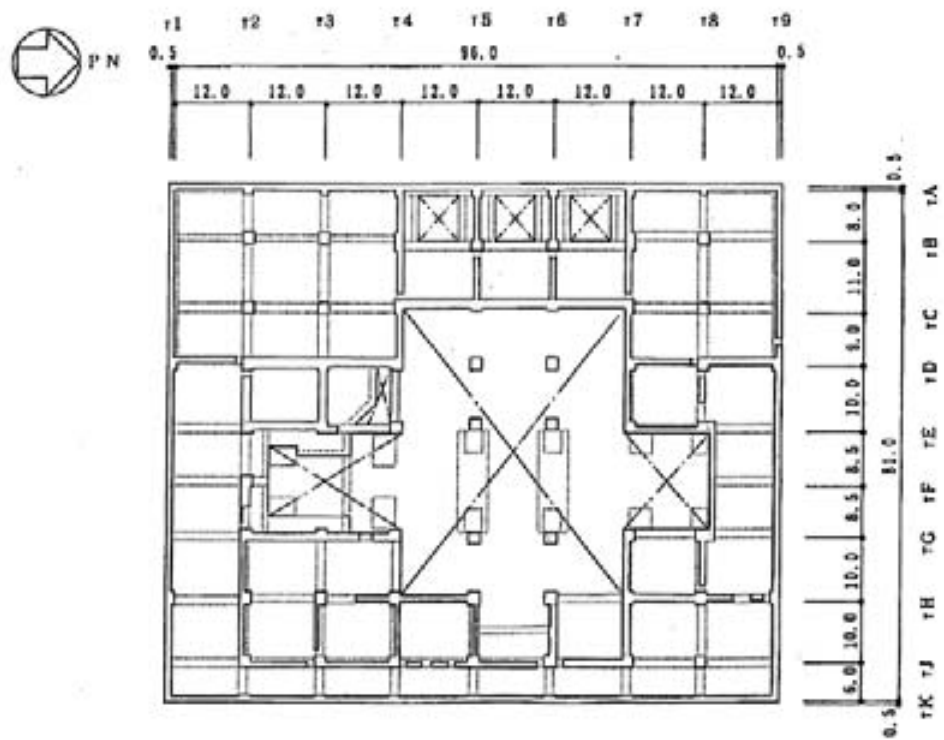
図-3.3.12 地下1階 (T.M.S.L. 4.9m)
