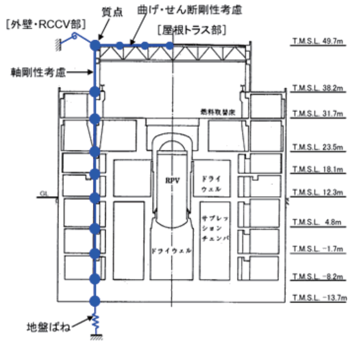
図-5.1.11 地震応答解析モデル（鉛直方向）
