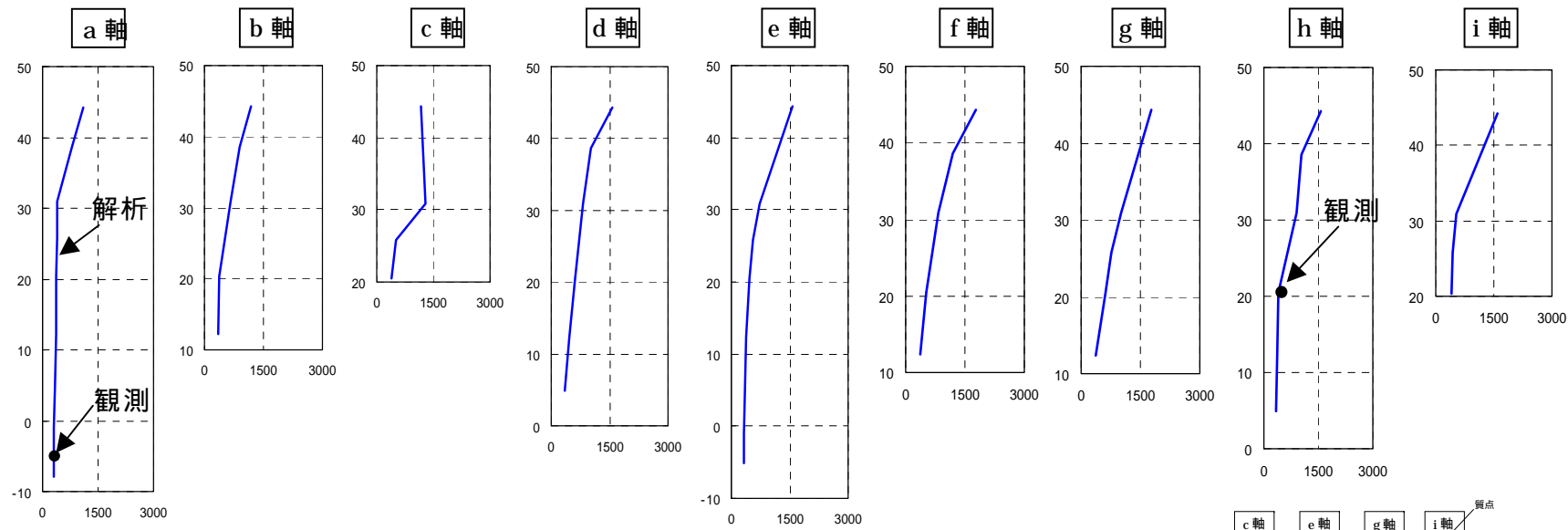
縦軸：T.M.S.L.(m)、横軸：最大応答加速度 (cm/s 2 )
