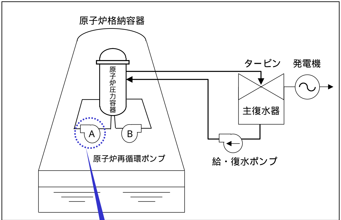
系統概略図
