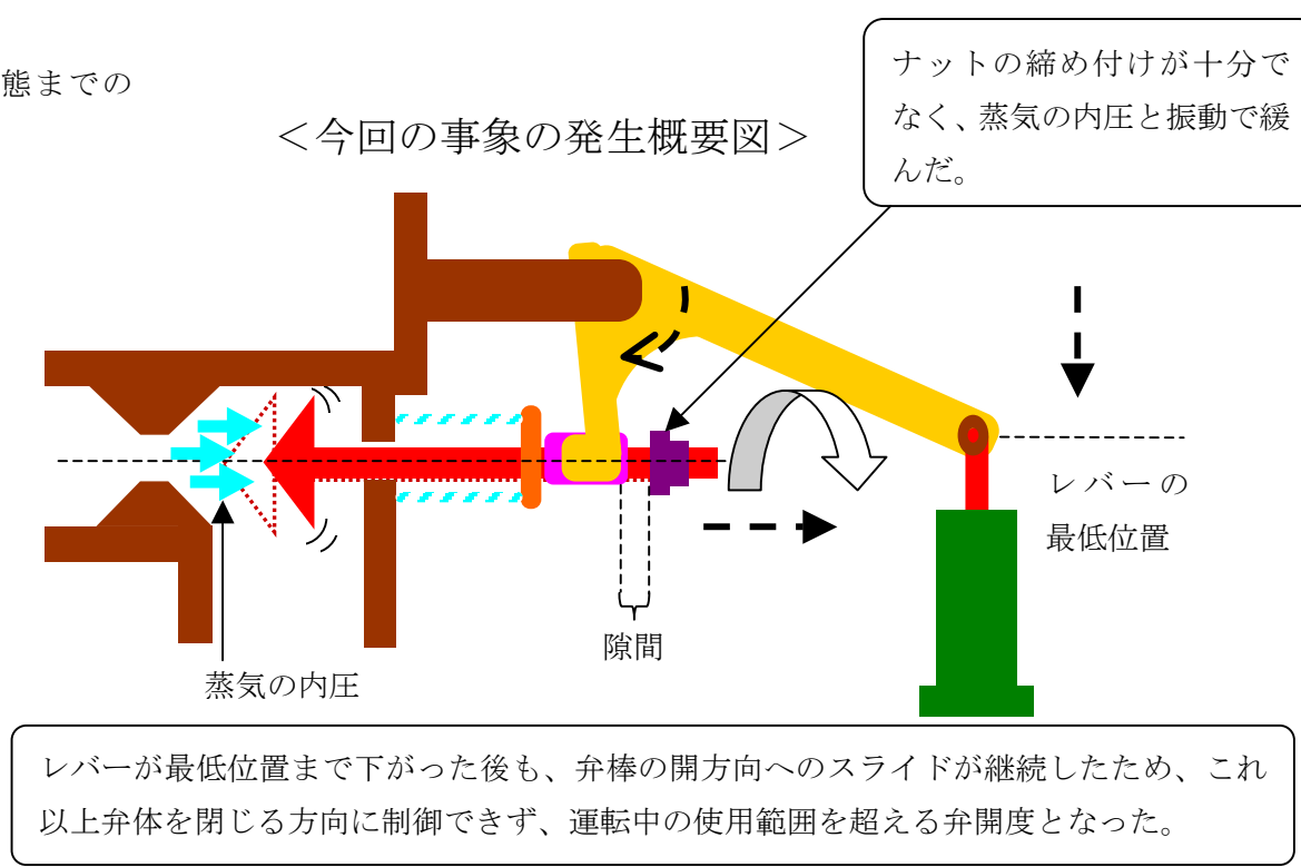
原子炉隔離時冷却系の蒸気加減弁の構造図および事象発生概要図
