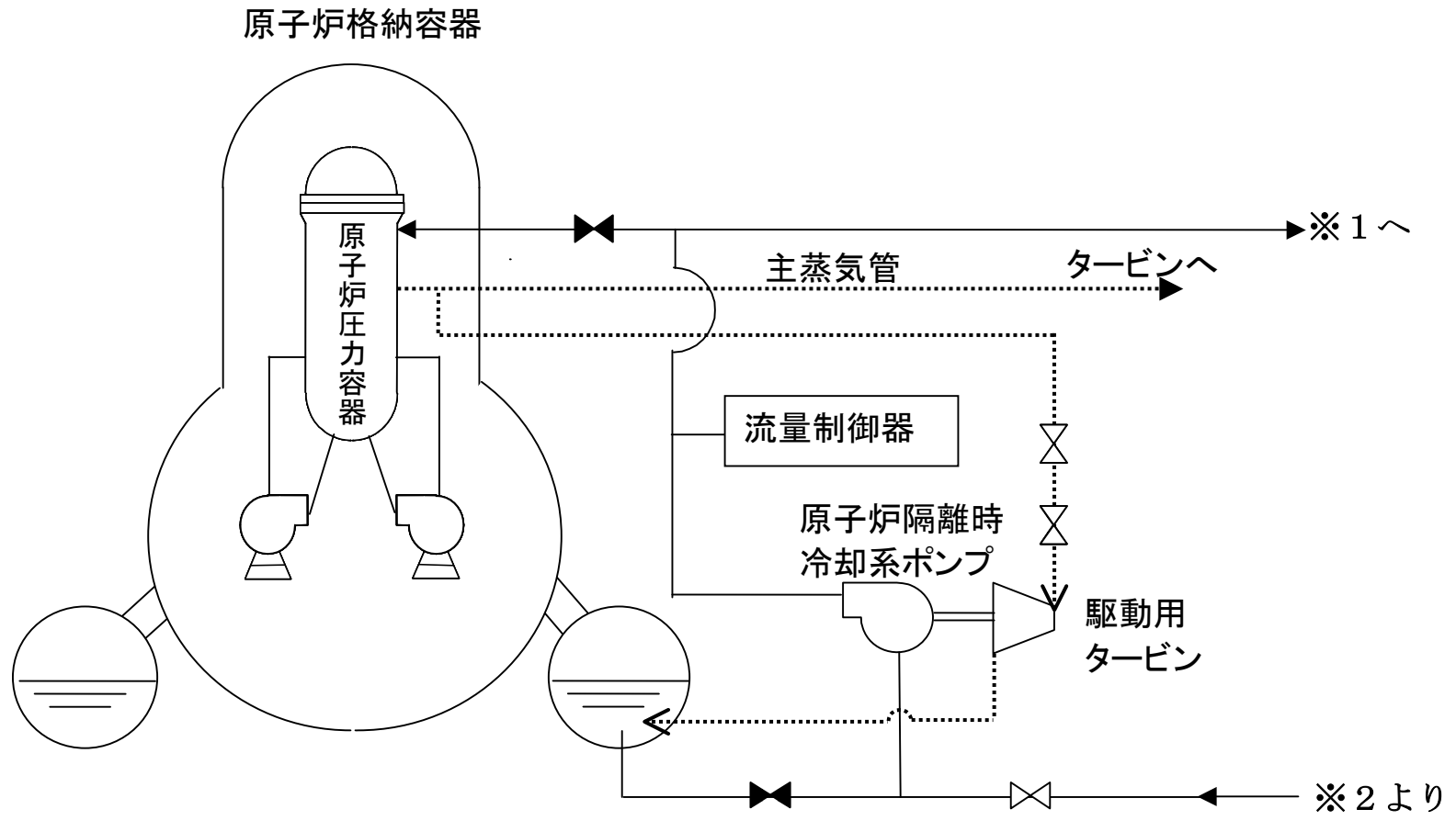
原子炉隔離時冷却系系統概略図（手動起動試験時）
