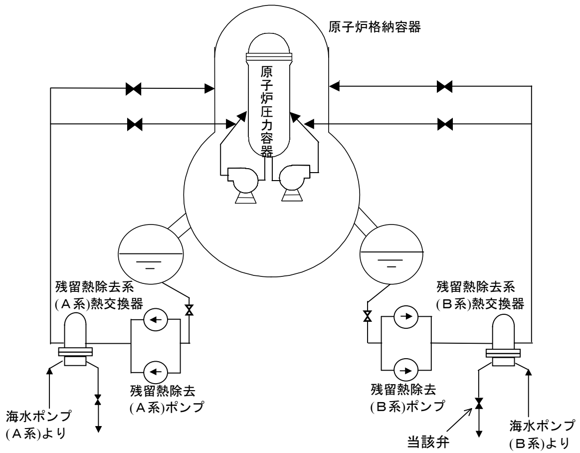
2号機残留熱除去系 系統概略図
