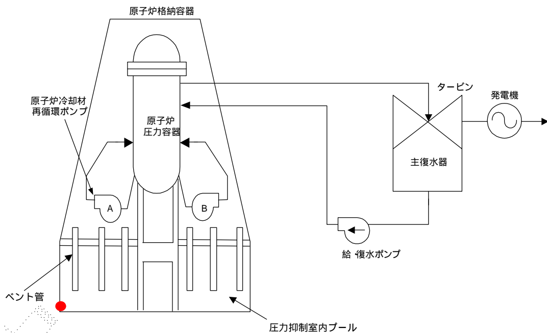
系統概略図
