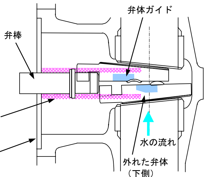
下側の弁体が外れて当該弁が閉じない状態
