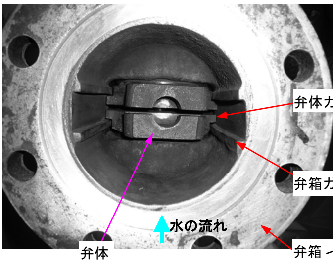
弁箱内部写真
