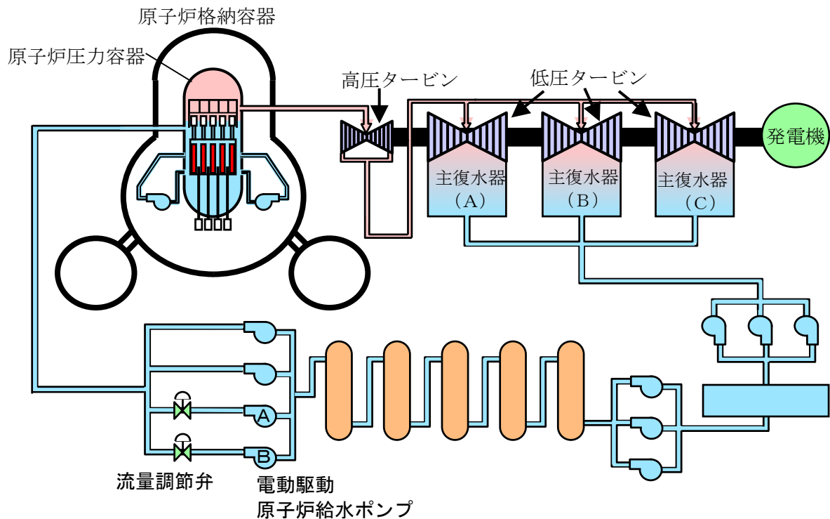
福島第一原子力発電所 4号機 系統概略図
