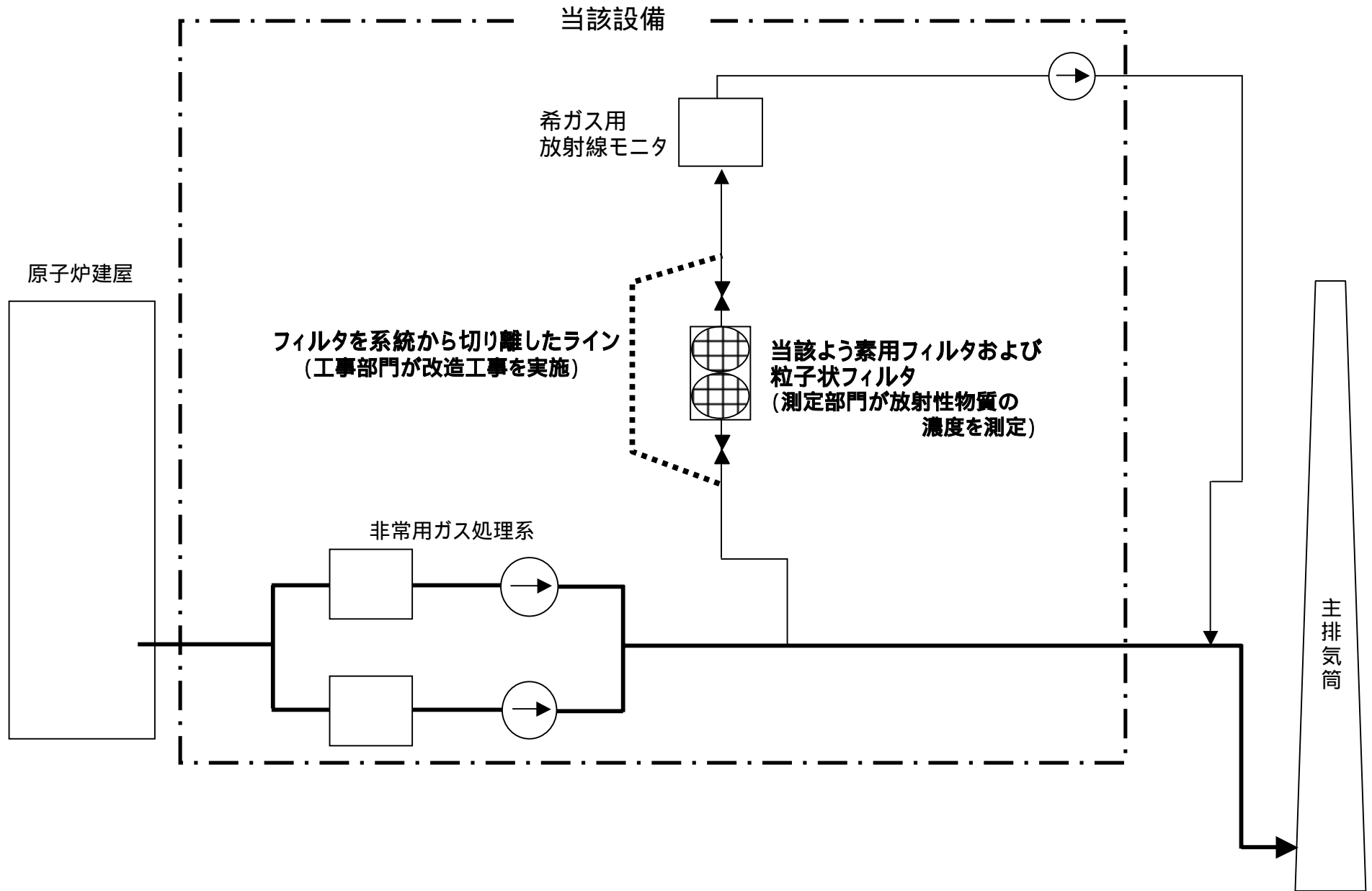
4号機 非常用ガス処理系 系統概略図
