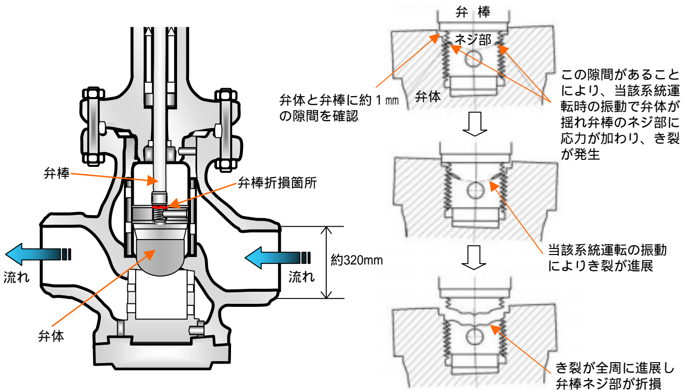
残留熱除去系 流量調節弁概略構造図および弁棒折損のメカニズム
