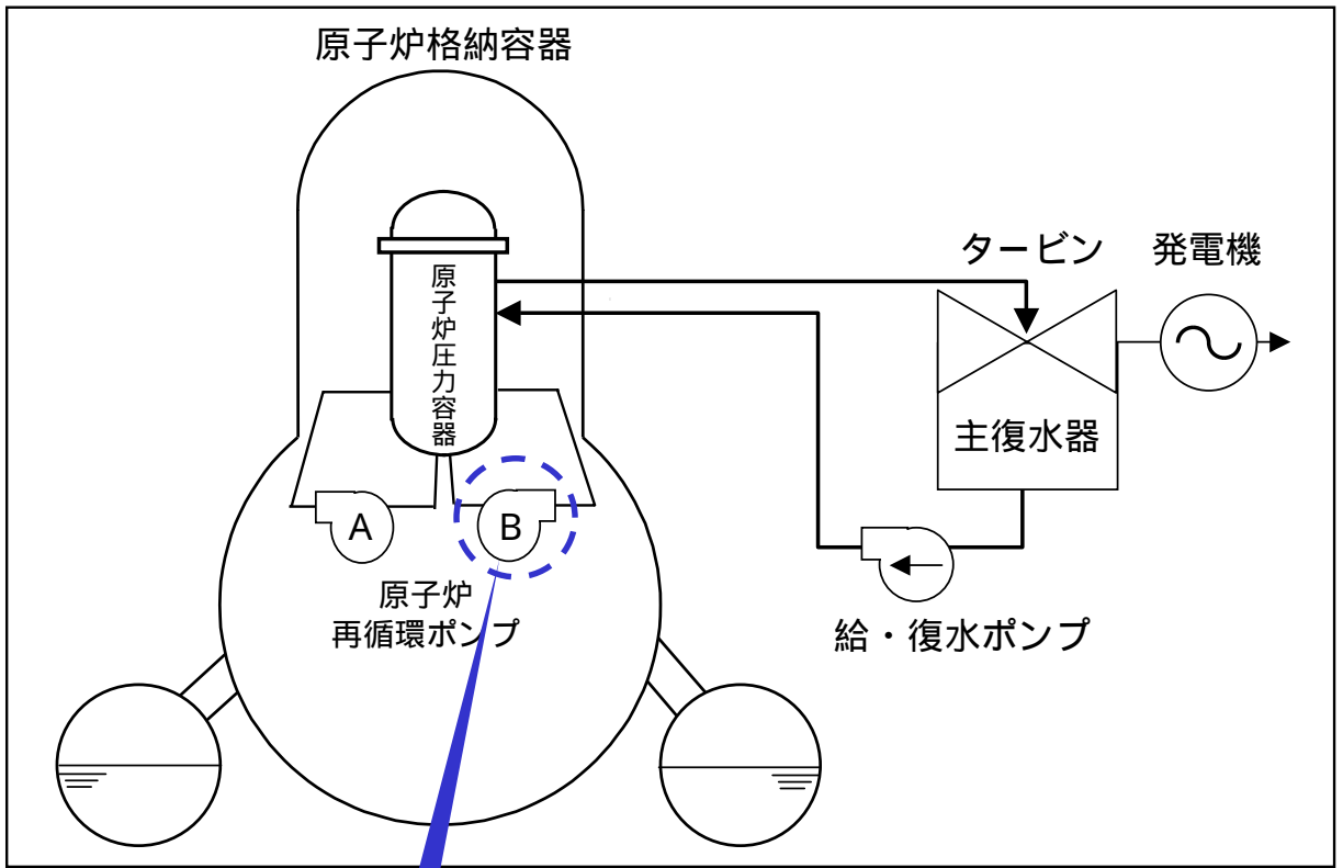
系統概略図
