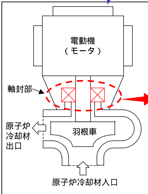
原子炉再循環ポンプ概略図
