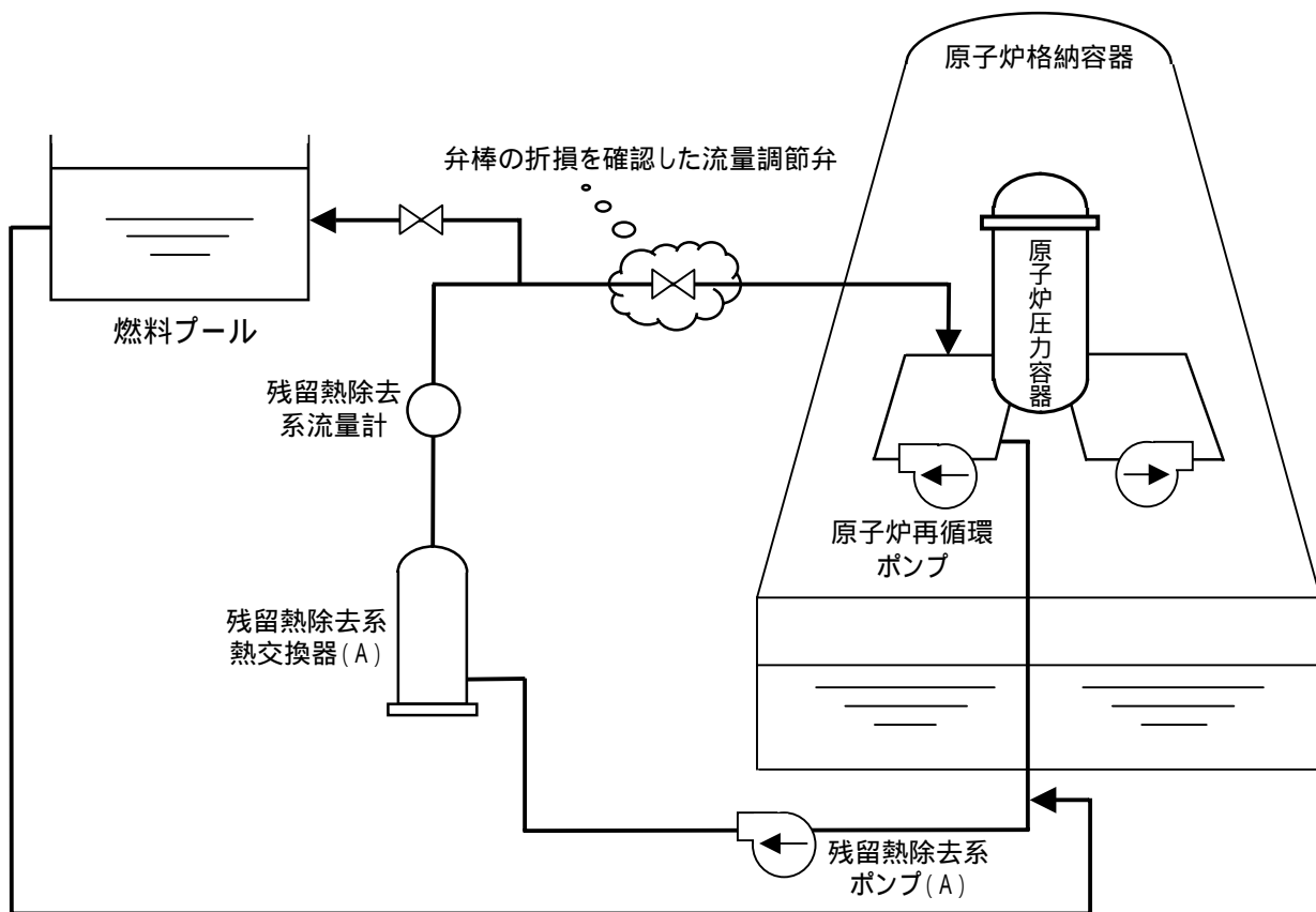
残留熱除去系 系統概略図
